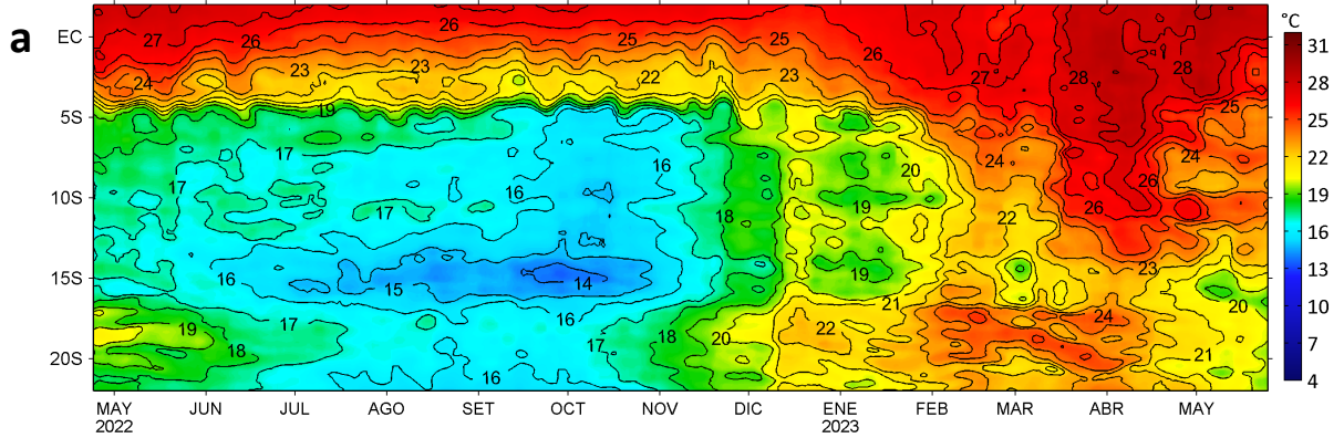
Anomalías de la Temperatura Superficial del mar (°C), franja costera de 60 m.n. 24 de abril 2022 - 25 de mayo 2023
