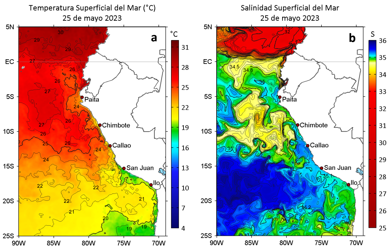
Figura 2. a) Temperatura superficial del mar ( ^{\circ}\text{C} ) y b) Salinidad superficial del mar para el 25 de mayo de 2023. Datos: OSTIA-UKMO-L4-GLOB-v2.0 (UK Met Office, 2012; Donlon et al, 2012) y del GLOBAL_ANALYSISFORECAST_PHY_001_024 (Lellouche, J. M. et al, 2013), respectivamente.
