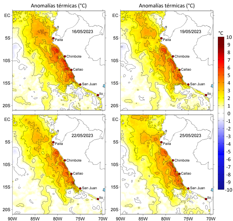
Figura 3. Anomalías de la temperatura superficial del mar ( ^{\circ}\text{C} ) para el a) 16, b) 19, c) 22 y d) 25 de mayo de 2023. Las anomalías se calcularon respecto de la climatología para el periodo 2007-2016. Datos: OSTIA-UKMO-L4-GLOB-v2.0 (UK Met Office, 2012; Donlon et al, 2012).
