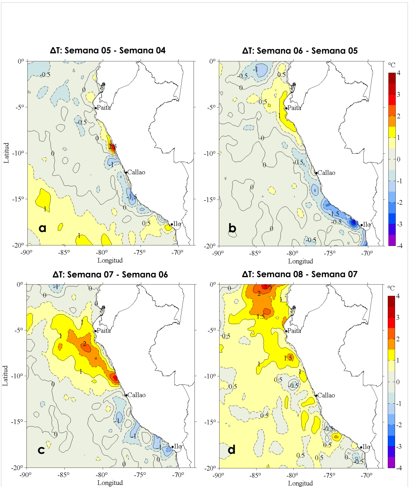
Figura 3. Variación semanal de la anomalía de la temperatura superficial del mar promedio (°C) en el océano Pacífico tropical oriental entre: a) la quinta (29 de enero - 04 de febrero) y cuarta (22 - 28 de enero) semana, b) la sexta (05 - 11 de febrero) y quinta (29 de enero - 04 de febrero) semana, c) la séptima (12 - 18 de febrero) y sexta (05 - 11 de febrero) semana, y d) la octava (19 - 25 de febrero) y séptima (12 - 18 de febrero) semana del presente año. Los mapas, que indican el grado de calentamiento o enfriamiento de una semana a otra, provienen del sensor AVHRR v2 del Centro Nacional de Datos Climáticos de la Administración Nacional del Océano y la Atmósfera (NCD/NOAA, según sus siglas en inglés). Las anomalías térmicas se calcularon de acuerdo con la climatología para el período 1982-2011. La barra de colores de las anomalías térmicas se presenta a la derecha. Procesamiento: LHF/AFIOF/DGIOCC/IMARPE.
