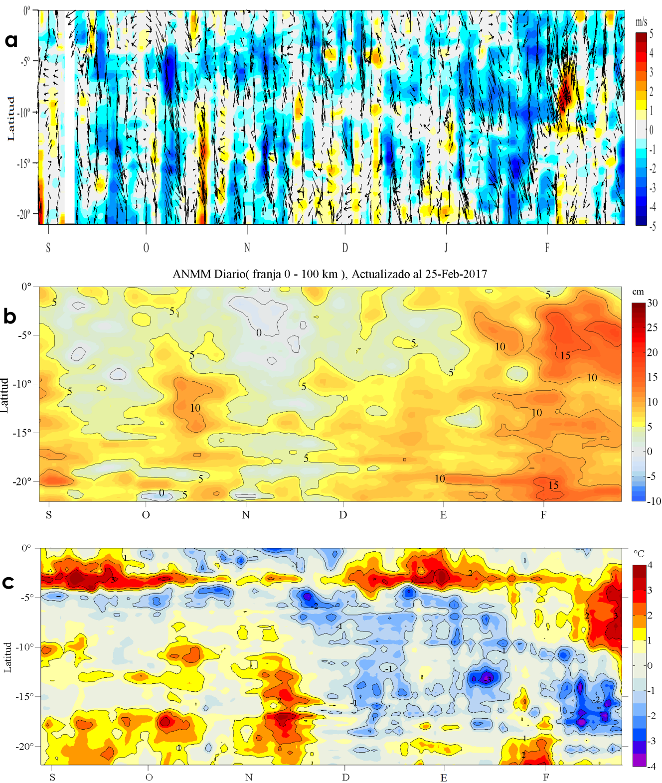
Figura 4. Evolución de las anomalías diarias de: a) velocidad del viento (m/s), b) nivel medio del mar (cm), c) temperatura superficial del mar (°C) para el último semestre actualizado al 25 de febrero de 2017. Datos: de IFREMER/CERSAT para (a), del Servicio de Monitoreo del Ambiente Marino Copernicus (CMEMS, según sus siglas en inglés) para (b) del satélite AVHRR v2 del Centro Nacional de Datos Climáticos de la Administración Nacional del Océano y la Atmósfera (NCDC/NOAA, según sus siglas en inglés) para (c). Las anomalías fueron calculadas para una franja de 100 km adyacente a la costa entre el ecuador y 21°S según los promedios climatológicos diarios de 2000-2014 para (a), de 1993-2013 para (b) y de 1982-2011 para (c). La barra de colores a la derecha muestra la escala de las anomalías en cada caso. Procesamiento: LHF/AFIOF/DGIOCC/IMARPE.
