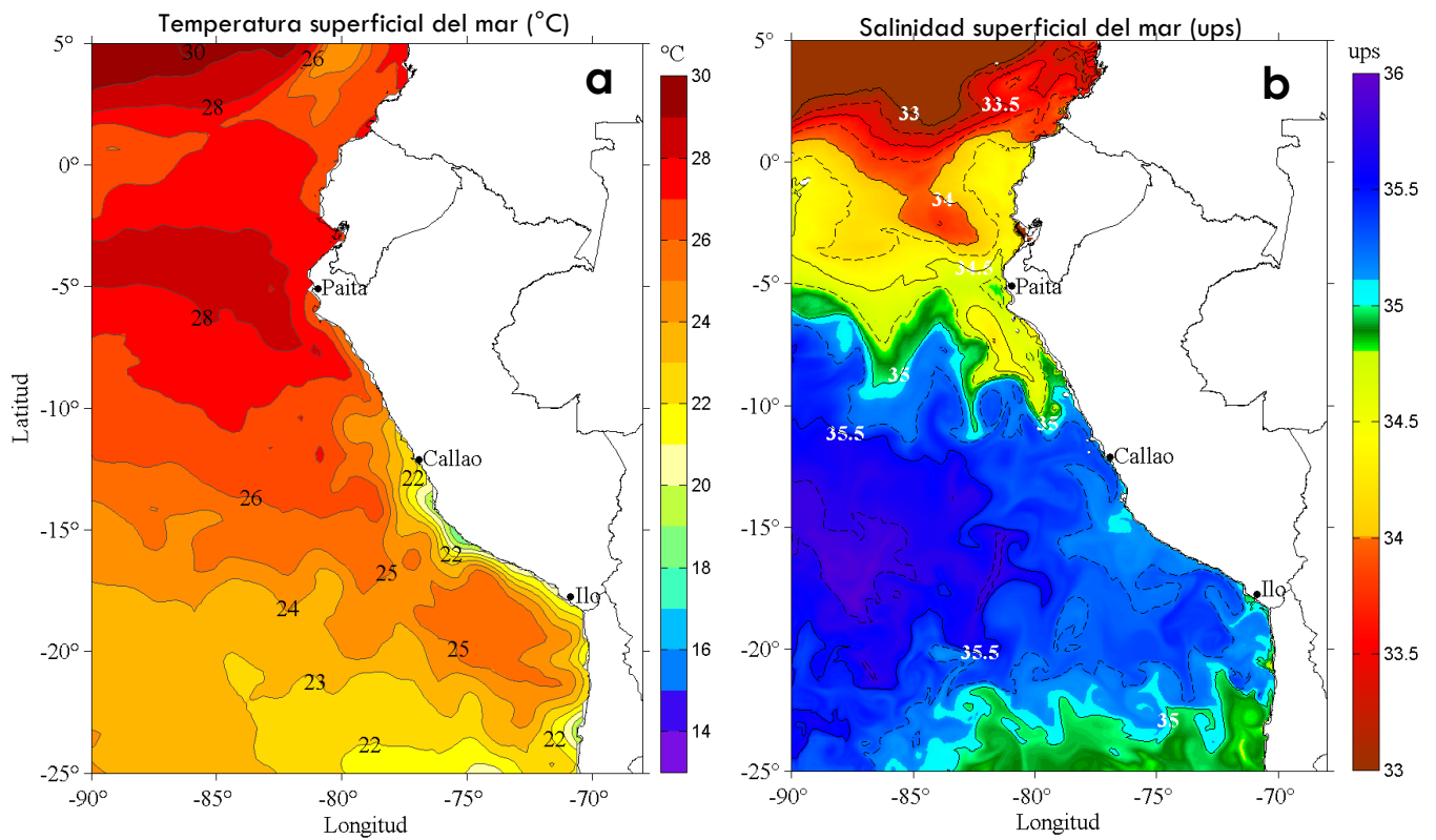
Figura 1. Distribución espacial promedio de: a) Temperatura Superficial del Mar ( ^{\circ}\text{C} ) y b) Salinidad Superficial del Mar, para la semana del 19 al 25 de febrero de 2017 en el océano Pacífico tropical oriental. Datos: AVHRR v2 del Centro Nacional de Datos Climáticos de la Administración Nacional del Océano y la Atmósfera (NCDC/NOAA, según sus siglas en inglés) para (a) y del Hybrid Coordinate Ocean Model (HYCOM; Halliwell et al., 1998; 2000; Bleck, 2001) para (b). Las escalas de colores de la temperatura como de la salinidad superficial del mar se presentan a la derecha de cada gráfico. Procesamiento: LHFM/AFIOF/DGIOCC/IMARPE.
