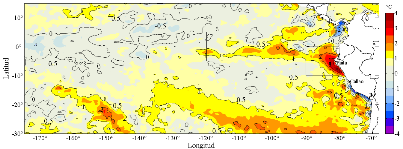
Figura 2. Anomalías promedio de la temperatura superficial del mar ( ^{\circ}\text{C} ) en el océano Pacífico tropical para la semana del 18 al 25 de febrero de 2017. Las regiones Niño 3.4 y Niño 1+2 en los sectores central y oriental del océano, respectivamente, están delimitadas con una línea de color gris. Datos: AVHRR Global Reyn_SmithOlv2R (Reynolds, et. al., 2007) de CMB/EMC/NCEP de la Administración Nacional del Océano y la Atmósfera (NOAA, según sus siglas en inglés). Las anomalías se calcularon con respecto de la climatología para el período 1982-2011. Procesamiento: IMARPE.
