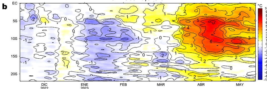
Figura 5. Evolución de las anomalías diarias de: a) Velocidad del viento (m/s) y b) Temperatura superficial del mar (°C) para el último semestre, actualizado al 13 de mayo de 2023. Datos: de IFREMER/CERSAT para (a) y de OSTIA-UKMO-L4-GLOB-v2.0 para (b). Las anomalías fueron calculadas para una franja de 60 m.n. adyacente a la costa entre el ecuador geográfico y 22°S según los promedios climatológicos diarios de 2000-2014 para (a) y de 2007-2016 para (b). La barra de colores a la derecha muestra la escala de las anomalías en cada caso.
