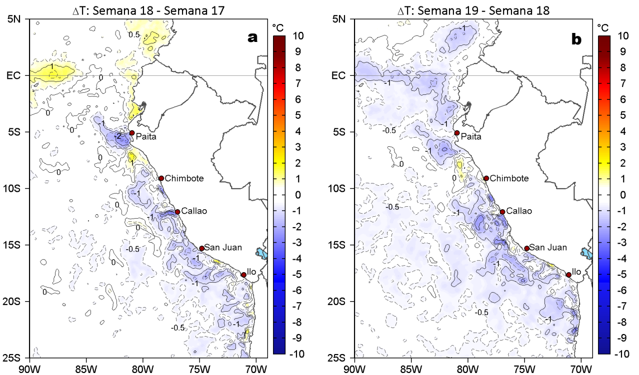
Figura 3. Variación semanal de la TSM (°C) en el océano Pacífico tropical oriental entre: a) décimo octava (30 de abril - 06 de mayo) y décimo séptima (23-29 de abril) semana de 2023 y b) décimo novena (07-13 de mayo) y décimo octava (30 de abril - 06 de mayo) semana de 2023. Los mapas, que indican el grado de calentamiento o enfriamiento de una semana a otra, provienen de OSTIA-UKMO-L4-GLOB-v2.0 (UK Met Office, 2012; Donlon et al, 2012). La barra de colores a la derecha muestra la diferencia de la temperatura entre la presente y la semana previa.
