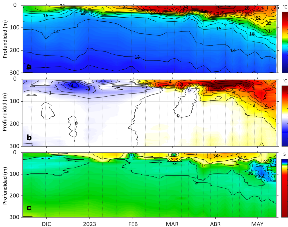
Figura 7. Diagrama Hovmöller de: a) Temperatura del mar (°C), b) Anomalías térmicas (°C) y c) Salinidad del mar, perfilador ARGO No. 6903002 localizado a 72 m.n. (5,92°S, 82,20°W) frente a Punta Falsa el 14 de mayo de 2023. Las anomalías de la temperatura del agua se calcularon de acuerdo a Domínguez et al (2017). Los puntos en la columna de agua indican los días en que el perfilador registró información. Datos: ARGO.
