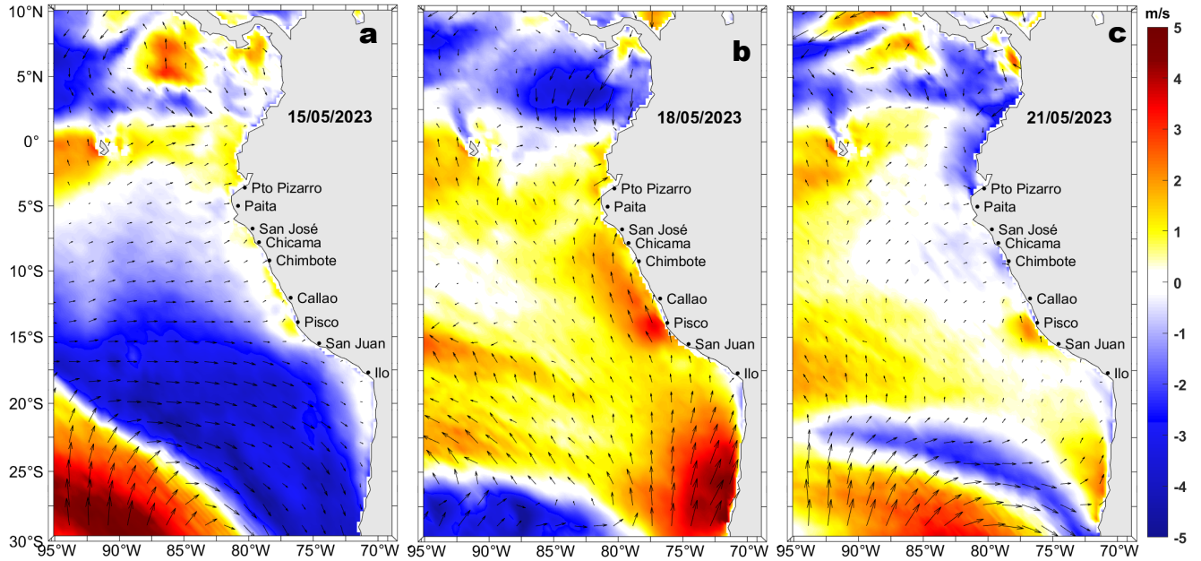
Figura 10. Distribución espacial del pronóstico de las anomalías de la Velocidad del Viento (VV, m/s) y dirección del viento (°) para el a) 15, b) 18 y c) 21 de mayo de 2023, frente a la costa entre Panamá y Chile. Fuente: Modelo Climate Forecast System (GFS) de la NOAA.
