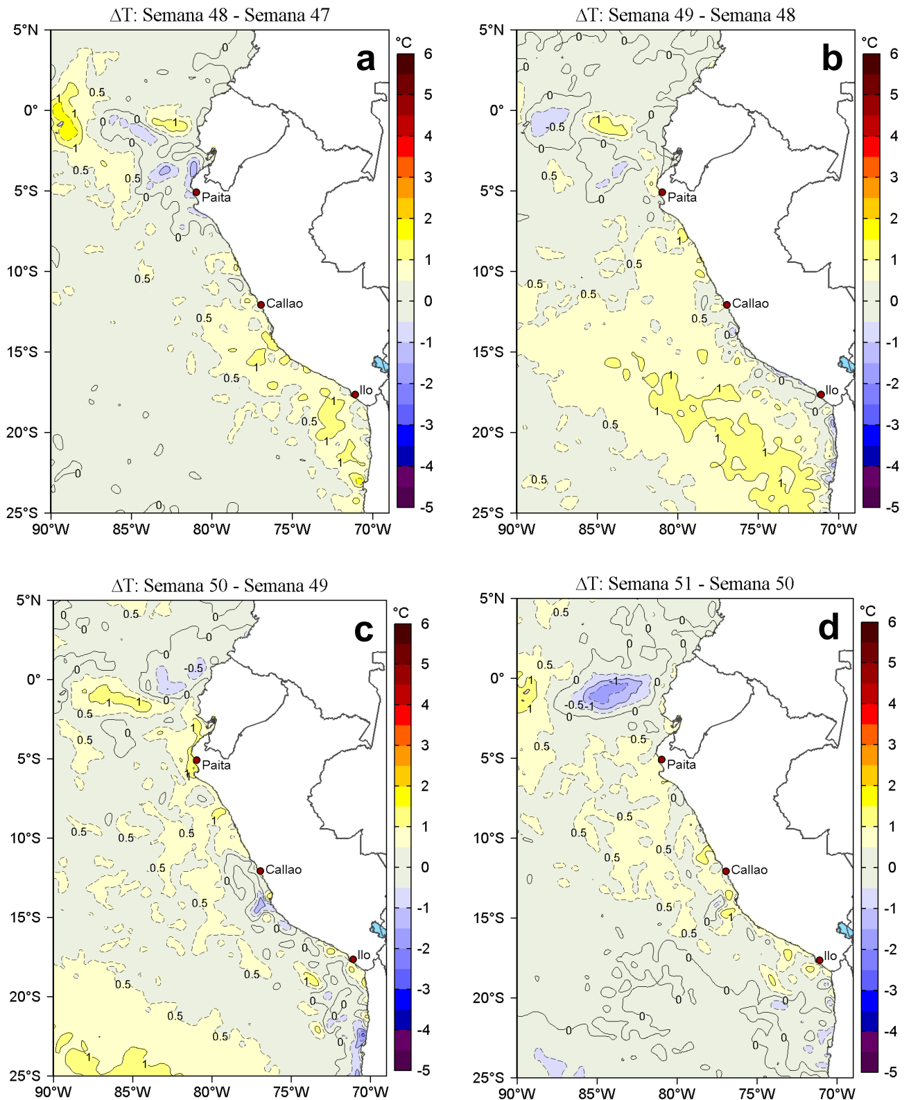
Figura 3. Variación semanal de la Temperatura Superficial del Mar (°C) en el océano Pacífico tropical oriental entre: a) cuadragésimo octava (26 de noviembre - 02 de diciembre) y cuadragésimo séptima (19-25 de noviembre) semana del 2018, b) cuadragésimo novena (03-09 de diciembre) y cuadragésimo octava (26 de noviembre - 02 de diciembre) semana del 2018, c) quincuagésima (10-16 de diciembre) y cuadragésimo novena (03-09 de diciembre) semana del 2018 y d) quincuagésima primera (17-23 de diciembre) y quincuagésima (10-16 de diciembre) semana del 2018. Los mapas, que indican el grado de calentamiento o enfriamiento de una semana a otra, provienen de OSTIA-UKMO-L4-GLOB-v2.0 (UK Met Office, 2012; Donlon et al, 2012). La barra de colores a la derecha muestra la diferencia de la temperatura entre la presente y la semana previa. Procesamiento: LHF/AFIOF/DGIOCC/IMARPE.
