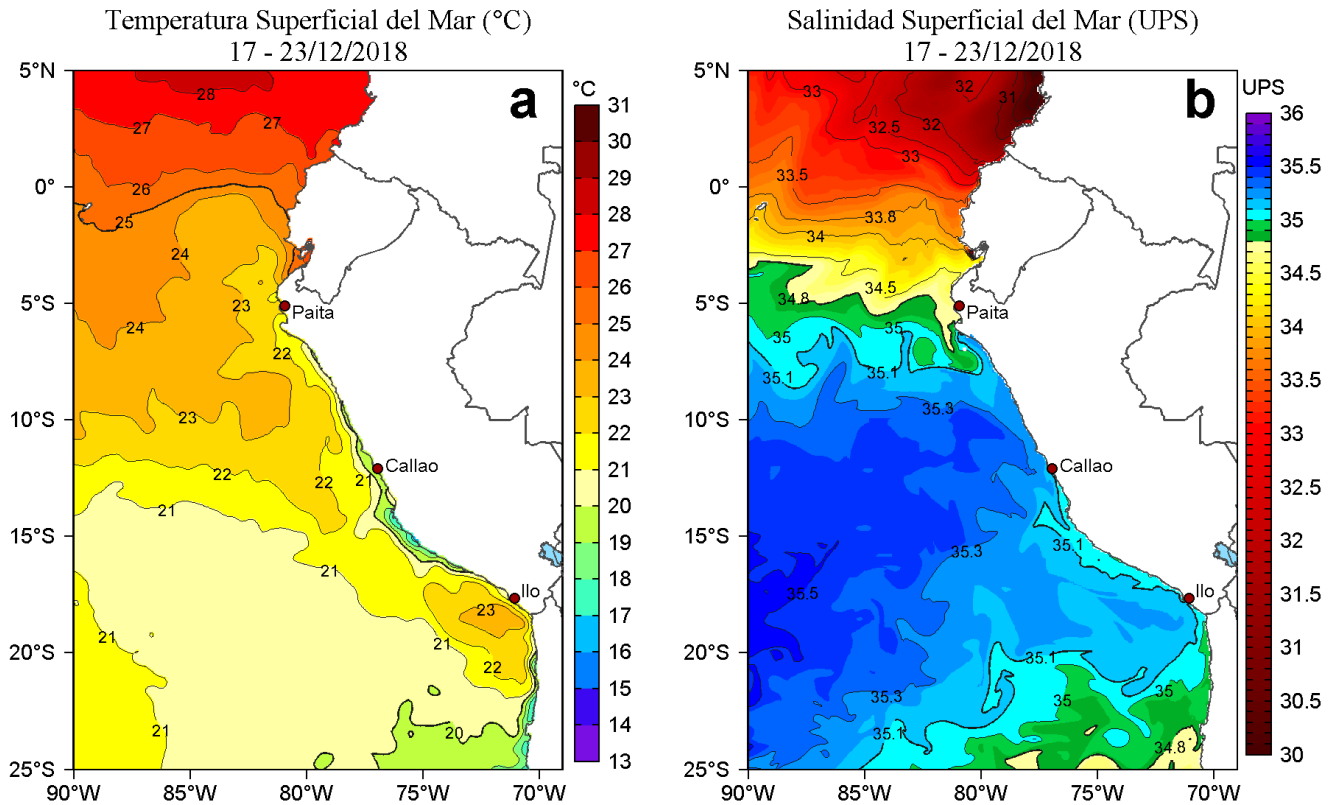
Figura 1. Distribución espacial promedio de: a) Temperatura Superficial del Mar (TSM, °C) y b) Salinidad Superficial del Mar (SSM, UPS) para la semana del 17 al 23 de diciembre de 2018 en el océano Pacífico tropical oriental. Datos: OSTIA-UKMO-L4-GLOB-v2.0 (UK Met Office, 2012; Donlon et al, 2012) disponible en https://podaac.jpl.nasa.gov/dataset/OSTIA-UKMO-L4-GLOB-v2.0 para (a) y del Hybrid Coordinate Ocean Model (HYCOM; Halliwell et al., 1998; 2000; Bleck, 2001) v. GOFS 3.1 para (b). Las escalas de colores de la TSM como de la SSM se presentan a la derecha de cada gráfico. Procesamiento: LHFM/AFIOF/DGIOCC/IMARPE.
