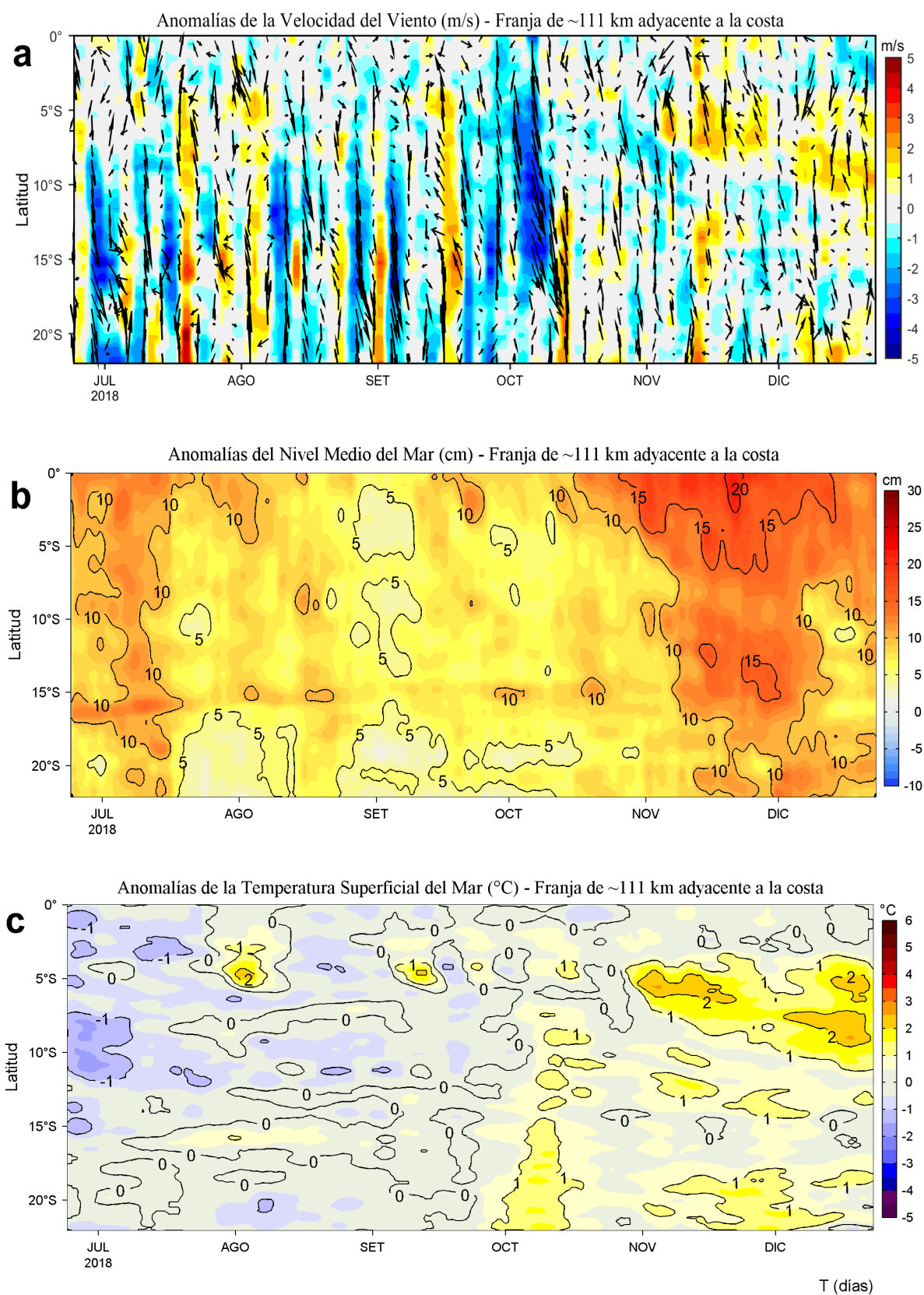
Figura 4. Evolución de las anomalías diarias de: a) Velocidad del viento (m/s), b) Nivel medio del mar (cm), c) Temperatura Superficial del Mar (°C) para el último semestre, actualizado al 23 de diciembre de 2018. Datos: de IFREMER/CERSAT para (a), del Servicio de Monitoreo del Ambiente Marino Copernicus (CMEMS en inglés) para (b), de OSTIA-UKMO-L4-GLOB-v2.0 para (c). Las anomalías fueron calculadas para una franja de 111 km adyacente a la costa entre el ecuador y 22°S según los promedios climatológicos diarios de 2000-2014 para (a), de 1993-2013 para (b) y de 2007-2016 para (c). La barra de colores a la derecha muestra la escala de las anomalías en cada caso. Procesamiento: LHF/AFIOF/DGIOCC/IMARPE.
