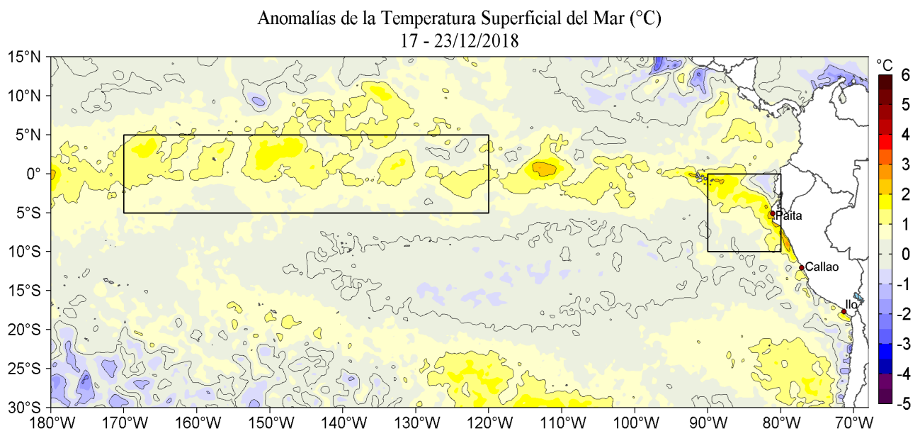
Figura 2. Anomalías promedio de la Temperatura Superficial del Mar (°C) en el océano Pacífico tropical para la semana del 17 al 23 de diciembre de 2018. Las regiones Niño 3.4 y Niño 1+2 en los sectores central y oriental del océano, respectivamente están delimitadas con una línea de color gris. Datos: OSTIA-UKMO-L4-GLOB-v2.0 (UK Met Office, 2012; Donlon et al, 2012) disponible en https://podaac.jpl.nasa.gov/dataset/OSTIA-UKMO-L4-GLOB-v2.0 ). Las anomalías se calcularon con respecto de la climatología para el período 2007-2016. Procesamiento: LHFM/AFIOF/DGIOCC/IMARPE.
