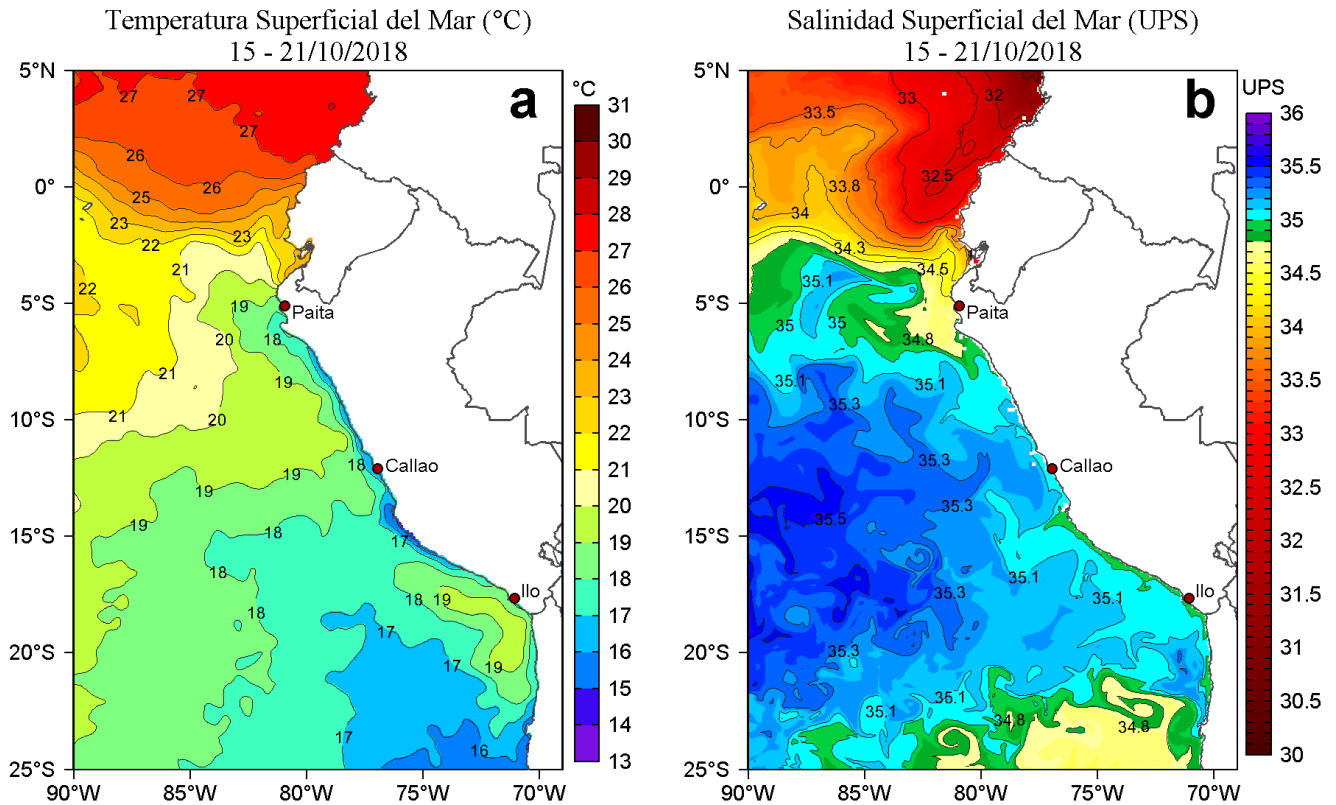
Figura 1. Distribución espacial promedio de: a) Temperatura Superficial del Mar (TSM, °C) y b) Salinidad Superficial del Mar (SSM, UPS) para la semana del 15 al 21 de octubre de 2018 en el océano Pacífico tropical oriental. Datos: OSTIA-UKMO-L4-GLOB-v2.0 (UK Met Office, 2012; Donlon et al, 2012) disponible en https://podaac.jpl.nasa.gov/dataset/OSTIA-UKMO-L4-GLOB-v2.0 para (a) y del Hybrid Coordinate Ocean Model (HYCOM; Halliwell et al., 1998; 2000; Bleck, 2001) para (b). Las escalas de colores de la TSM como de la SSM se presentan a la derecha de cada gráfico. Procesamiento: LHF/AFIOF/DGIOCC/IMARPE.
