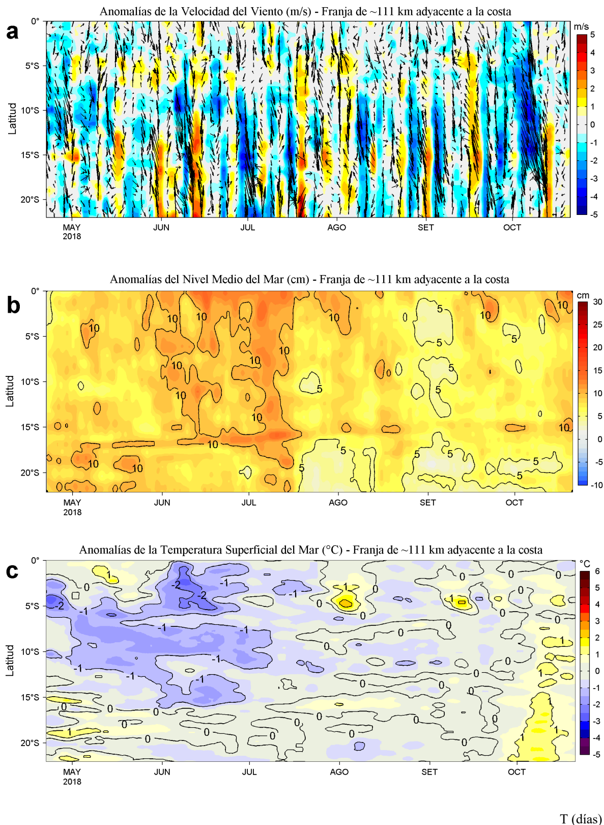
Figura 4. Evolución de las anomalías diarias de: a) Velocidad del viento (m/s), b) Nivel medio del mar (cm), c) Temperatura Superficial del Mar (°C) para el último semestre actualizado al 21 de octubre de 2018. Datos: de IFREMER/CERSAT para (a), del Servicio de Monitoreo del Ambiente Marino Copernicus (CMEMS, según sus siglas en inglés) para (b), de OSTIA-UKMO-L4-GLOB-v2.0 para (c). Las anomalías fueron calculadas para una franja de 111 km adyacente a la costa entre el ecuador y 22°S según los promedios climatológicos diarios de 2000-2014 para (a), de 1993-2013 para (b) y de 2007-2016 para (c). La barra de colores a la derecha muestra la escala de las anomalías en cada caso. Procesamiento: LHF/AFIOF/DGIOCC/MARPE.
