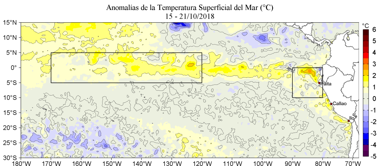
Figura 2. Anomalías promedio de la Temperatura Superficial del Mar (°C) en el océano Pacífico tropical para la semana del 15 al 21 de octubre de 2018. Las regiones Niño 3.4 y Niño 1+2 en los sectores central y oriental del océano, respectivamente están delimitadas con una línea de color gris. Datos: OSTIA-UKMO-L4-GLOB-v2.0 (UK Met Office, 2012; Donlon et al, 2012) disponible en https://podaac.jpl.nasa.gov/dataset/OSTIA-UKMO-L4-GLOB-v2.0 . Las anomalías se calcularon con respecto de la climatología para el período 2007-2016. Procesamiento: LHF/AFIOF/DGIOCC/IMARPE.
