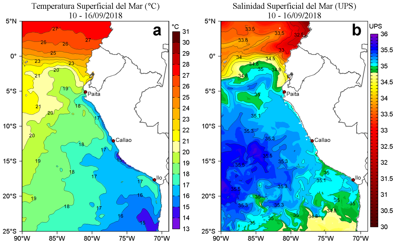
Figura 1. Distribución espacial promedio de: a) Temperatura Superficial del Mar (TSM, °C) y b) Salinidad Superficial del Mar (SSM, UPS) para la semana del 10 al 16 de setiembre de 2018 en el océano Pacífico tropical oriental. Datos: OSTIA-UKMO-L4-GLOB-v2.0 (UK Met Office, 2012; Donlon et al, 2012) disponible en https://podaac.jpl.nasa.gov/dataset/OSTIA-UKMO-L4-GLOB-v2.0 para (a) y del Hybrid Coordinate Ocean Model (HYCOM; Halliwell et al., 1998; 2000; Bleck, 2001) para (b). Las escalas de colores de la TSM como de la SSM se presentan a la derecha de cada gráfico. Procesamiento: LHF/AFIOF/DGIOCC/IMARPE.
