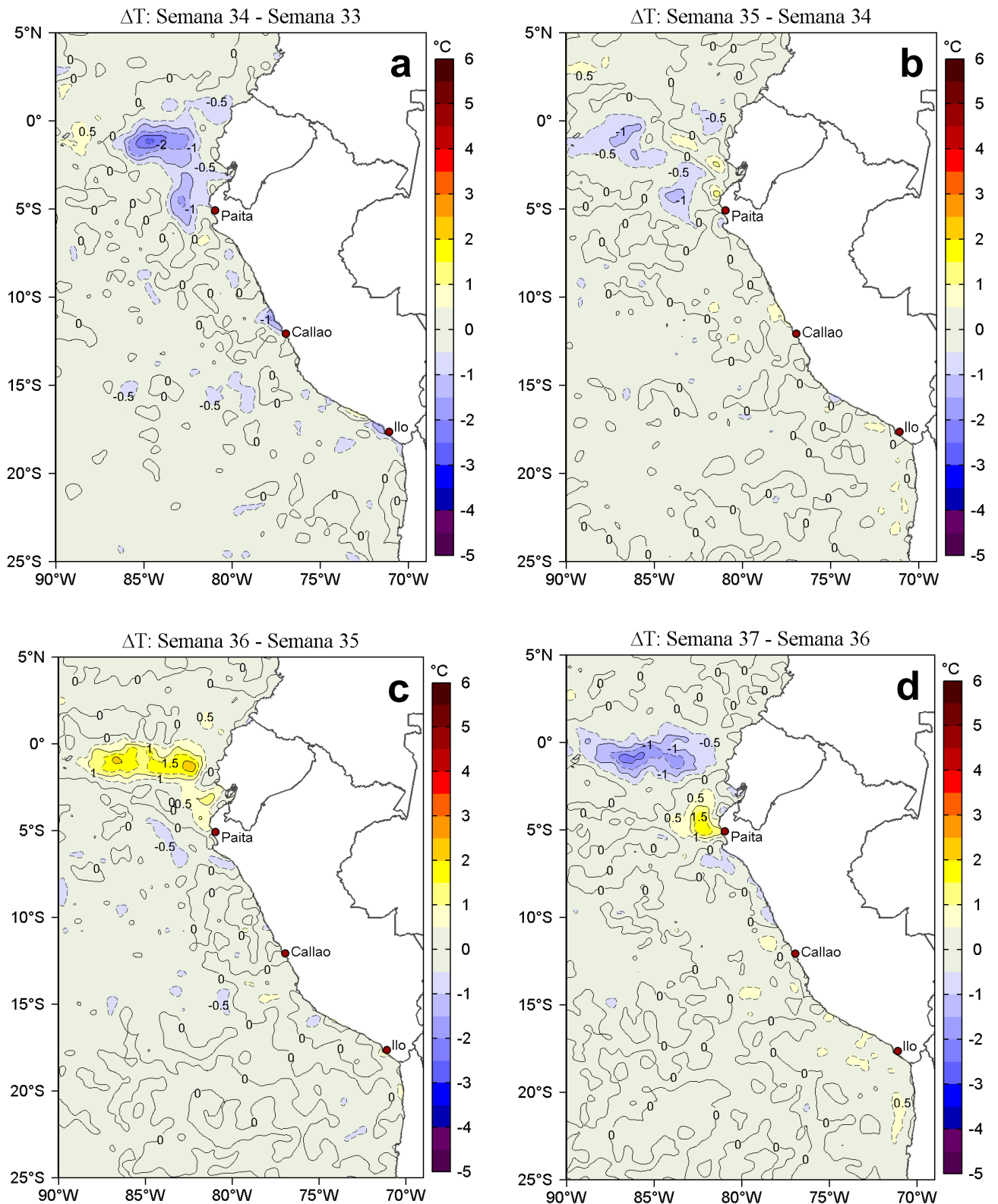
Figura 3. Variación semanal de la Temperatura Superficial del Mar (°C) en el océano Pacífico tropical oriental entre: a) trigésimo cuarta (20-26 de agosto) y trigésimo tercera (13-19 de agosto) semana del 2018, b) trigésimo quinta (27 de agosto - 02 de setiembre) y trigésimo cuarta (20-26 de agosto) semana del 2018, c) trigésimo sexta (03-09 de setiembre) y trigésimo quinta (27 de agosto - 02 de setiembre) semana del 2018 y d) trigésimo séptima (10-16 de setiembre) y trigésimo sexta (03-09 de setiembre) semana del 2018. Los mapas, que indican el grado de calentamiento o enfriamiento de una semana a otra, provienen de OSTIA-UKMO-L4-GLOB-v2.0 (UK Met Office, 2012; Donlon et al, 2012). La barra de colores a la derecha muestra la diferencia de la temperatura entre la presente y la semana previa. Procesamiento: LHFM/AFIOF/DGIOCC/IMARPE.
