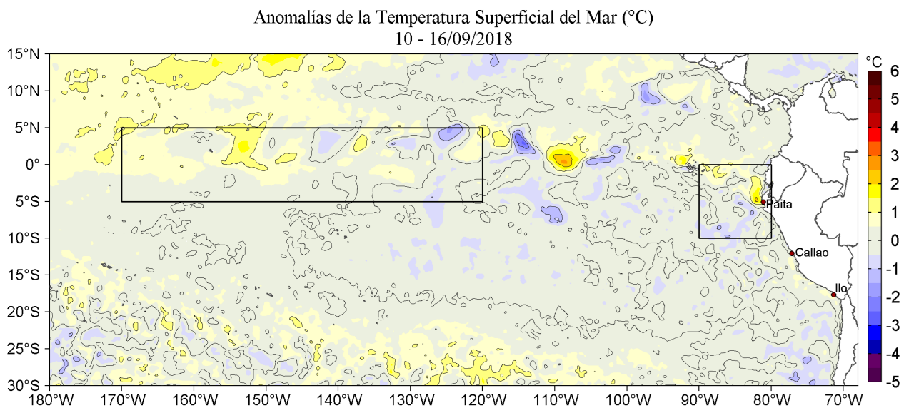
Figura 2. Anomalías promedio de la Temperatura Superficial del Mar (°C) en el océano Pacífico tropical para la semana del 10 al 16 de setiembre de 2018. Las regiones Niño 3.4 y Niño 1+2 en los sectores central y oriental del océano, respectivamente están delimitadas con una línea de color gris. Datos: OSTIA-UKMO-L4-GLOB-v2.0 (UK Met Office, 2012; Donlon et al, 2012) disponible en https://podaac.jpl.nasa.gov/dataset/OSTIA-UKMO-L4-GLOB-v2.0 . Las anomalías se calcularon con respecto de la climatología para el período 2007-2016. Procesamiento: LHF/AFIOF/DGIOCC/IMARPE.
