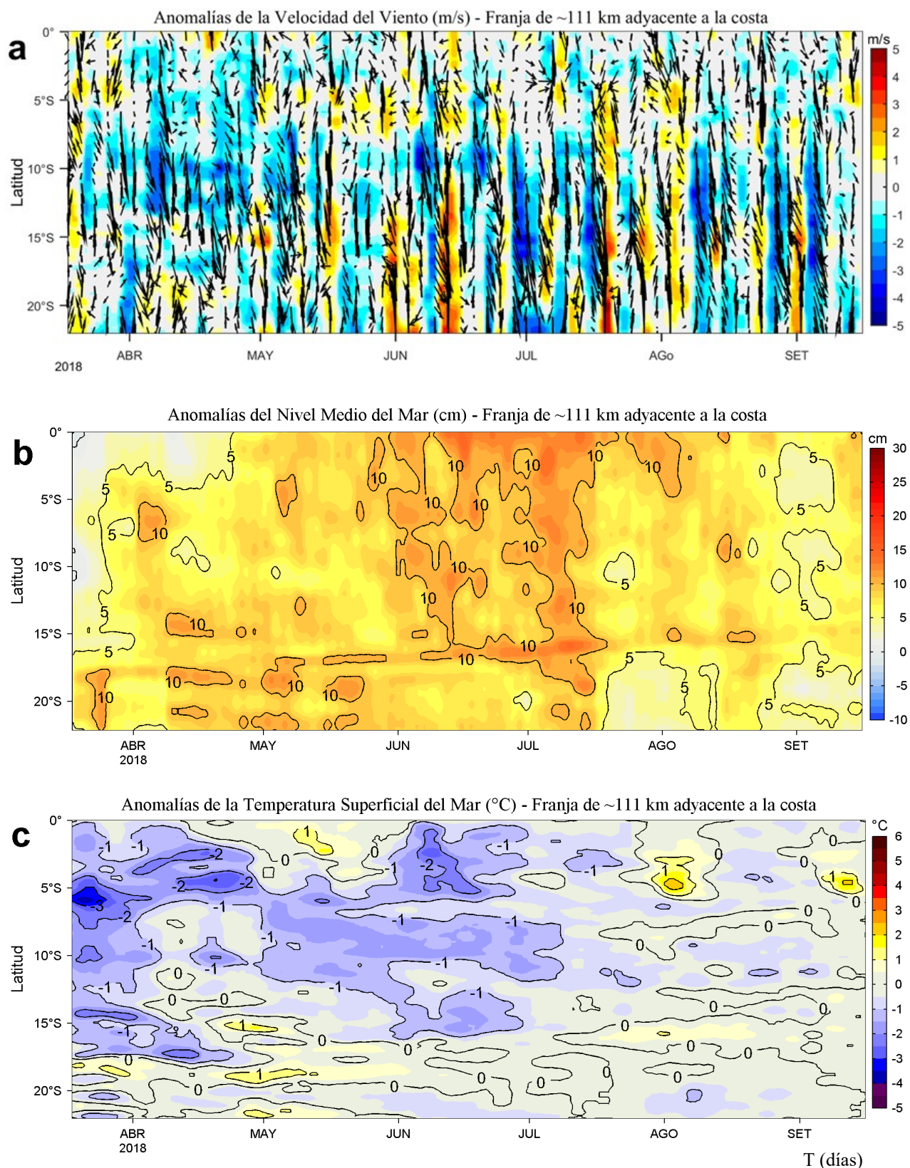
Figura 4. Evolución de las anomalías diarias de: a) Velocidad del viento (m/s), b) Nivel medio del mar (cm), c) Temperatura Superficial del Mar (°C) para el último semestre actualizado al 16 de setiembre de 2018. Datos: de IFREMER/CERSAT para (a), del Servicio de Monitoreo del Ambiente Marino Copernicus (CMEMS, según sus siglas en inglés) para (b), de OSTIA-UKMO-L4-GLOB-v2.0 para (c). Las anomalías fueron calculadas para una franja de 111 km adyacente a la costa entre el ecuador y 22°S según los promedios climatológicos diarios de 2000-2014 para (a), de 1993-2013 para (b) y de 2007-2016 para (c). La barra de colores a la derecha muestra la escala de las anomalías en cada caso. Procesamiento: LHF/AFIOF/DGIOCC/IMARPE.
