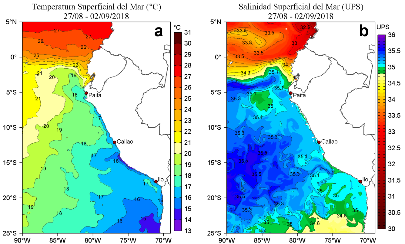
Figura 1. Distribución espacial promedio de: a) Temperatura Superficial del Mar (TSM, °C) y b) Salinidad Superficial del Mar (SSM, UPS) para la semana del 27 de agosto al 02 de setiembre de 2018 en el océano Pacífico tropical oriental. Datos: OSTIA-UKMO-L4-GLOB-v2.0 (UK Met Office, 2012; Donlon et al, 2012) disponible en https://podaac.jpl.nasa.gov/dataset/OSTIA-UKMO-L4-GLOB-v2.0 ) para (a) y del Hybrid Coordinate Ocean Model (HYCOM; Halliwell et al., 1998; 2000; Bleck, 2001) para (b). Las escalas de colores de la TSM como de la SSM se presentan a la derecha de cada gráfico. Procesamiento: LHF/AFIOF/DGIOCC/IMARPE.
