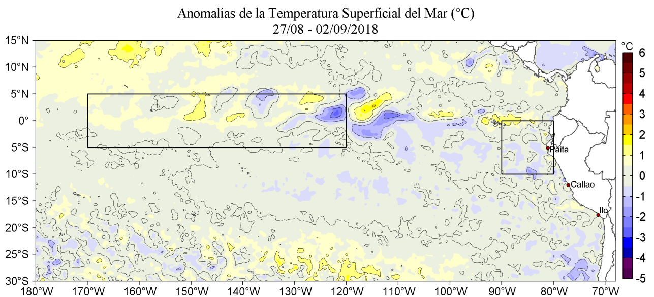
Figura 2. Anomalías promedio de la Temperatura Superficial del Mar (°C) en el océano Pacífico tropical para la semana del 27 de agosto al 02 de setiembre de 2018. Las regiones Niño 3.4 y Niño 1+2 en los sectores central y oriental del océano, respectivamente están delimitadas con una línea de color gris. Datos: OSTIA-UKMO-L4-GLOB-v2.0 (UK Met Office, 2012; Donlon et al, 2012) disponible en https://podaac.jpl.nasa.gov/dataset/OSTIA-UKMO-L4-GLOB-v2.0 ). Las anomalías se calcularon con respecto de la climatología para el período 2007-2016. Procesamiento: LHF/AFIOF/DGIOCC/IMARPE.
