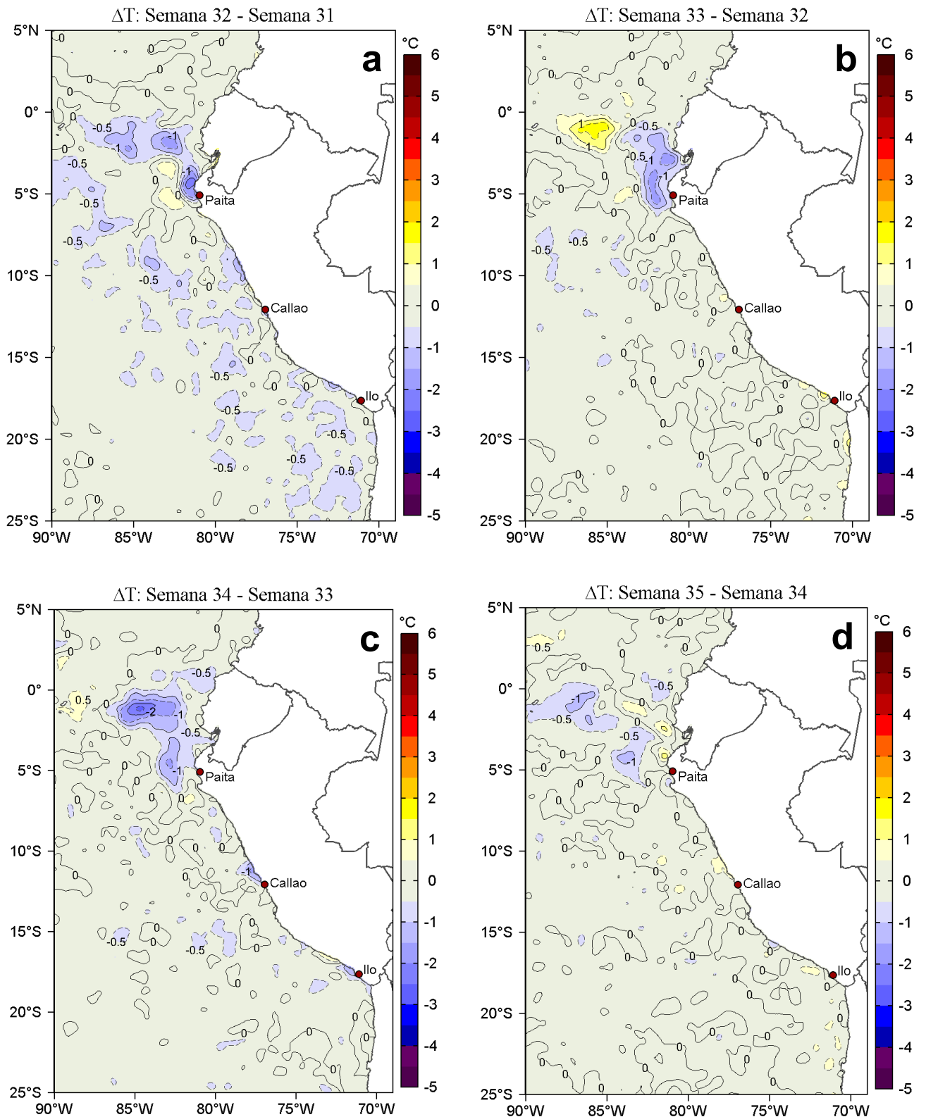
Figura 3. Variación semanal de la Temperatura Superficial del Mar ( ^{\circ}\text{C} ) en el océano Pacífico tropical oriental entre: a) trigésimo segunda (06-12 de agosto) y trigésimo primera (30 de julio - 05 de agosto) semana del 2018, b) trigésimo tercera (13-19 de agosto) y trigésimo segunda (06-12 de agosto) semana del 2018, c) trigésimo cuarta (20-26 de agosto) y trigésimo tercera (13-19 de agosto) semana del 2018 y d) trigésimo quinta (27 de agosto - 02 de setiembre) y trigésimo cuarta (20-26 de agosto) semana del 2018.
