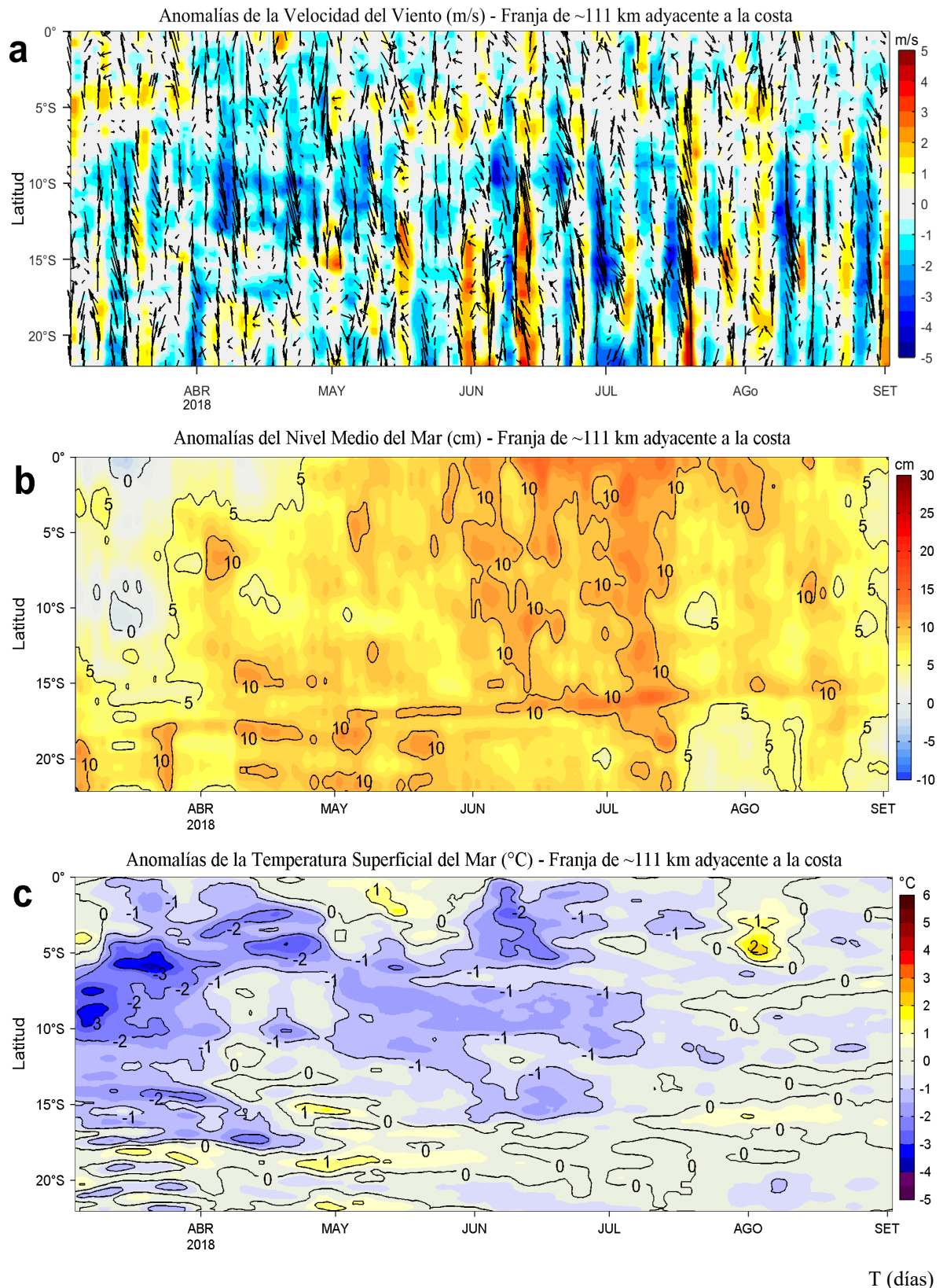
Figura 4. Evolución de las anomalías diarias de: a) Velocidad del viento (m/s), b) Nivel medio del mar (cm), c) Temperatura Superficial del Mar (°C) para el último semestre actualizado al 02 de setiembre de 2018. Datos: de IFREMER/CERSAT para (a), del Servicio de Monitoreo del Ambiente Marino Copernicus (CMEMS, según sus siglas en inglés) para (b), de OSTIA-UKMO-L4-GLOB-v2.0 para (c). Las anomalías fueron calculadas para una franja de 111 km adyacente a la costa entre el ecuador y 22°S según los promedios climatológicos diarios de 2000-2014 para (a), de 1993-2013 para (b) y de 2007-2016 para (c). La barra de colores a la derecha muestra la escala de las anomalías en cada caso. Procesamiento: LHF/AFIOF/DGIOCC/IMARPE.
