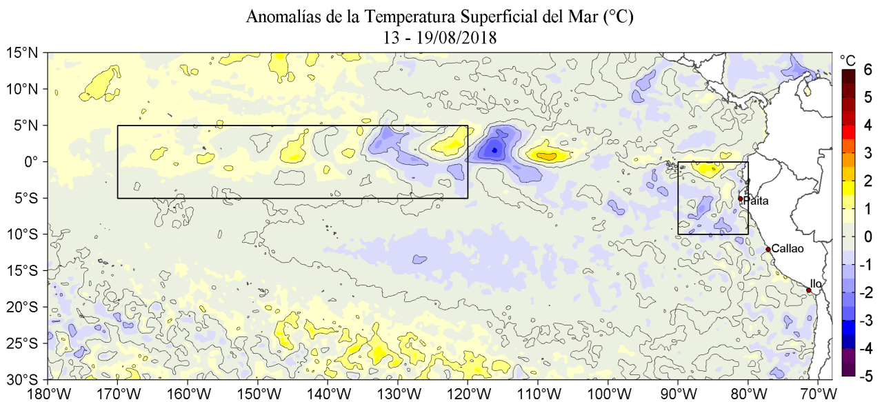
Figura 2. Anomalías promedio de la Temperatura Superficial del Mar (°C) en el océano Pacífico tropical para la semana del 13 al 19 de agosto de 2018. Las regiones Niño 3.4 y Niño 1+2 en los sectores central y oriental del océano, respectivamente están delimitadas con una línea de color gris. Datos: OSTIA-UKMO-L4-GLOB-v2.0 (UK Met Office, 2012; Donlon et al, 2012) disponible en https://podaac.jpl.nasa.gov/dataset/OSTIA-UKMO-L4-GLOB-v2.0 ). Las anomalías se calcularon con respecto de la climatología para el período 2007-2016. Procesamiento: LHF/AFIOF/DGIOCC/IMARPE.
