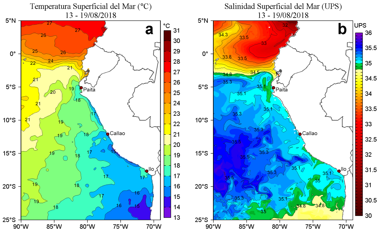
Figura 1. Distribución espacial promedio de: a) Temperatura Superficial del Mar (TSM, °C) y b) Salinidad Superficial del Mar (SSM, UPS) para la semana del 13 al 19 de agosto de 2018 en el océano Pacífico tropical oriental. Datos: OSTIA-UKMO-L4-GLOB-v2.0 (UK Met Office, 2012; Donlon et al, 2012) disponible en https://podaac.jpl.nasa.gov/dataset/OSTIA-UKMO-L4-GLOB-v2.0 para (a) y del Hybrid Coordinate Ocean Model (HYCOM; Halliwell et al., 1998; 2000; Bleck, 2001) para (b). Las escalas de colores de la TSM como de la SSM se presentan a la derecha de cada gráfico. Procesamiento: LHF/AFIOF/DGIOCC/IMARPE.
