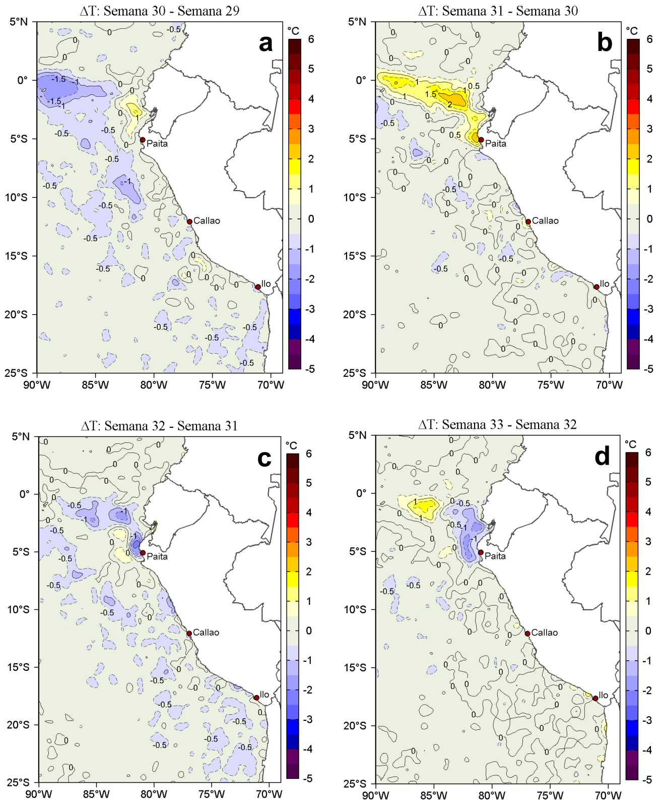
Figura 3. Variación semanal de la Temperatura Superficial del Mar ( ^{\circ}\text{C} ) en el océano Pacífico tropical oriental entre: a) trigésima (23-29 de julio) y vigésimo novena (16-22 de julio) semana del 2018, b) trigésimo primera (30 de julio - 05 de agosto) y trigésima (23-29 de julio) semana del 2018, c) trigésimo segunda (06-12 de agosto) y trigésimo primera (30 de julio - 05 de agosto) semana del 2018 y d) trigésimo tercera (13-19 de agosto) y trigésimo segunda (06-12 de agosto) semana del 2018. Los mapas, que indican el grado de calentamiento o enfriamiento de una semana a otra, provienen de OSTIA-UKMO-L4-GLOB-v2.0 (UK Met Office, 2012; Donlon et al, 2012). La barra de colores a la derecha muestra la diferencia de la temperatura entre la presente y la semana previa. Procesamiento: LHFM/AFIOF/DGIOCC/IMARPE.
