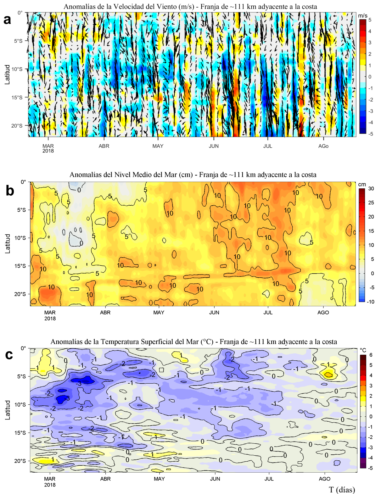
Figura 4. Evolución de las anomalías diarias de: a) Velocidad del viento (m/s), b) Nivel medio del mar (cm), c) Temperatura Superficial del Mar (°C) para el último semestre actualizado al 19 de agosto de 2018. Datos: de IFREMER/CERSAT para (a), del Servicio de Monitoreo del Ambiente Marino Copernicus (CMEMS, según sus siglas en inglés) para (b), de OSTIA-UKMO-L4-GLOB-v2.0 para (c). Las anomalías fueron calculadas para una franja de 111 km adyacente a la costa entre el ecuador y 22°S según los promedios climatológicos diarios de 2000-2014 para (a), de 1993-2013 para (b) y de 2007-2016 para (c). La barra de colores a la derecha muestra la escala de las anomalías en cada caso. Procesamiento: LHFM/AFIOF/DGIOCC/MARPE.
