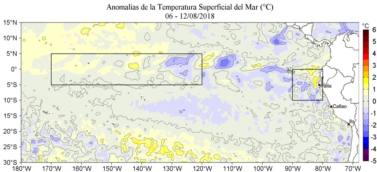
Figura 2. Anomalías promedio de la Temperatura Superficial del Mar (°C) en el océano Pacífico tropical para la semana del 06 al 12 de agosto de 2018. Las regiones Niño 3.4 y Niño 1+2 en los sectores central y oriental del océano, respectivamente están delimitadas con una línea de color gris. Datos: OSTIA-UKMO-L4-GLOB-v2.0 (UK Met Office, 2012; Donlon et al, 2012) disponible en https://podaac.jpl.nasa.gov/dataset/OSTIA-UKMO-L4-GLOB-v2.0 . Las anomalías se calcularon con respecto de la climatología para el período 2007-2016. Procesamiento: LHF/AFIOF/DGIOCC/IMARPE.
