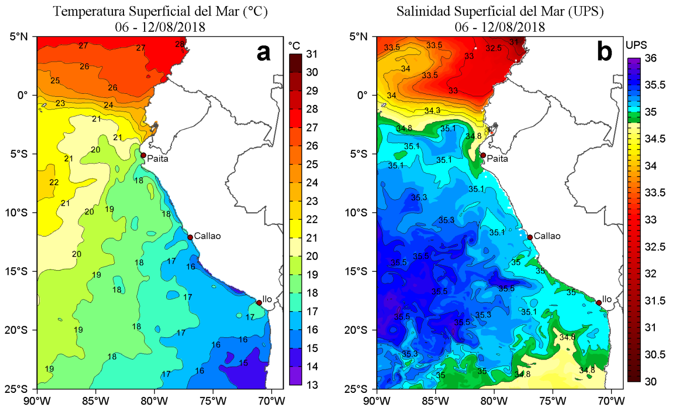
Figura 1. Distribución espacial promedio de: a) Temperatura Superficial del Mar (TSM, °C) y b) Salinidad Superficial del Mar (SSM, UPS) para la semana del 06 al 12 de agosto de 2018 en el océano Pacífico tropical oriental. Datos: OSTIA-UKMO-L4-GLOB-v2.0 (UK Met Office, 2012; Donlon et al, 2012) disponible en https://podaac.jpl.nasa.gov/dataset/OSTIA-UKMO-L4-GLOB-v2.0 para (a) y del Hybrid Coordinate Ocean Model (HYCOM; Halliwell et al., 1998; 2000; Bleck, 2001) para (b). Las escalas de colores de la TSM como de la SSM se presentan a la derecha de cada gráfico. Procesamiento: LHF/AFIOF/DGIOCC/IMARPE.
