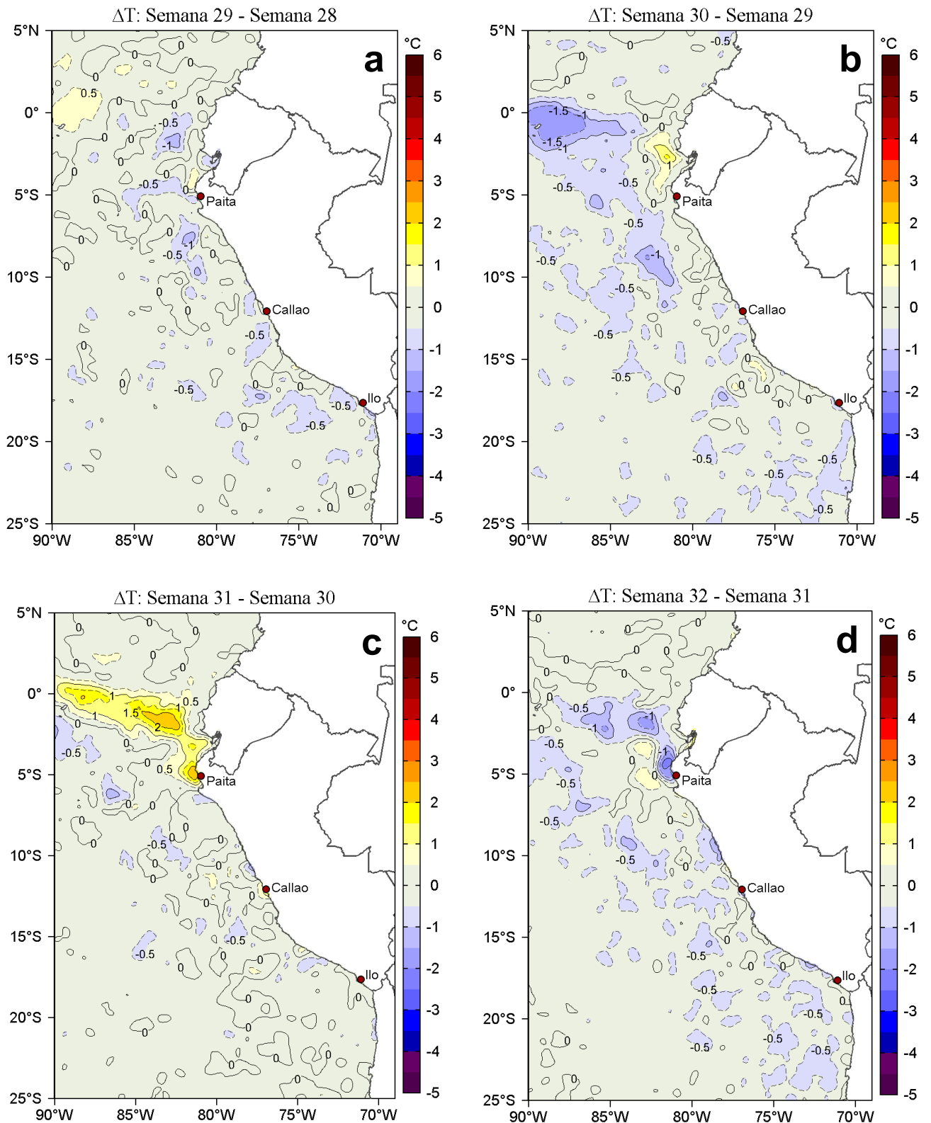
Figura 3. Variación semanal de la Temperatura Superficial del Mar ( ^{\circ}\text{C} ) en el océano Pacífico tropical oriental entre: a) vigésimo novena (16-22 de julio) y vigésimo octava (09-15 de julio) semana del 2018, b) trigésima (23-29 de julio) y vigésimo novena (16-22 de julio) semana del 2018, c) trigésimo primera (30 de julio - 05 de agosto) y trigésima (23-29 de julio) semana del 2018 y d) trigésimo segunda (06-12 de agosto) y trigésimo primera (30 de julio - 05 de agosto) semana del 2018. Los mapas, que indican el grado de calentamiento o enfriamiento de una semana a otra, provienen de OSTIA-UKMO-L4-GLOB-v2.0 (UK Met Office, 2012; Donlon et al, 2012). La barra de colores a la derecha muestra la diferencia de la temperatura entre la presente y la semana previa. Procesamiento: LHFM/AFIOF/DGIOCC/IMARPE.
