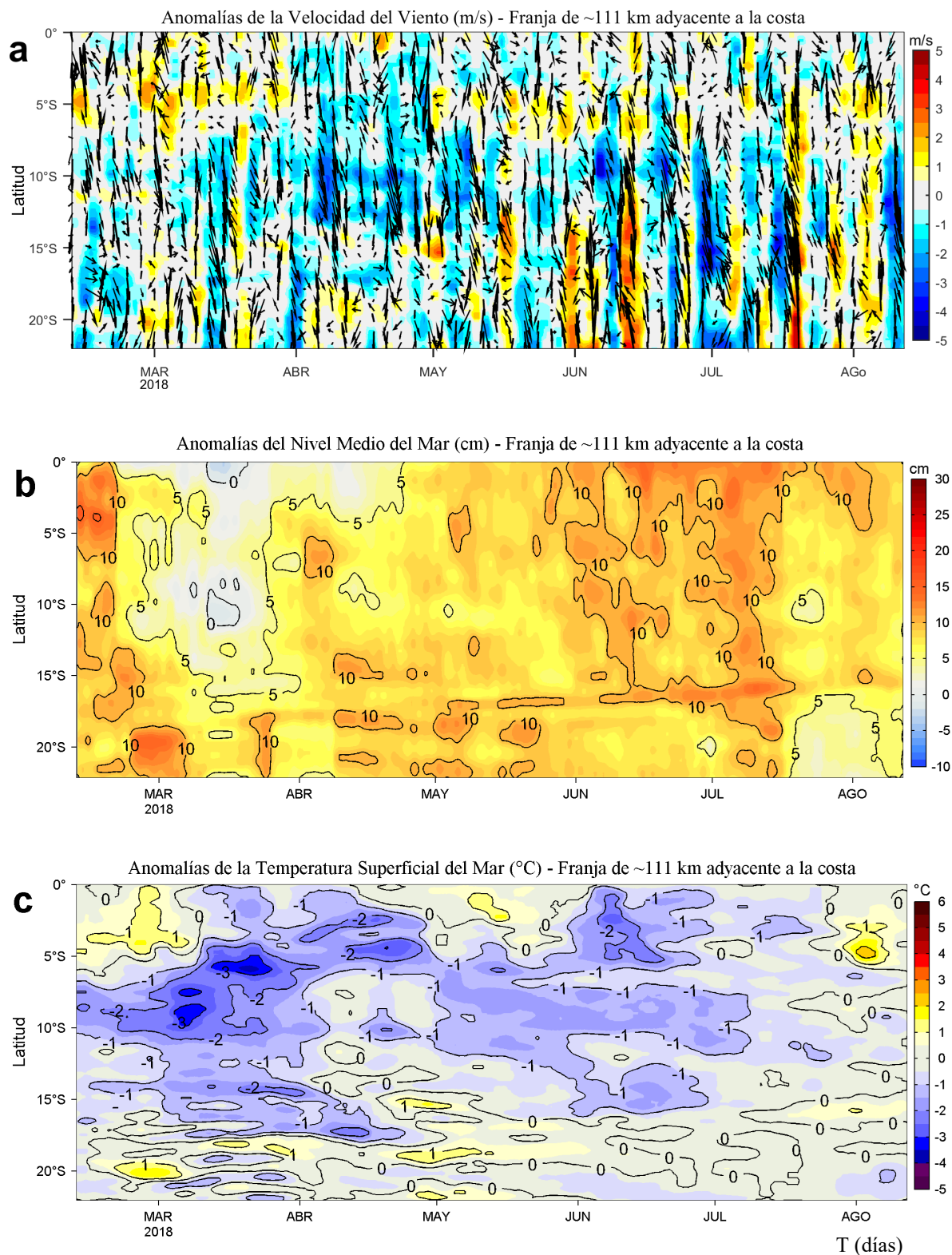
Figura 4. Evolución de las anomalías diarias de: a) Velocidad del viento (m/s), b) Nivel medio del mar (cm), c) Temperatura Superficial del Mar (°C) para el último semestre actualizado al 12 de agosto de 2018. Datos: de IFREMER/CERSAT para (a), del Servicio de Monitoreo del Ambiente Marino Copernicus (CMEMS, según sus siglas en inglés) para (b), de OSTIA-UKMO-L4-GLOB-v2.0 para (c). Las anomalías fueron calculadas para una franja de 111 km adyacente a la costa entre el ecuador y 22°S según los promedios climatológicos diarios de 2000-2014 para (a), de 1993-2013 para (b) y de 2007-2016 para (c). La barra de colores a la derecha muestra la escala de las anomalías en cada caso. Procesamiento: LHF/AFIOF/DGIOCC/IMARPE.
