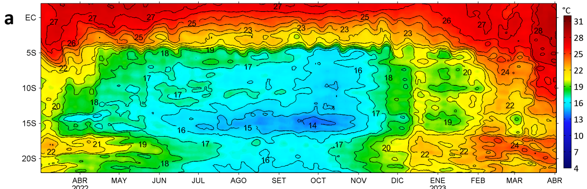
Anomalías de la Temperatura Superficial del mar (°C), franja costera de 60 m.n. 02 de marzo 2022 - 02 de abril 2023
