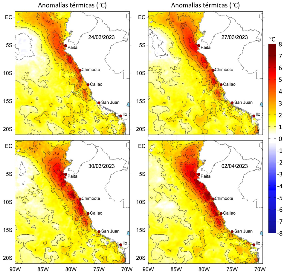
Figura 3. Anomalías de la temperatura superficial del mar ( ^{\circ}\text{C} ) para el a) 24, b) 27 y c) 30 de marzo, así como para el d) 02 de abril de 2023. Las anomalías se calcularon respecto de la climatología para el periodo 2007-2016. Datos: OSTIA-UKMO-L4-GLOB-v2.0 (UK Met Office, 2012; Donlon et al, 2012).
