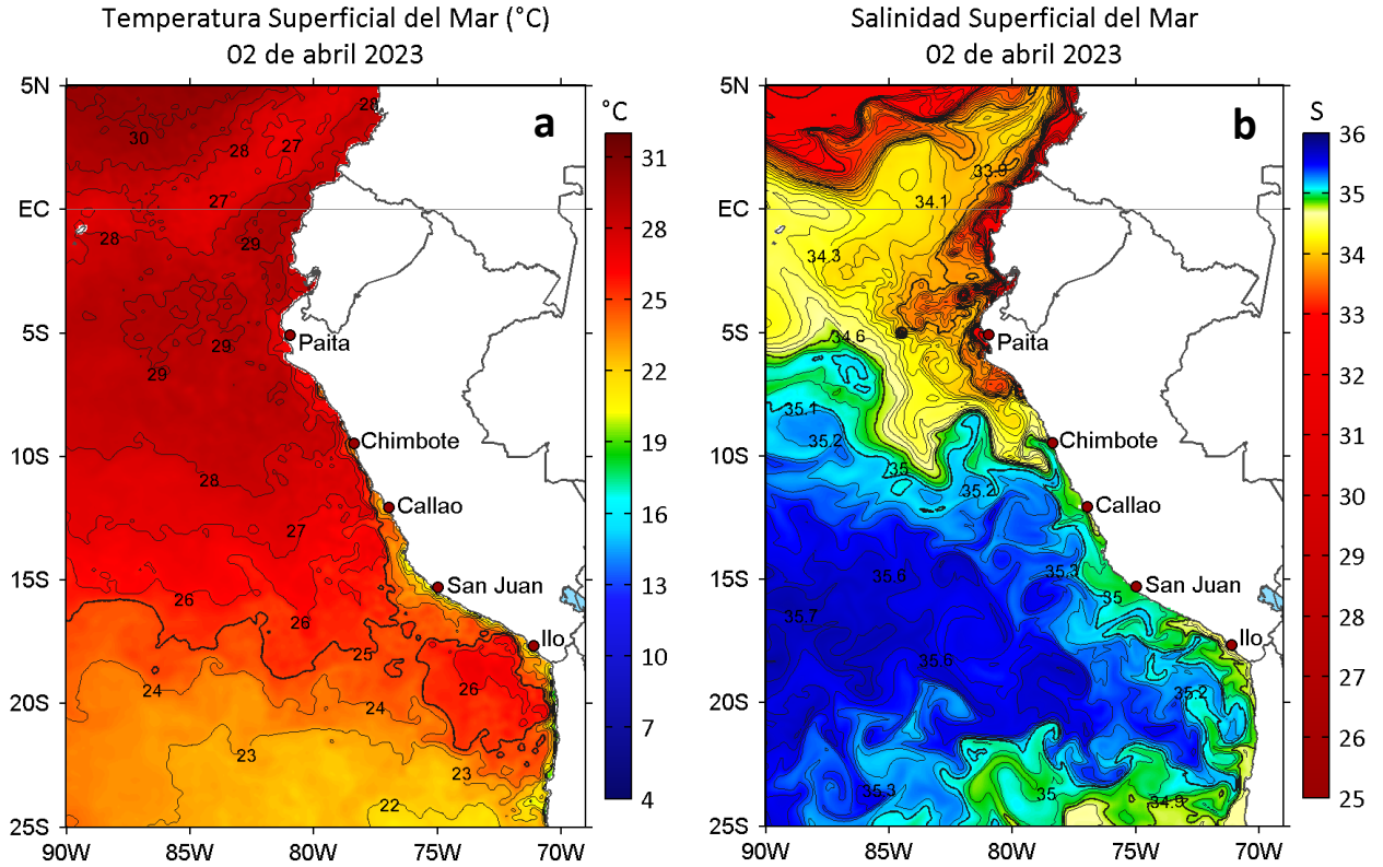
Figura 2. a) Temperatura superficial del mar ( ^{\circ}\text{C} ) y b) Salinidad superficial del mar para el 02 de abril de 2023. Datos: OSTIA-UKMO-L4-GLOB-v2.0 (UK Met Office, 2012; Donlon et al, 2012) y del GLOBAL_ANALYSIS_FORECAST_PHY_001_024 (Lellouche, J. M. et al, 2013), respectivamente.
