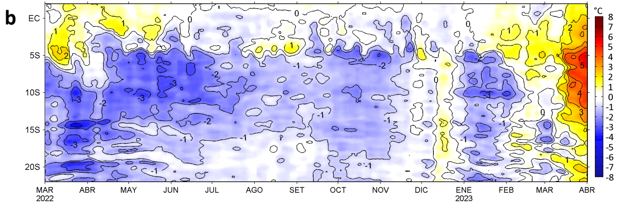
Anomalías de la Temperatura Superficial del mar (°C), franja costera de 60 m.n. 01 de marzo 2022 - 01 de abril 2023
