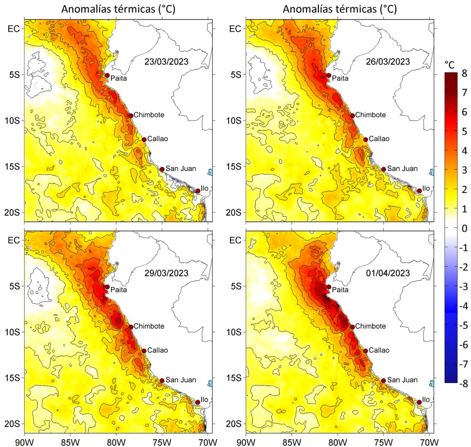
Figura 3. Anomalías de la temperatura superficial del mar ( ^{\circ}\text{C} ) para el a) 23, b) 26 y c) 29 de marzo, así como para el d) 01 de abril de 2023. Las anomalías se calcularon respecto de la climatología para el periodo 2007-2016. Datos: OSTIA-UKMO-L4-GLOB-v2.0 (UK Met Office, 2012; Donlon et al, 2012).
