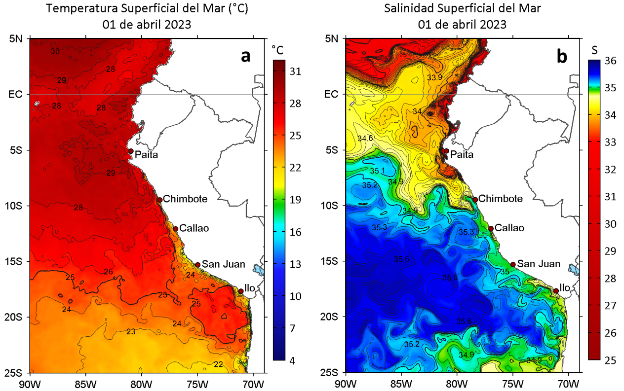
Figura 2. a) Temperatura superficial del mar ( ^{\circ}\text{C} ) y b) Salinidad superficial del mar para el 01 de abril de 2023. Datos: OSTIA-UKMO-L4-GLOB-v2.0 (UK Met Office, 2012; Donlon et al, 2012) y del GLOBAL_ANALYSIS_FORECAST_PHY_001_024 (Lellouche, J. M. et al, 2013), respectivamente.
