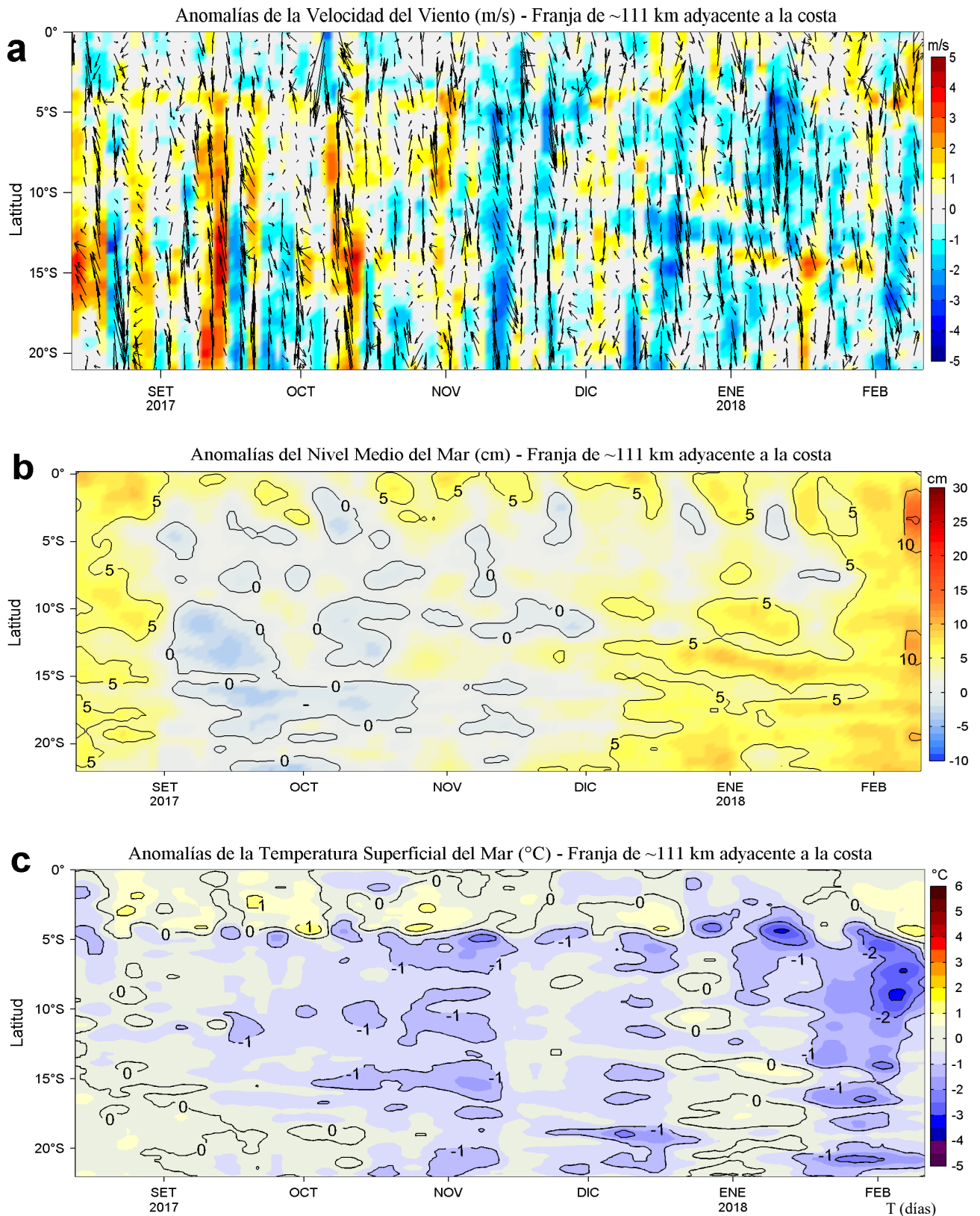
Figura 4. Evolución de las anomalías diarias de: a) Velocidad del viento (m/s), b) Nivel medio del mar (cm), c) Temperatura Superficial del Mar (°C) para el último semestre actualizado al 11 de febrero de 2018. Datos: de IFREMER/CERSAT para (a), del Servicio de Monitoreo del Ambiente Marino Copernicus (CMEMS, según sus siglas en inglés) para (b), de OSTIA-UKMO-L4-GLOB-v2.0 para (c). Las anomalías fueron calculadas para una franja de 111 km adyacente a la costa entre el ecuador y 22°S según los promedios climatológicos diarios de 2000-2014 para (a), de 1993-2013 para (b) y de 2007-2016 para (c). La barra de colores a la derecha muestra la escala de las anomalías en cada caso. Procesamiento: LHF/M/AFIOF/DGIOCC/IMARPE.
