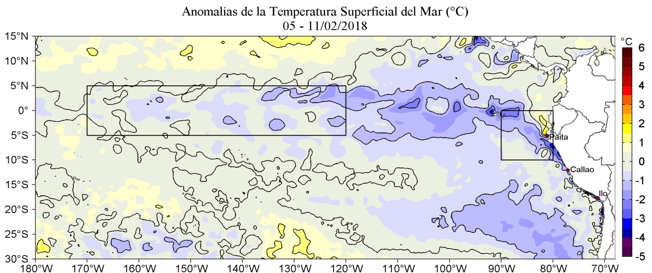
Figura 2. Anomalías promedio de la Temperatura Superficial del Mar (°C) en el océano Pacífico tropical para la semana del 05 al 11 de febrero de 2018. Las regiones Niño 3.4 y Niño 1+2 en los sectores central y oriental del océano, respectivamente están delimitadas con una línea de color gris. Datos: OSTIA-UKMO-L4-GLOB-v2.0 (UK Met Office, 2012; Donlon et al, 2012) disponible en https://podaac.jpl.nasa.gov/dataset/OSTIA-UKMO-L4-GLOB-v2.0 . Las anomalías se calcularon con respecto de la climatología para el período 2007-2016. Procesamiento: LHFM/AFIOF/DGIOCC/IMARPE.
