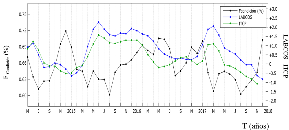
Figura 7. Series de tiempo mensual del Índice LABCOS (línea punteada de color azul), del Índice Térmico Costero Peruano (ITCP, línea de color verde) y el Factor de Condición (%), en color negro) desde mayo de 2014. La metodología para estimar estos índices se encuentran en Quispe y Vásquez (2015), Quispe et al (2016), Takahashi, et al. (2014) y Perea et al (2015), respectivamente. Procesamiento: LHF/AFIOF/DGIOCC/IMARPE.
