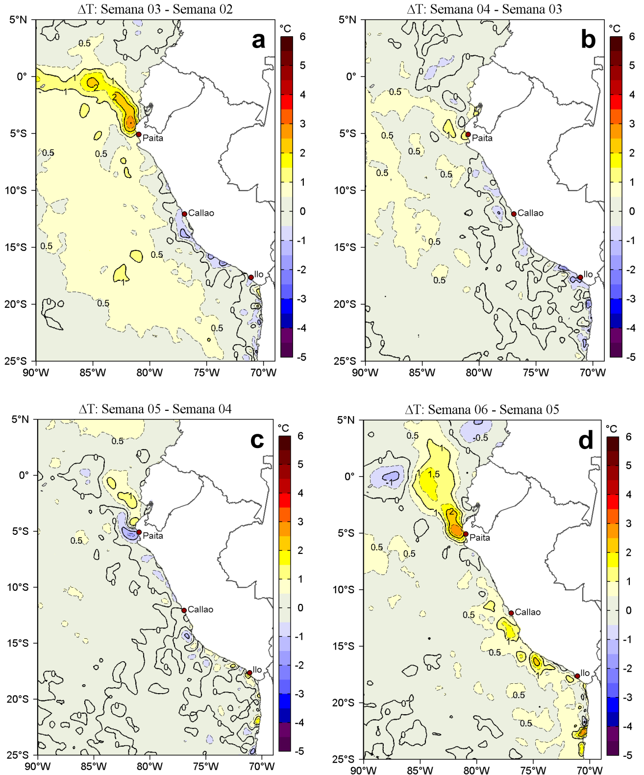
Figura 3. Variación semanal de la Temperatura Superficial del Mar ( ^{\circ}\text{C} ) en el océano Pacífico tropical oriental entre: a) la tercera (15-21 de enero) y segunda (08-14 de enero) semana del 2018, b) la cuarta (22-28 de enero) y tercera (15-21 de enero) semana del 2018, c) la quinta (29 de enero - 04 de febrero) y cuarta (22-28 de enero) semana del 2018, y d) la sexta (05-11 de febrero) y quinta (29 de enero - 04 de febrero) semana del 2018.
