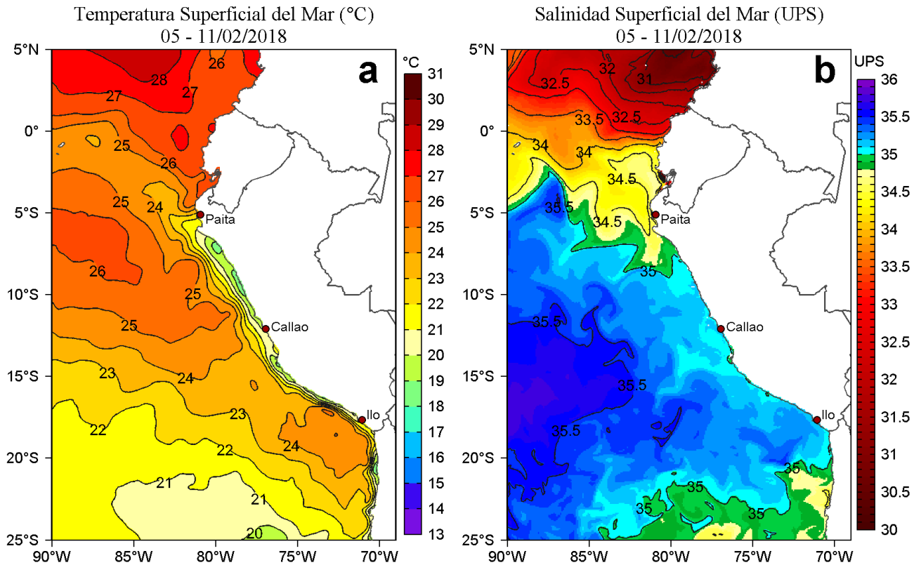
Figura 1. Distribución espacial promedio de: a) Temperatura Superficial del Mar (TSM, °C) y b) Salinidad Superficial del Mar (SSM, UPS) para la semana del 05 al 11 de febrero de 2018 en el océano Pacífico tropical oriental. Datos: OSTIA-UKMO-L4-GLOB-v2.0 (UK Met Office, 2012; Donlon et al, 2012) disponible en https://podaac.jpl.nasa.gov/dataset/OSTIA-UKMO-L4-GLOB-v2.0 para (a) y del Hybrid Coordinate Ocean Model (HYCOM; Halliwell et al., 1998; 2000; Bleck, 2001) para (b). Las escalas de colores de la TSM como de la SSM se presentan a la derecha de cada gráfico. Procesamiento: LHFM/AFIOF/DGIOCC/IMARPE.
