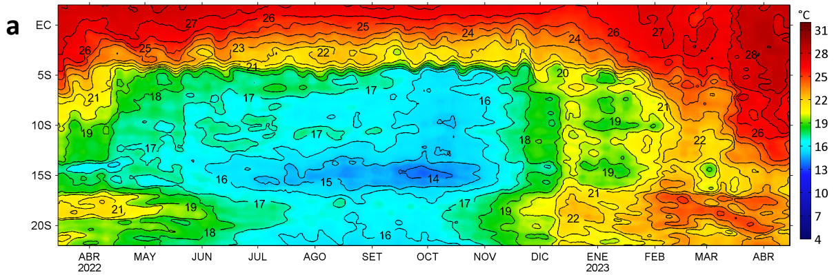
Anomalías de la Temperatura Superficial del mar (°C), franja costera de 60 m.n. 15 de marzo 2022 - 15 de abril 2023
