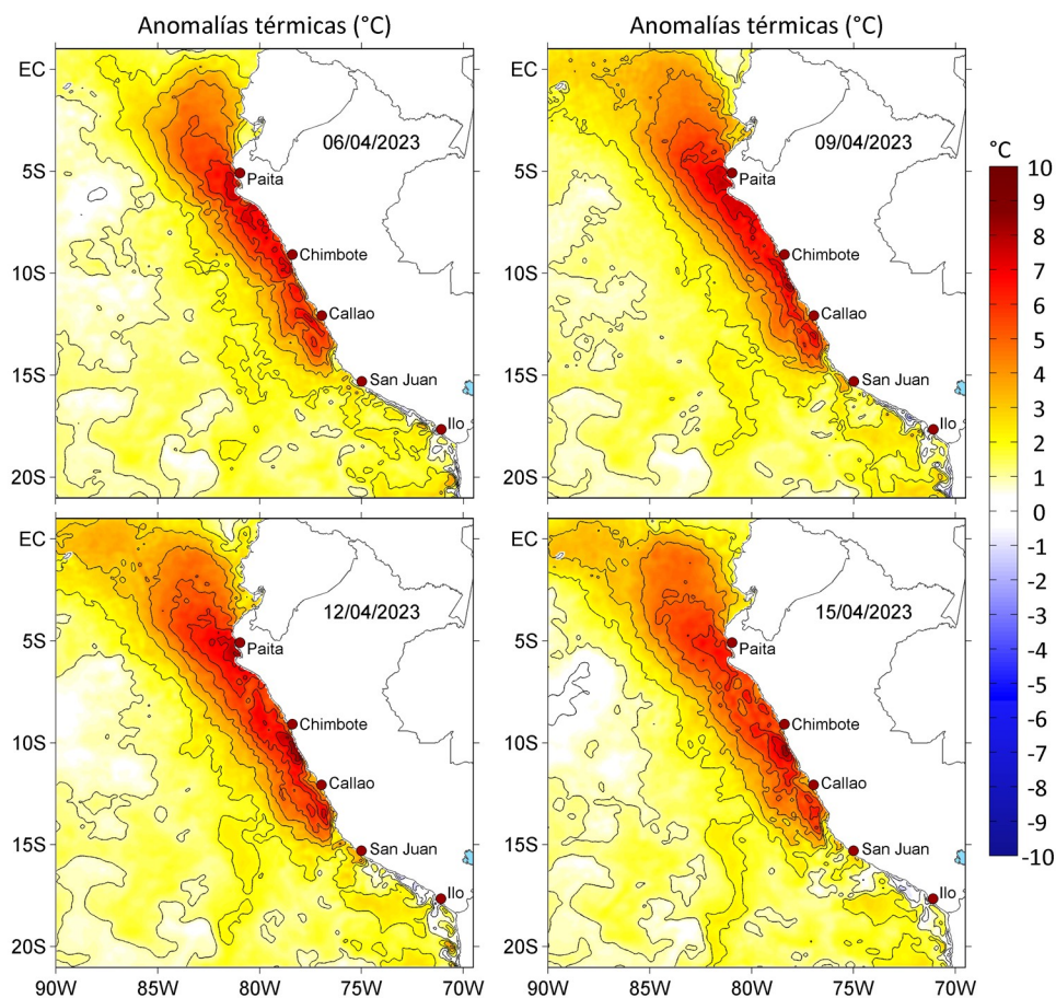
Figura 3. Anomalías de la temperatura superficial del mar ( ^{\circ}\text{C} ) para el a) 06, b) 09, c) 12 y d) 15 de abril de 2023. Las anomalías se calcularon respecto de la climatología para el periodo 2007-2016. Datos: OSTIA-UKMO-L4-GLOB-v2.0 (UK Met Office, 2012; Donlon et al, 2012).
