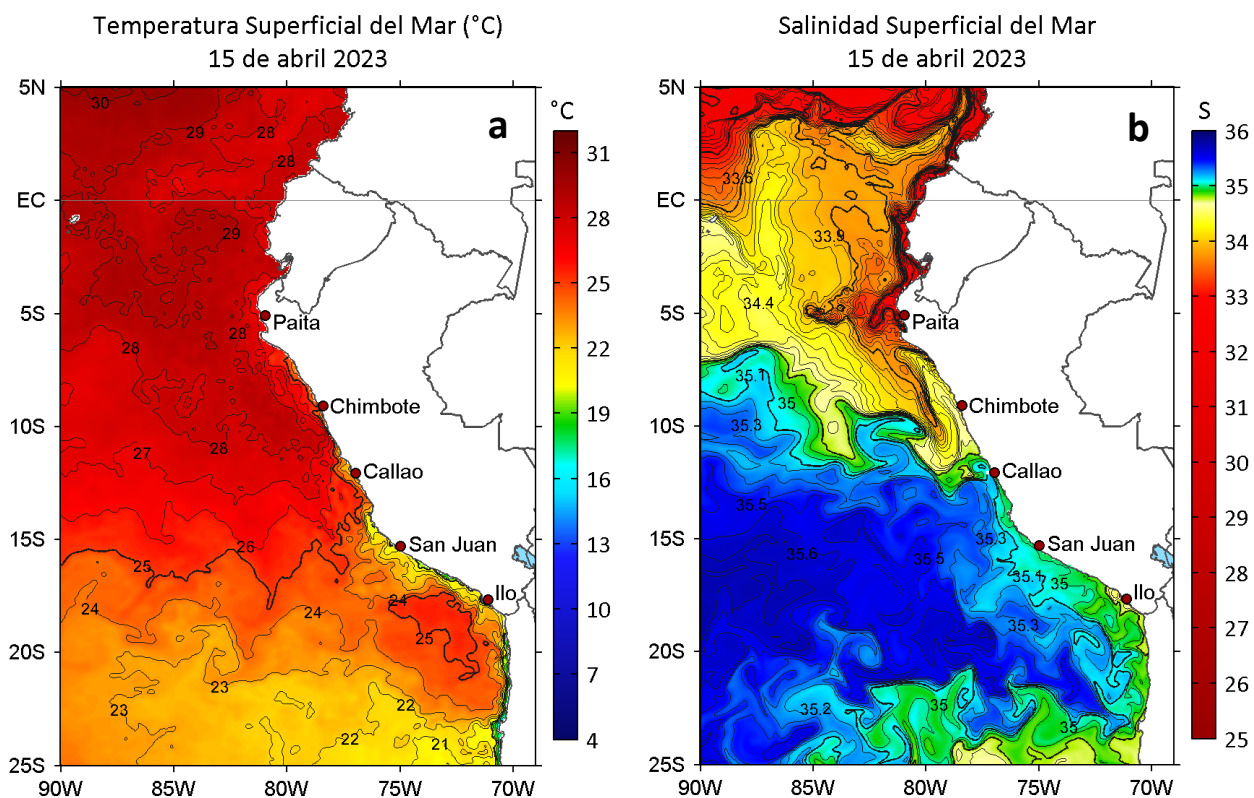
Figura 2. a) Temperatura superficial del mar ( ^{\circ}\text{C} ) y b) Salinidad superficial del mar para el 15 de abril de 2023. Datos: OSTIA-UKMO-L4-GLOB-v2.0 (UK Met Office, 2012; Donlon et al, 2012) y del GLOBAL_ANALYSIS_FORECAST_PHY_001_024 (Lellouche, J. M. et al, 2013), respectivamente.
