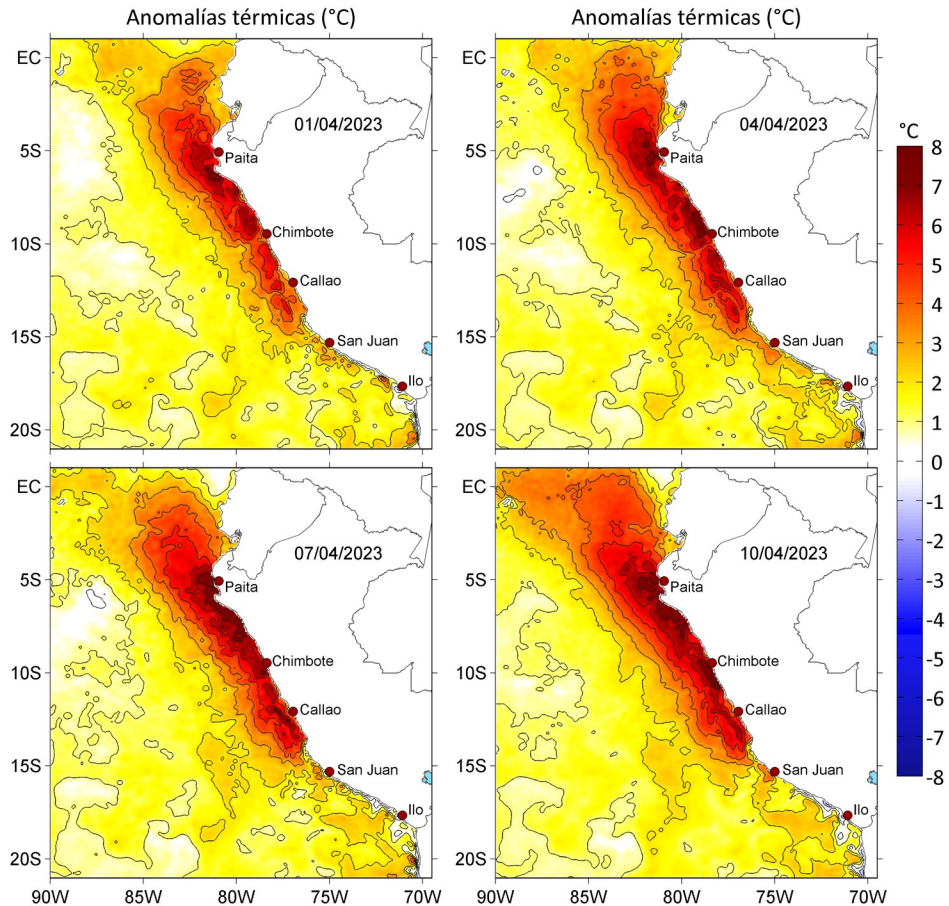
Figura 3. Anomalías de la temperatura superficial del mar ( ^{\circ}\text{C} ) para el a) 01, b) 04, c) 07 y d) 10 de abril de 2023. Las anomalías se calcularon respecto de la climatología para el periodo 2007-2016. Datos: OSTIA-UKMO-L4-GLOB-v2.0 (UK Met Office, 2012; Donlon et al, 2012).
