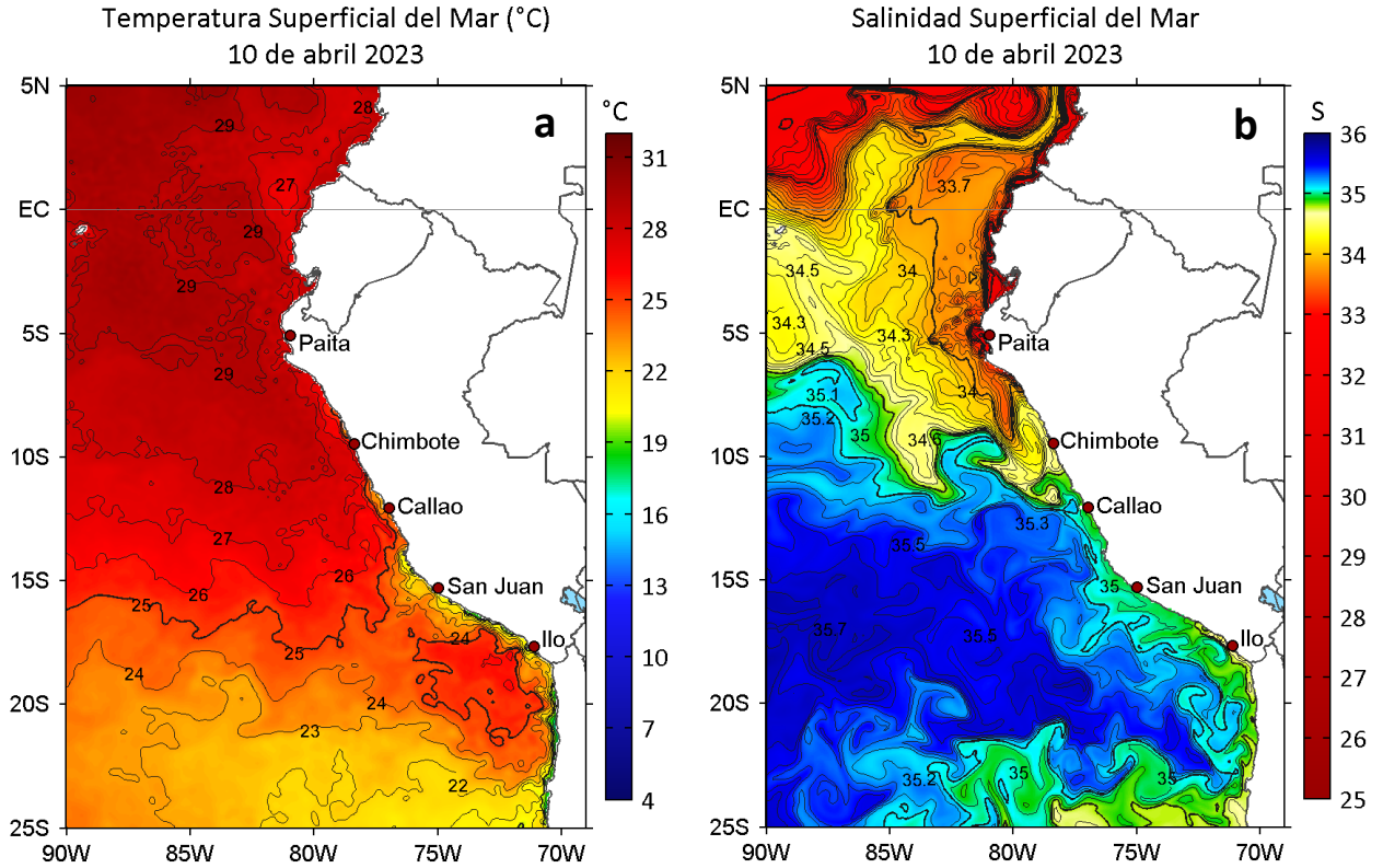
Figura 2. a) Temperatura superficial del mar ( ^{\circ}\text{C} ) y b) Salinidad superficial del mar para el 10 de abril de 2023. Datos: OSTIA-UKMO-L4-GLOB-v2.0 (UK Met Office, 2012; Donlon et al, 2012) y del GLOBAL_ANALYSIS_FORECAST_PHY_001_024 (Lellouche, J. M. et al, 2013), respectivamente.
