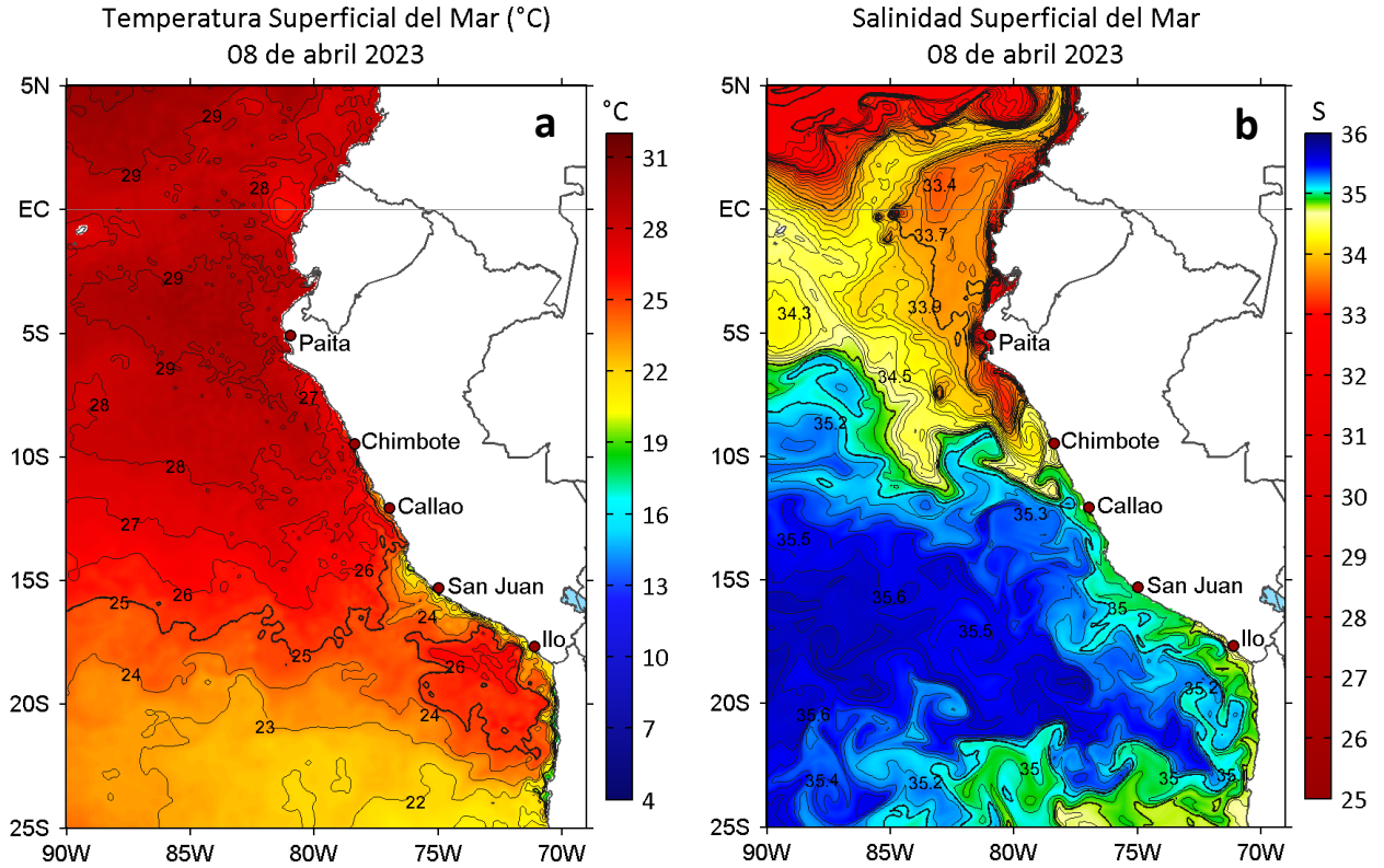
Figura 2. a) Temperatura superficial del mar ( ^{\circ}\text{C} ) y b) Salinidad superficial del mar para el 08 de abril de 2023. Datos: OSTIA-UKMO-L4-GLOB-v2.0 (UK Met Office, 2012; Donlon et al, 2012) y del GLOBAL_ANALYSIS_FORECAST_PHY_001_024 (Lellouche, J. M. et al, 2013), respectivamente.
