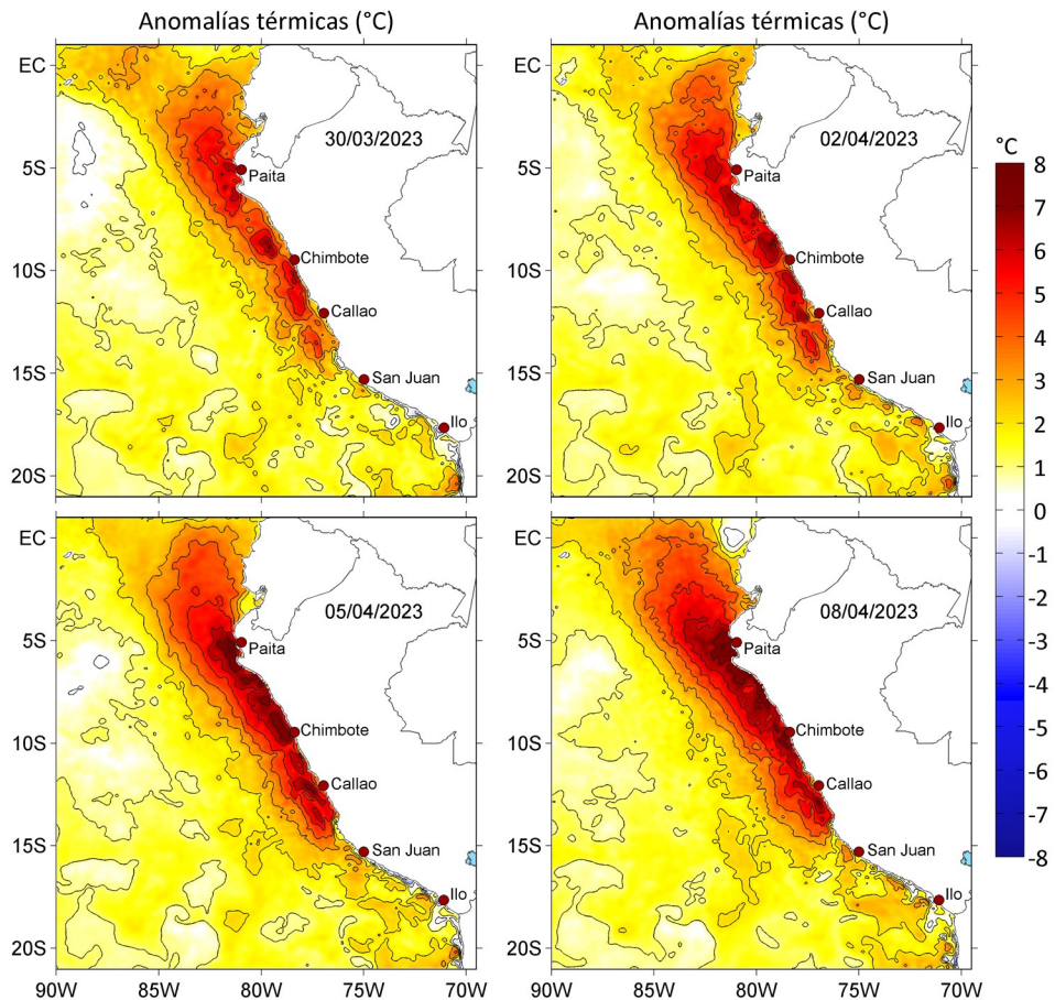
Figura 3. Anomalías de la temperatura superficial del mar ( ^{\circ}\text{C} ) para el a) 30 de marzo, b) 02, c) 05 y d) 08 de abril de 2023. Las anomalías se calcularon respecto de la climatología para el periodo 2007-2016. Datos: OSTIA-UKMO-L4-GLOB-v2.0 (UK Met Office, 2012; Donlon et al, 2012).
