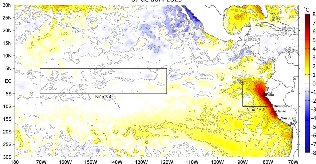
Figura 1. Anomalías de la temperatura superficial del mar ( ^{\circ}\text{C} ) en el océano Pacífico tropical. Las regiones Niño 3.4 ( 5^{\circ}\text{N}-5^{\circ}\text{S} , 170^{\circ}\text{W}-120^{\circ}\text{W} ) y Niño 1+2 ( 0^{\circ}-10^{\circ}\text{S} , 90^{\circ}\text{W}-80^{\circ}\text{W} ) están delimitadas con una línea de color negro. Las anomalías se estimaron de acuerdo a la climatología para el periodo 2007-2016. Los datos provienen de OSTIA-UKMO-L4-GLOB-v2.0 (UK Met Office, 2012; Donlon et al, 2012) disponibles en https://podaac.jpl.nasa.gov/dataset/OSTIA-UKMO-L4-GLOB-v2.0 .
