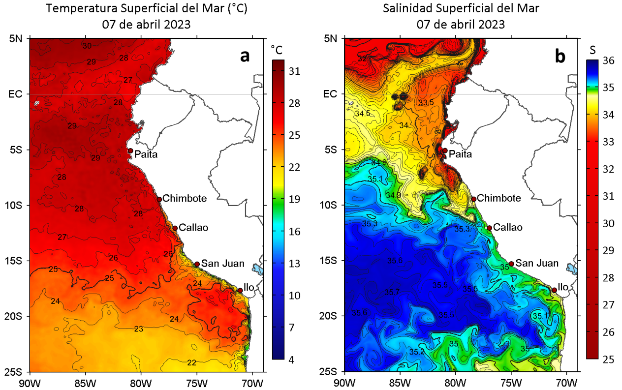
Figura 2. a) Temperatura superficial del mar ( ^{\circ}\text{C} ) y b) Salinidad superficial del mar para el 07 de abril de 2023. Datos: OSTIA-UKMO-L4-GLOB-v2.0 (UK Met Office, 2012; Donlon et al, 2012) y del GLOBAL_ANALYSIS_FORECAST_PHY_001_024 (Lellouche, J. M. et al, 2013), respectivamente.
