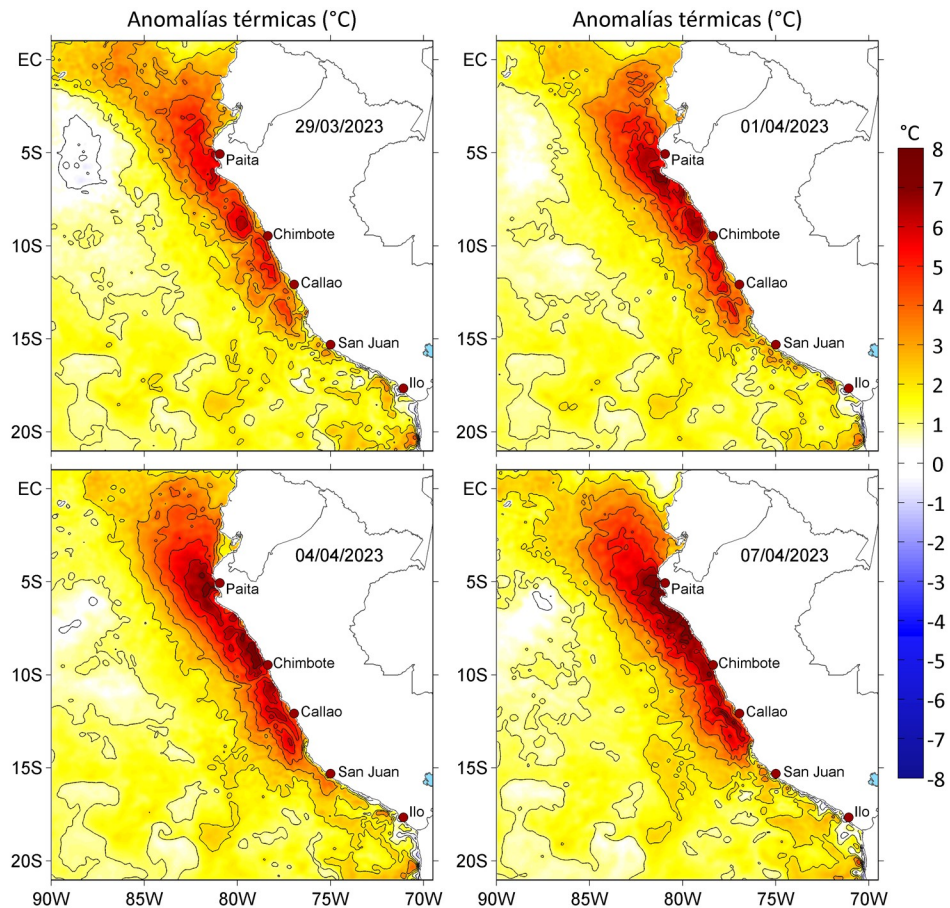
Figura 3. Anomalías de la temperatura superficial del mar ( ^{\circ}\text{C} ) para el a) 29 de marzo, b) 01, c) 04 y d) 07 de abril de 2023. Las anomalías se calcularon respecto de la climatología para el periodo 2007-2016. Datos: OSTIA-UKMO-L4-GLOB-v2.0 (UK Met Office, 2012; Donlon et al, 2012).
