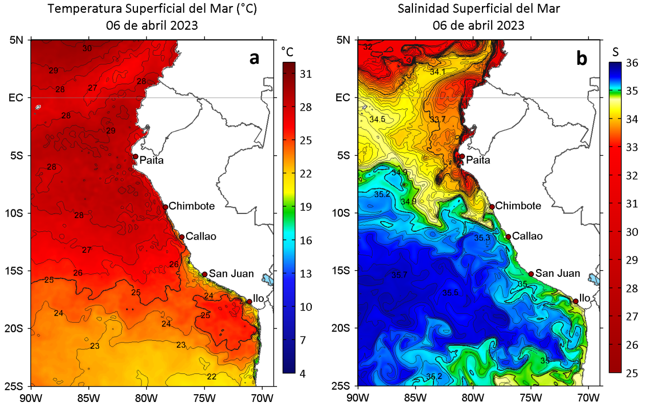
Figura 2. a) Temperatura superficial del mar ( ^{\circ}\text{C} ) y b) Salinidad superficial del mar para el 06 de abril de 2023. Datos: OSTIA-UKMO-L4-GLOB-v2.0 (UK Met Office, 2012; Donlon et al, 2012) y del GLOBAL_ANALYSIS_FORECAST_PHY_001_024 (Lellouche, J. M. et al, 2013), respectivamente.
