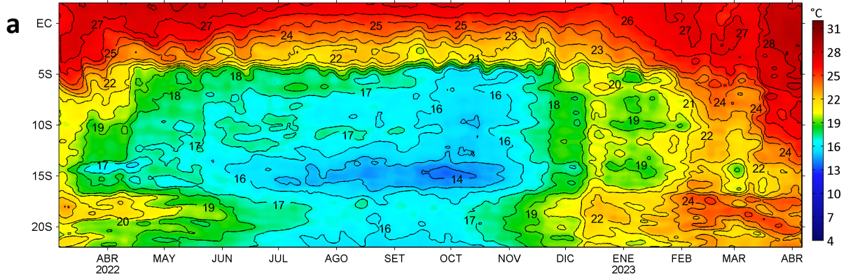
Anomalías de la Temperatura Superficial del mar (°C), franja costera de 60 m.n. 06 de marzo 2022 - 06 de abril 2023
