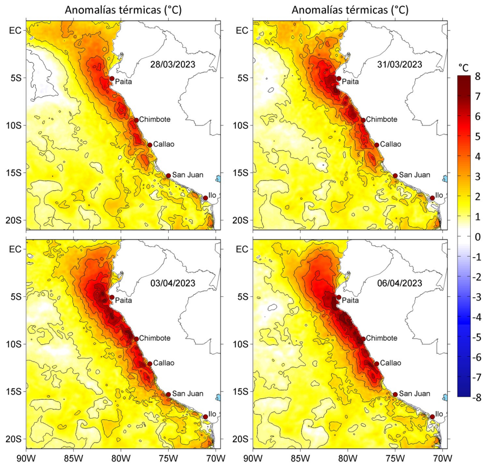
Figura 3. Anomalías de la temperatura superficial del mar ( ^{\circ}\text{C} ) para el a) 28 y b) 31 de marzo, así como para el c) 03 y d) 06 de abril de 2023. Las anomalías se calcularon respecto de la climatología para el periodo 2007-2016. Datos: OSTIA-UKMO-L4-GLOB-v2.0 (UK Met Office, 2012; Donlon et al, 2012).
