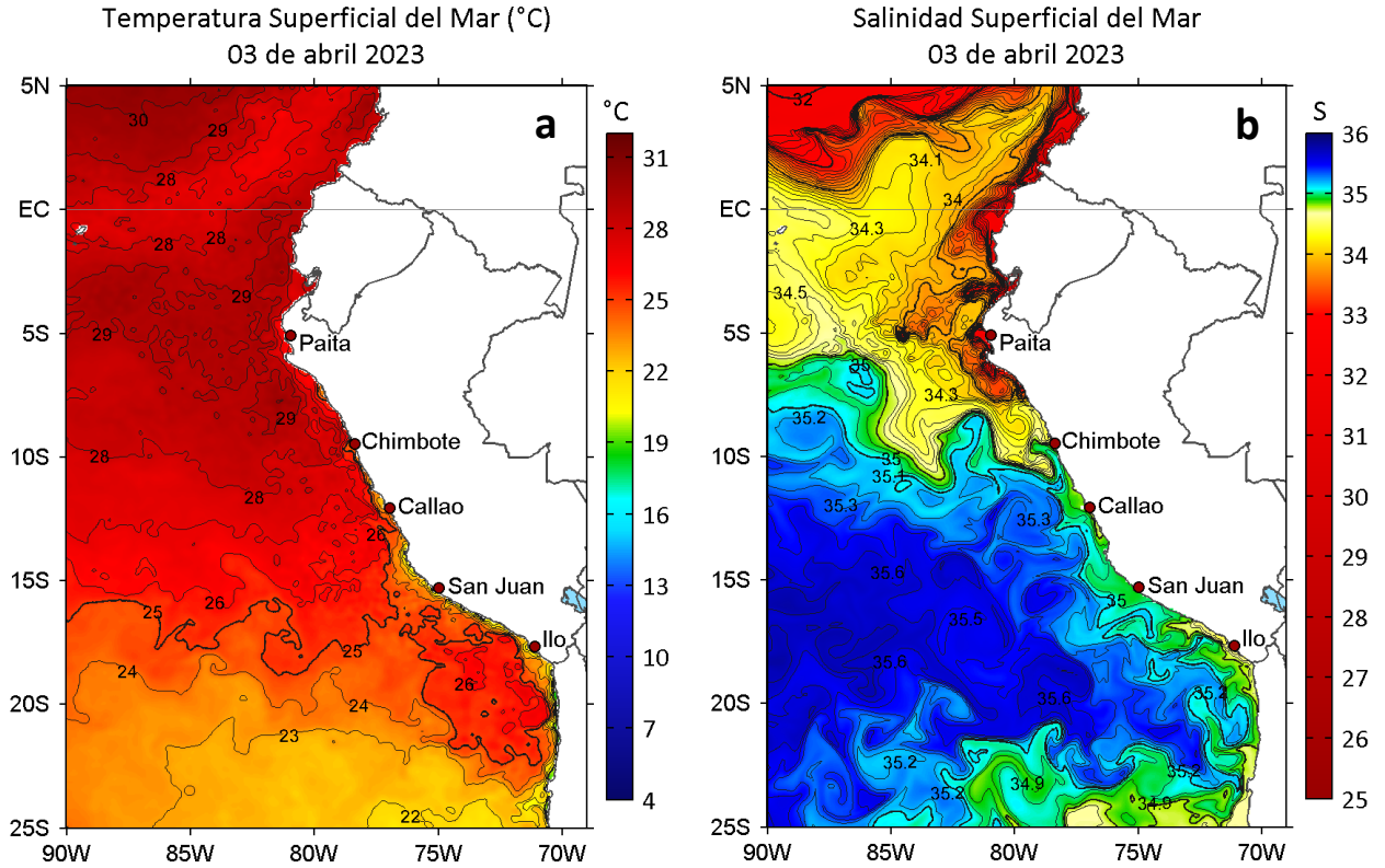
Figura 2. a) Temperatura superficial del mar ( ^{\circ}\text{C} ) y b) Salinidad superficial del mar para el 03 de abril de 2023. Datos: OSTIA-UKMO-L4-GLOB-v2.0 (UK Met Office, 2012; Donlon et al, 2012) y del GLOBAL_ANALYSIS_FORECAST_PHY_001_024 (Lellouche, J. M. et al, 2013), respectivamente.
