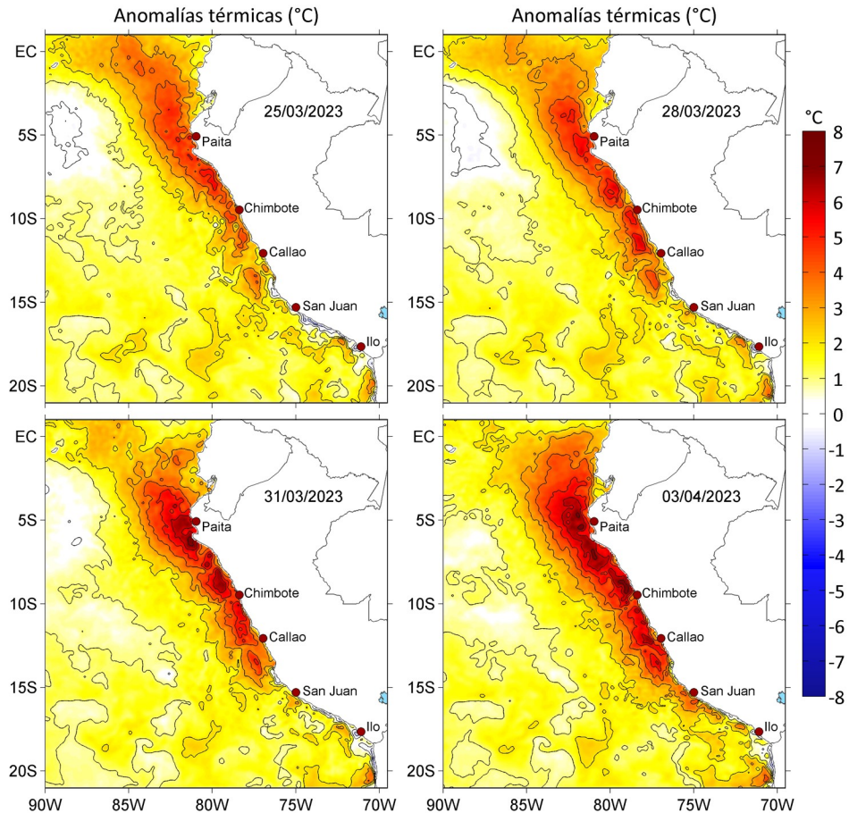
Figura 3. Anomalías de la temperatura superficial del mar ( ^{\circ}\text{C} ) para el a) 25, b) 28 y c) 31 de marzo, así como para el d) 03 de abril de 2023. Las anomalías se calcularon respecto de la climatología para el periodo 2007-2016. Datos: OSTIA-UKMO-L4-GLOB-v2.0 (UK Met Office, 2012; Donlon et al, 2012).
