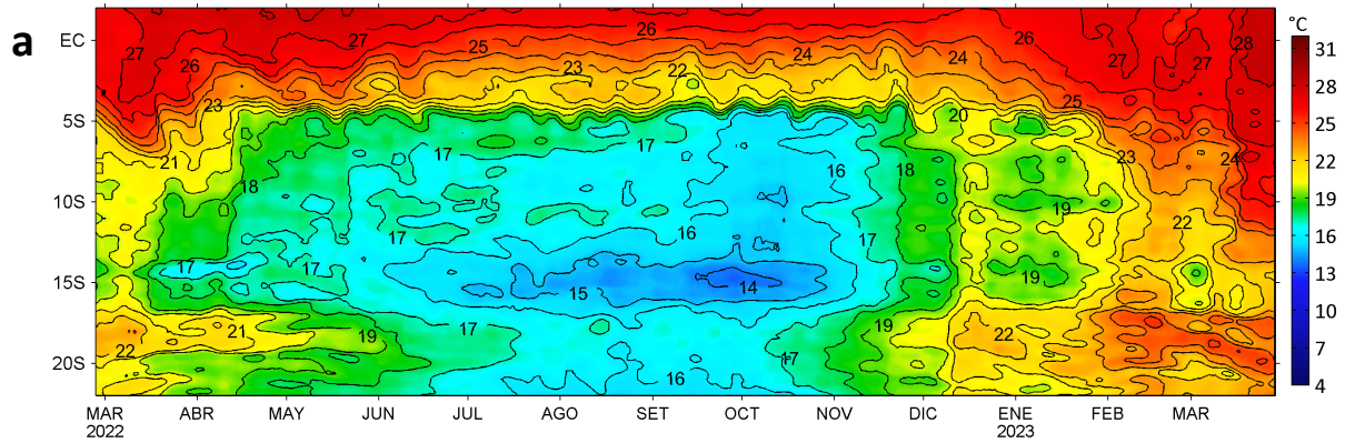
Anomalías de la Temperatura Superficial del mar (°C), franja costera de 60 m.n. 26 de febrero 2022 - 29 de marzo 2023
