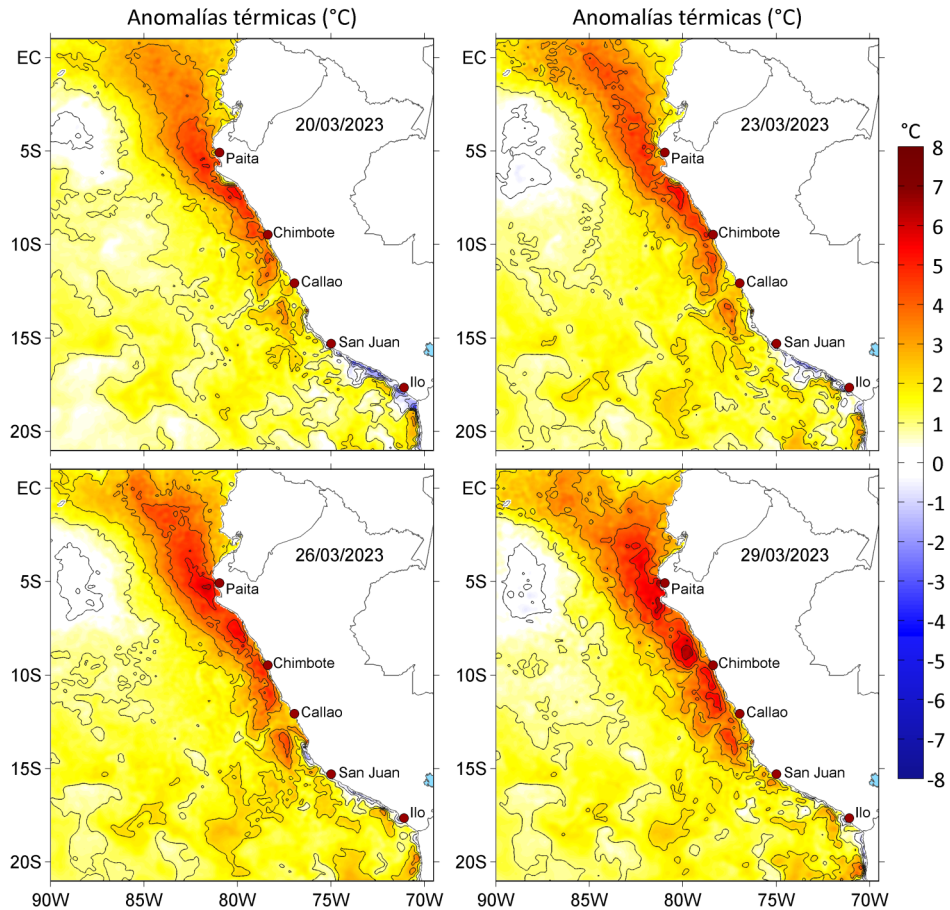
Figura 3. Anomalías de la temperatura superficial del mar ( ^{\circ}\text{C} ) para el a) 20, b) 23, c) 26 y d) 29 de marzo de 2023. Las anomalías se calcularon respecto de la climatología para el periodo 2007-2016. Datos: OSTIA-UKMO-L4-GLOB-v2.0 (UK Met Office, 2012; Donlon et al, 2012).
