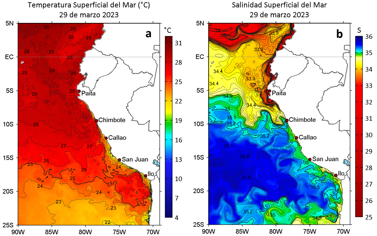
Figura 2. a) Temperatura superficial del mar ( ^{\circ}\text{C} ) y b) Salinidad superficial del mar para el 29 de marzo de 2023. Datos: OSTIA-UKMO-L4-GLOB-v2.0 (UK Met Office, 2012; Donlon et al, 2012) y del GLOBAL_ANALYSIS_FORECAST_PHY_001_024 (Lellouche, J. M. et al, 2013), respectivamente.
