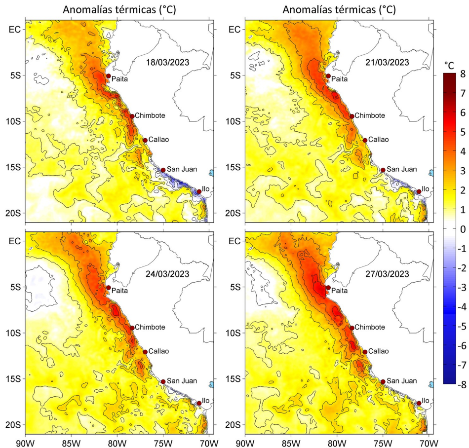
Figura 3. Anomalías de la temperatura superficial del mar ( ^{\circ}\text{C} ) para el a) 18, b) 21, c) 24 y d) 27 de marzo de 2023. Las anomalías se calcularon respecto de la climatología para el periodo 2007-2016. Datos: OSTIA-UKMO-L4-GLOB-v2.0 (UK Met Office, 2012; Donlon et al, 2012).
