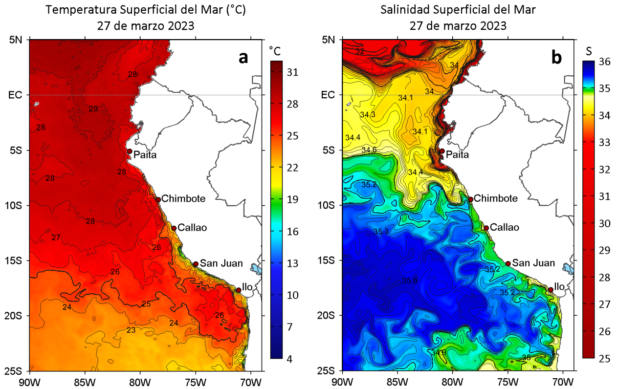
Figura 2. a) Temperatura superficial del mar ( ^{\circ}\text{C} ) y b) Salinidad superficial del mar para el 27 de marzo de 2023. Datos: OSTIA-UKMO-L4-GLOB-v2.0 (UK Met Office, 2012; Donlon et al, 2012) y del GLOBAL_ANALYSIS_FORECAST_PHY_001_024 (Lellouche, J. M. et al, 2013), respectivamente.
