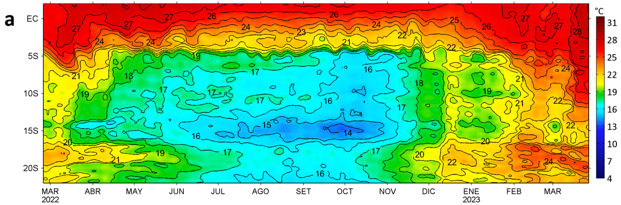
Anomalías de la Temperatura Superficial del mar (°C), franja costera de 60 m.n. 24 de febrero 2022 - 27 de marzo 2023
