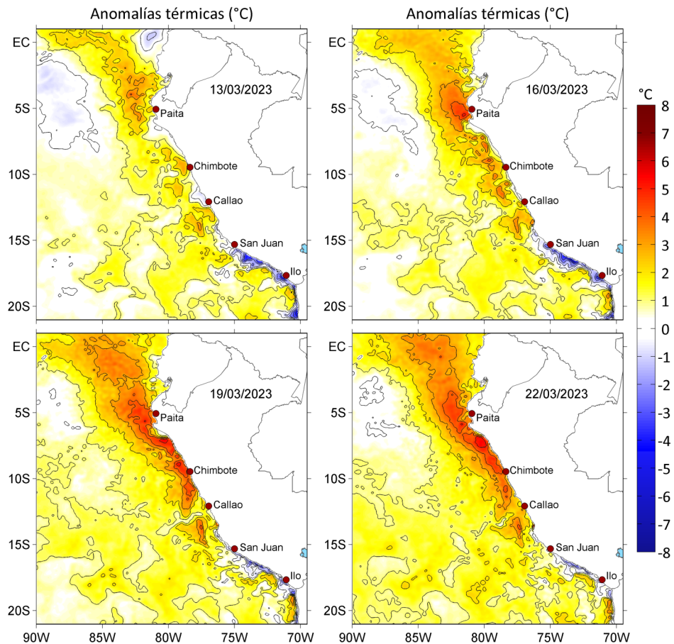
Figura 3. Anomalías de la temperatura superficial del mar ( ^{\circ}\text{C} ) para el a) 13, b) 16, c) 19 y d) 22 de marzo de 2023. Las anomalías se calcularon respecto de la climatología para el periodo 2007-2016. Datos: OSTIA-UKMO-L4-GLOB-v2.0 (UK Met Office, 2012; Donlon et al, 2012).
