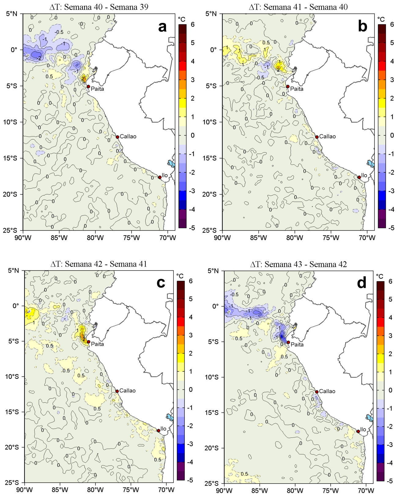
Figura 3. Variación semanal de la temperatura superficial del mar (°C) en el océano Pacífico tropical oriental entre: a) cuadragésima (30 de setiembre - 06 de octubre) y trigésima novena (23-29 de setiembre) semana del 2020, b) cuadragésima primera (07-13 de octubre) y cuadragésima (30 de setiembre - 06 de octubre) semana del 2020, c) cuadragésima segunda (14-20 de octubre) y cuadragésima primera (07-13 de octubre) semana del 2020 y d) cuadragésima tercera (21-27 de octubre) y cuadragésima segunda (14-20 de octubre) semana del 2020. Los mapas, que indican el grado de calentamiento o enfriamiento de una semana a otra, provienen de OSTIA-UKMO-L4-GLOB-v2.0 (UK Met Office, 2012; Donlon et al, 2012). La barra de colores a la derecha muestra la diferencia de la temperatura entre la presente y la semana previa. Procesamiento: LHF/AFIOF/DGIOCC/IMARPE.
