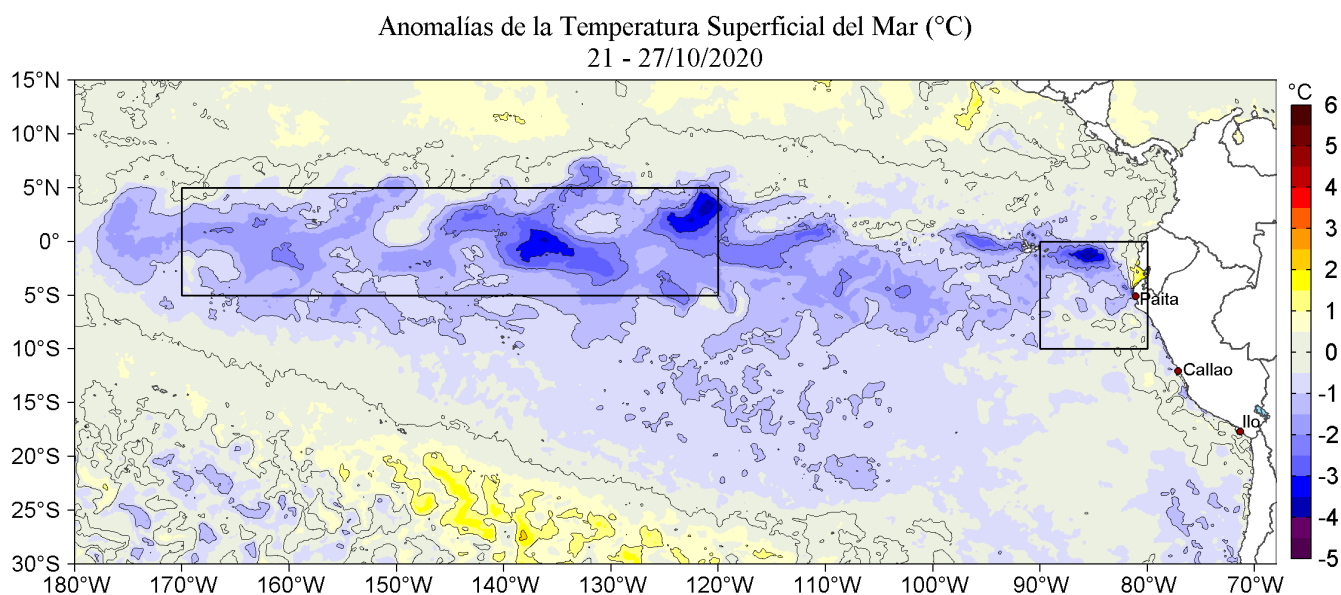
Figura 2. Anomalías promedio de la Temperatura superficial del mar (°C) en el océano Pacífico tropical para la semana del 21 al 27 de octubre de 2020. Las regiones Niño 3.4 y Niño 1+2 en los sectores central y oriental del océano, respectivamente están delimitadas con una línea de color gris. Datos: OSTIA-UKMO-L4-GLOB-v2.0 (UK Met Office, 2012; Donlon et al, 2012) disponible en https://podaac.jpl.nasa.gov/dataset/OSTIA-UKMO-L4-GLOB-v2.0 . Las anomalías se calcularon con respecto de la climatología para el período 2007-2016. Procesamiento: LHF/AFIOF/DGIOCC/IMARPE.
