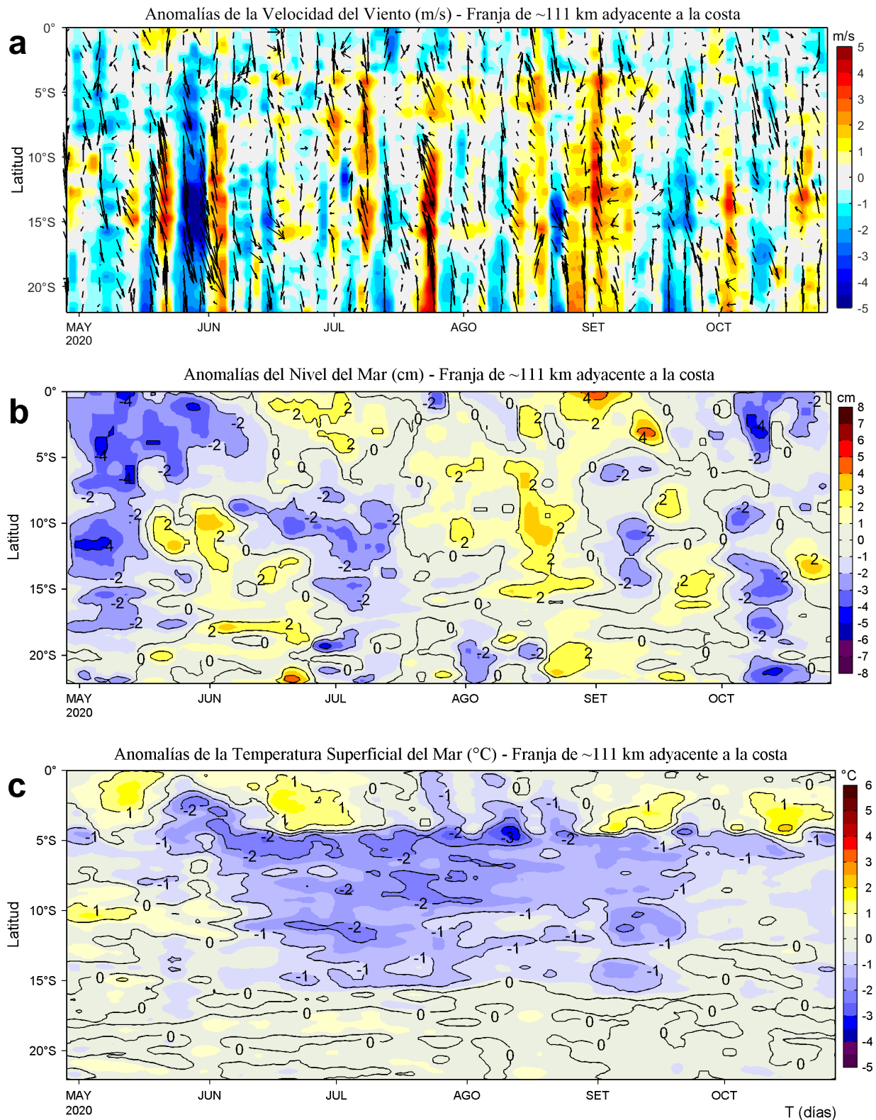
Figura 4. Evolución de las anomalías diarias de: a) Velocidad del viento (m/s), b) Nivel del mar (cm), c) Temperatura superficial del mar (°C) para el último semestre, actualizado al 27 de octubre de 2020. Los datos de anomalías de nivel del mar consideran un filtro pasa alto de 120 días. Datos: de IFREMER/CERSAT para (a), del Servicio de Monitoreo del Ambiente Marino Copernicus (CMEMS en inglés) para (b), de OSTIA-UKMO-L4-GLOB-v2.0 para (c). Las anomalías fueron calculadas para una franja de 111 km adyacente a la costa entre el ecuador geográfico y 22°S según los promedios climatológicos diarios de 2000-2014 para (a), de 1993-2010 para (b) y de 2007-2016 para (c). La barra de colores a la derecha muestra la escala de las anomalías en cada caso. Procesamiento: LHF/AFIOF/DGIOCC/IMARPE.
