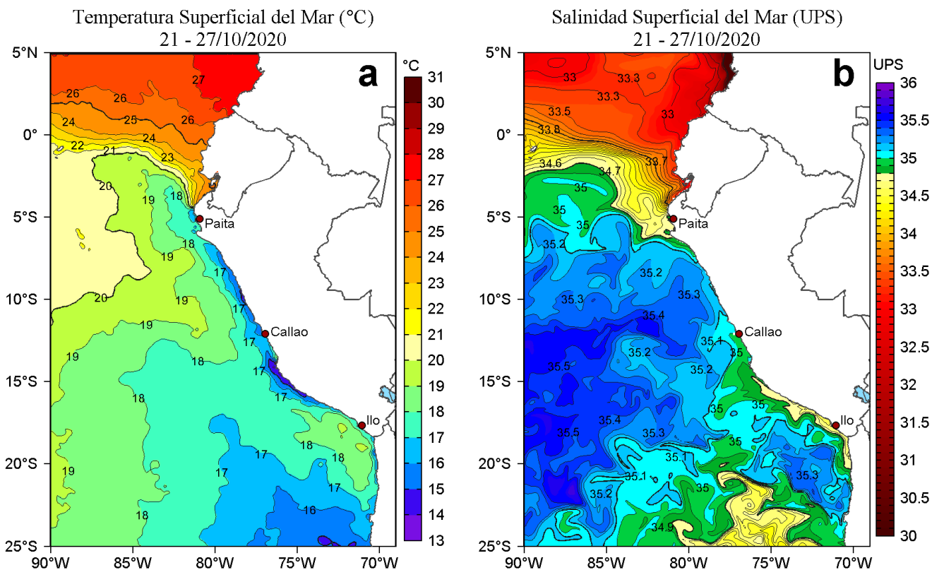
Figura 1. Distribución espacial promedio de: a) Temperatura superficial del mar (TSM, °C) y b) Salinidad superficial del mar (SSM, ups) para la semana del 21 al 27 de octubre de 2020 en el océano Pacífico tropical oriental. Datos: OSTIA-UKMO-L4-GLOB-v2.0 (UK Met Office, 2012; Donlon et al, 2012) disponible en https://podaac.jpl.nasa.gov/dataset/OSTIA-UKMO-L4-GLOB-v2.0 para (a) y del GLOBAL_ANALYSIS_FORECAST_PHY_001_024 (Lellouche, J.-M. et al, 2013) disponible en http://marine.copernicus.eu/services-portfolio/access-to-products/?option=com_csw&view=details&product_id=GLOBAL_ANALYSIS_FORECAST_PHY_001_024 para (b). Las escalas de colores de la TSM como de la SSM se presentan a la derecha de cada gráfico. Procesamiento: LHF/AFIOF/DGIOCC/IMARPE.
