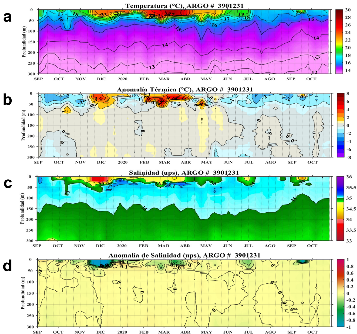
Figura 5. Diagrama Hovmöller de: a) Temperatura del mar (°C), b) Anomalías térmicas (°C), c) Salinidad del agua de mar (ups) y d) Anomalía de la salinidad del mar (ups) a 58 m.n. frente a Punta Falsa (81,99°W y 5,99°S) de setiembre del 2019 al 25 de octubre de 2020. Las anomalías de la temperatura del agua (°C) y de salinidad (ups) se calcularon de acuerdo a Domínguez et al (2017). Los puntos en la columna de agua indican los días en que el perfilador ARGO registró información. Datos: ARGO. Procesamiento: LHQM/AFIOQ/DGIOCC/IMARPE.
