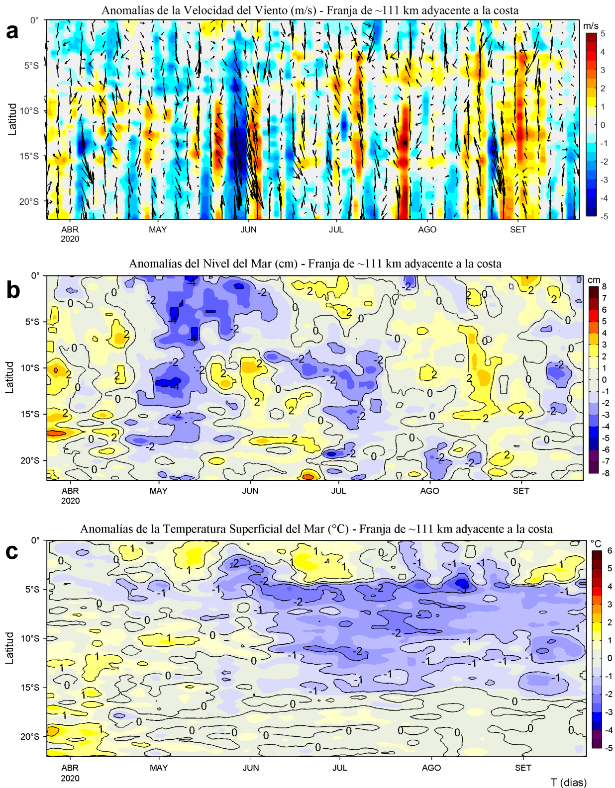
Figura 4. Evolución de las anomalías diarias de: a) Velocidad del viento (m/s), b) Nivel del mar (cm), c) Temperatura superficial del mar (°C) para el último semestre, actualizado al 22 de setiembre de 2020. Los datos de anomalías de nivel del mar consideran un filtro pasa alto de 120 días. Datos: de IFREMER/CERSAT para (a), del Servicio de Monitoreo del Ambiente Marino Copernicus (CMEMS en inglés) para (b), de OSTIA-UKMO-L4-GLOB-v2.0 para (c). Las anomalías fueron calculadas para una franja de 111 km adyacente a la costa entre el ecuador y 22°S según los promedios climatológicos diarios de 2000-2014 para (a), de 1993-2010 para (b) y de 2007-2016 para (c). La barra de colores a la derecha muestra la escala de las anomalías en cada caso. Procesamiento: LHF/AFIOF/DGIOCC/IMARPE.
