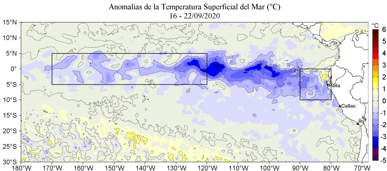
Figura 2. Anomalías promedio de la Temperatura superficial del mar (°C) en el océano Pacífico tropical para la semana del 16 al 22 de setiembre de 2020. Las regiones Niño 3.4 y Niño 1+2 en los sectores central y oriental del océano, respectivamente están delimitadas con una línea de color gris. Datos: OSTIA-UKMO-L4-GLOB-v2.0 (UK Met Office, 2012; Donlon et al, 2012) disponible en https://podaac.jpl.nasa.gov/dataset/OSTIA-UKMO-L4-GLOB-v2.0 . Las anomalías se calcularon con respecto de la climatología para el período 2007-2016. Procesamiento: LHF/AFIOF/DGIOCC/IMARPE.
