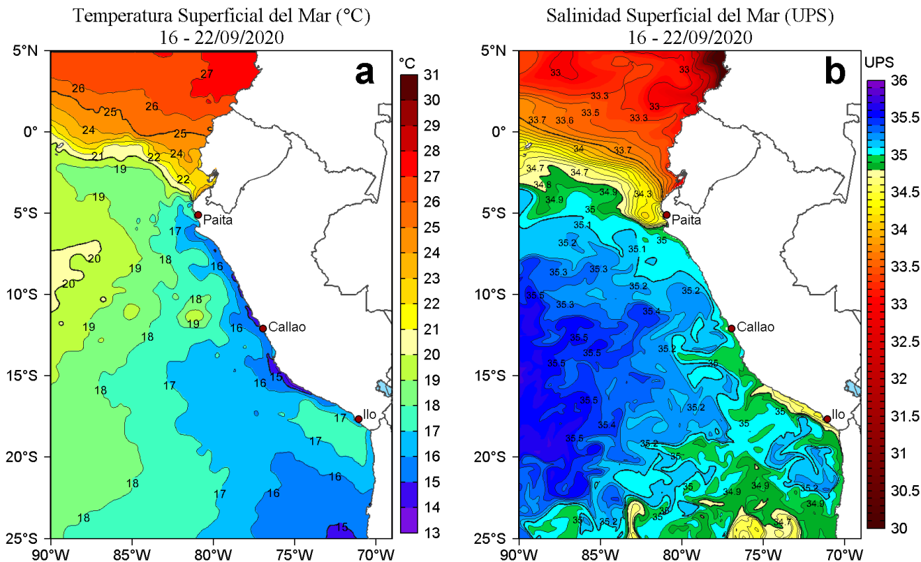
Figura 1. Distribución espacial promedio de: a) Temperatura superficial del mar (TSM, °C) y b) Salinidad superficial del mar (SSM, ups) para la semana del 16 al 22 de setiembre de 2020 en el océano Pacífico tropical oriental. Datos: OSTIA-UKMO-L4-GLOB-v2.0 (UK Met Office, 2012; Donlon et al, 2012) disponible en https://podaac.jpl.nasa.gov/dataset/OSTIA-UKMO-L4-GLOB-v2.0 para (a) y del GLOBAL_ANALYSIS_FORECAST_PHY_001_024 (Lellouche, J.-M. et al, 2013) disponible en http://marine.copernicus.eu/services-portfolio/access-to-products/?option=com_csw&view=details&product_id=GLOBAL_ANALYSIS_FORECAST_PHY_001_024 para (b). Las escalas de colores de la TSM como de la SSM se presentan a la derecha de cada gráfico. Procesamiento: LHF/AFIOF/DGIOCC/IMARPE.
