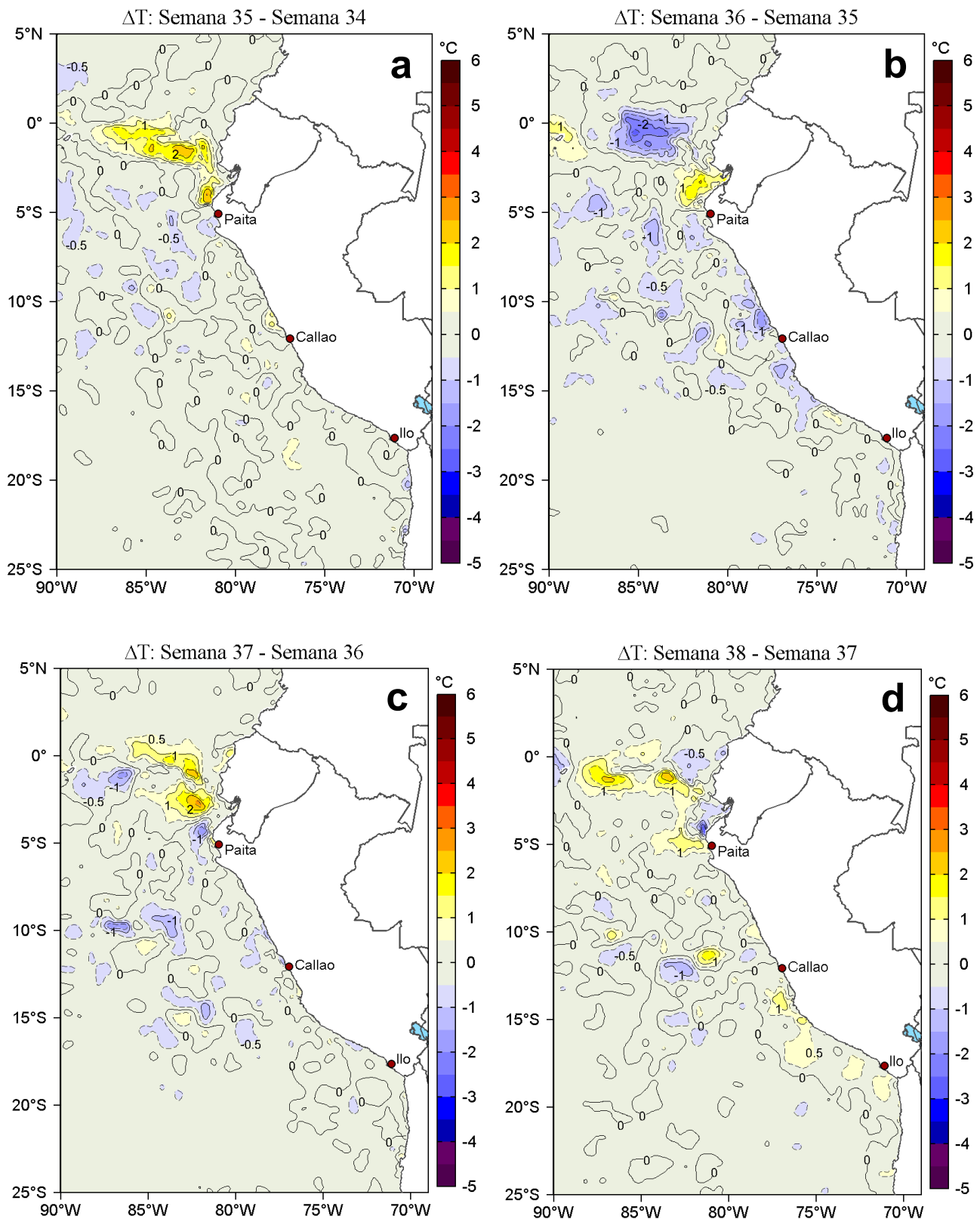
Figura 3. Variación semanal de la temperatura superficial del mar (°C) en el océano Pacífico tropical oriental entre: a) trigésima quinta (26 de agosto - 01 de setiembre) y trigésima cuarta (19-25 de agosto) semana del 2020, b) trigésima sexta (02-08 de setiembre) y trigésima quinta (26 de agosto - 01 de setiembre) semana del 2020, c) trigésima séptima (09-15 de setiembre) y trigésima sexta (02-08 de setiembre) semana del 2020 y d) trigésima octava (16-22 de setiembre) y trigésima séptima (09-15 de setiembre) semana del 2020. Los mapas, que indican el grado de calentamiento o enfriamiento de una semana a otra, provienen de OSTIA-UKMO-L4-GLOB-v2.0 (UK Met Office, 2012; Donlon et al, 2012). La barra de colores a la derecha muestra la diferencia de la temperatura entre la presente y la semana previa. Procesamiento: LHF/AFIOF/DGIOCC/IMARPE.
