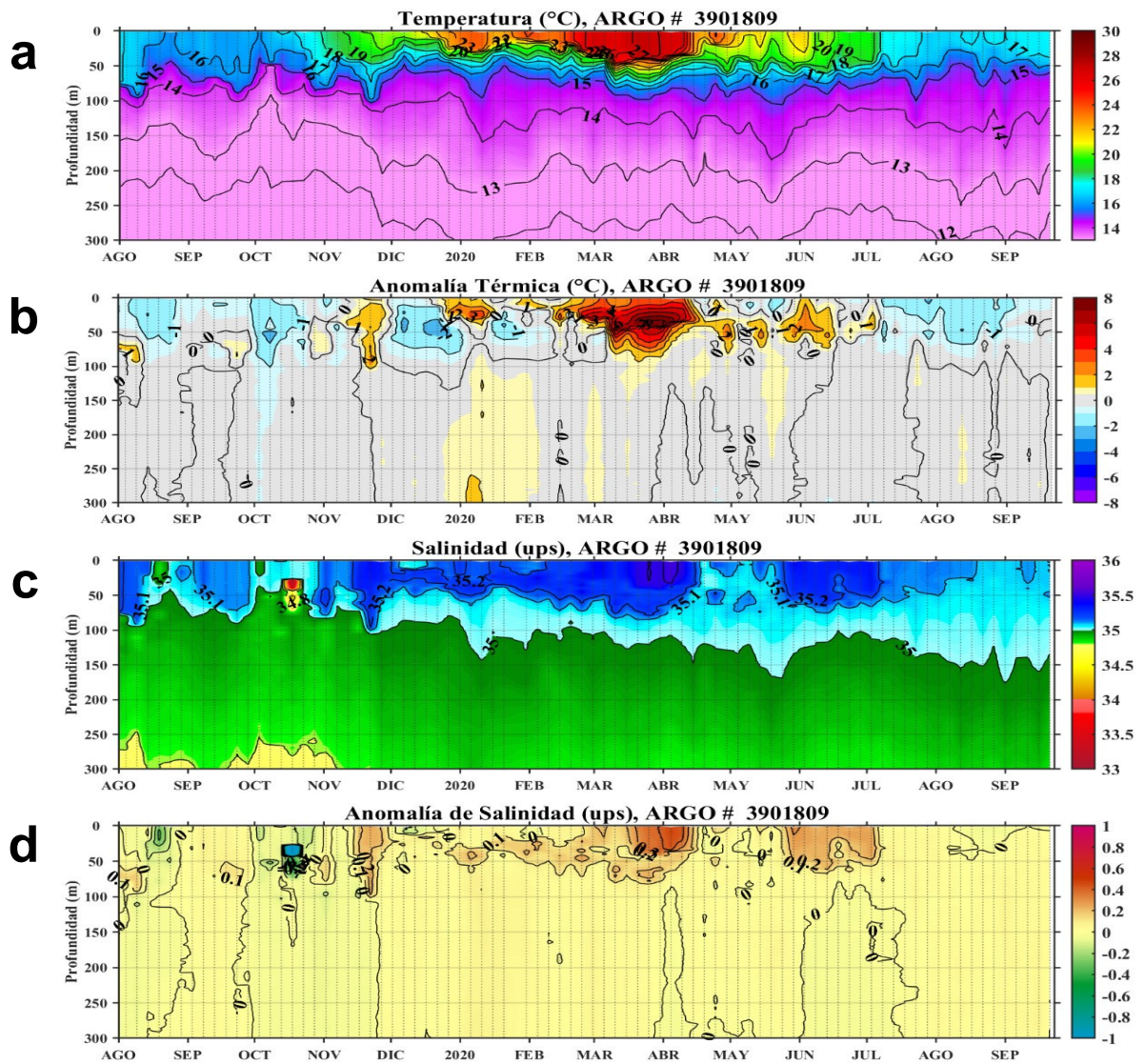
Figura 5. Diagrama Hovmöller de: a) Temperatura del mar (°C), b) Anomalías térmicas (°C), c) Salinidad del agua de mar (ups) y d) Anomalía de la salinidad del mar (ups) a 98,44 m.n. frente a Chicama (~80,93°W y ~8,01°S) de agosto del 2019 al 20 de setiembre de 2020. Las anomalías de la temperatura del agua (°C) y de salinidad (ups) se calcularon de acuerdo a Domínguez et al (2017). Los puntos en la columna de agua indican los días en que el perfilador ARGO registró información. Datos: ARGO. Procesamiento: LHQM/AFIOQ/DGIOCC/IMARPE.
