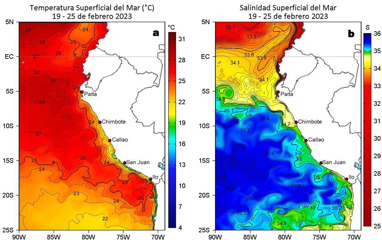
Figura 2. Distribución espacial promedio de: a) TSM (°C) y b) Salinidad superficial del mar (SSM) para la semana del 19 al 25 de febrero 2023. Datos: OSTIA-UKMO-L4-GLOB-v2.0 (UK Met Office, 2012; Donlon et al, 2012) disponible en https://podaac.jpl.nasa.gov/dataset/OSTIA-UKMO-L4-GLOB-v2.0 para (a) y del GLOBAL_ANALYSIS_FORECAST_PHY_001_024 (Lellouche, J. M. et al, 2013) disponible en http://marine.copernicus.eu/services-portfolio/access-to-products/?option=com_csw&view=details&product_id=GLOBAL_ANALYSIS_FORECAST_PHY_001_024 para (b). Las escalas de colores se presentan a la derecha de cada gráfico.
