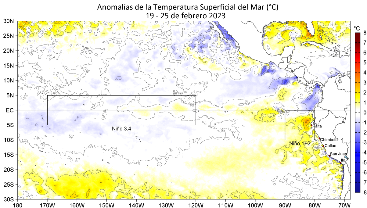
Figura 1. Anomalías promedio de la Temperatura superficial del mar (TSM, °C) en el océano Pacífico tropical para la semana del 19 al 25 de febrero 2023. Las regiones Niño 3.4 y Niño 1+2 en los sectores central y oriental del océano, respectivamente, están delimitadas con una línea de color gris. Datos: OSTIA-UKMO-L4-GLOB-v2.0 (UK Met Office, 2012; Donlon et al, 2012) disponible en https://podaac.jpl.nasa.gov/dataset/OSTIA-UKMO-L4-GLOB-v2.0 . Las anomalías se calcularon con respecto de la climatología para el periodo 2007-2016.
