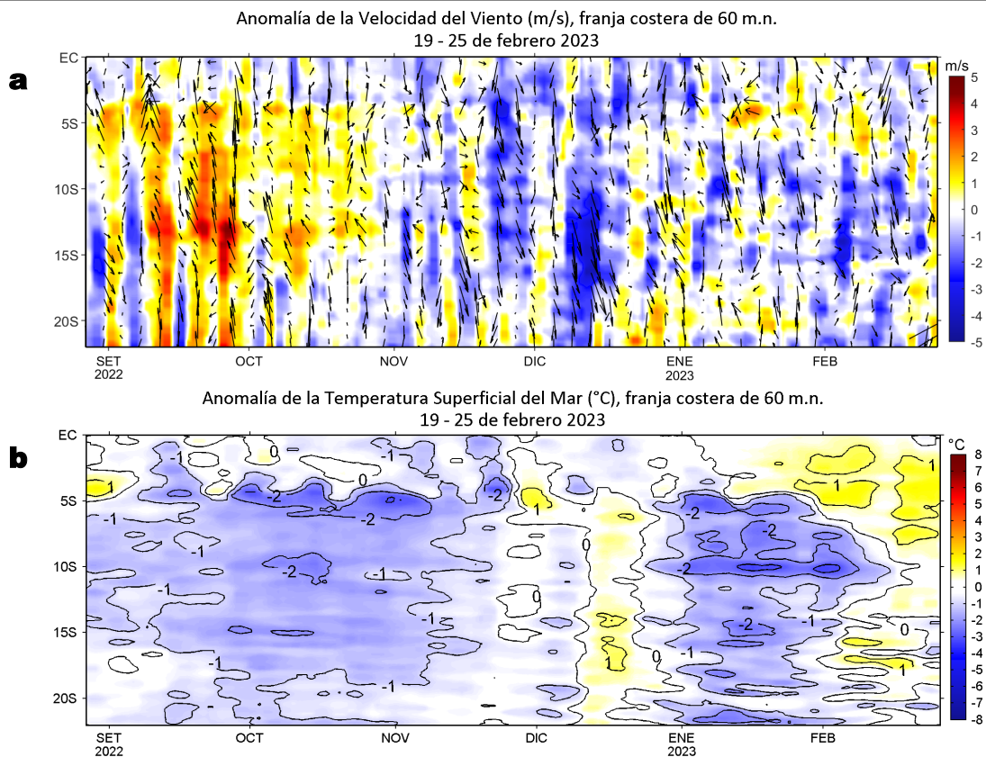
Figura 4. Evolución de las anomalías diarias de: a) Velocidad del viento (m/s) y b) Temperatura superficial del mar (°C) para el último semestre, actualizado al 25 de febrero de 2023. Datos: de IFREMER/CERSAT para (a) y de OSTIA-UKMO-L4-GLOB-v2.0 para (b). Las anomalías fueron calculadas para una franja de 60 m.n. adyacente a la costa entre el ecuador geográfico y 22°S según los promedios climatológicos diarios de 2000-2014 para (a) y de 2007-2016 para (b). La barra de colores a la derecha muestra la escala de las anomalías en cada caso.
