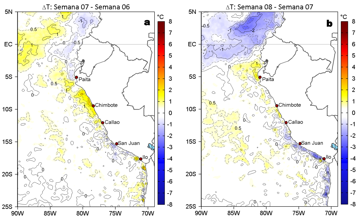
Figura 3. Variación semanal de la TSM (°C) en el océano Pacífico tropical oriental entre: a) séptima (12-18 de febrero) y sexta (05-11 de febrero) semana de 2023 y b) octava (19-25 de febrero) y séptima (12-18 de febrero) semana de 2023. Los mapas, que indican el grado de calentamiento o enfriamiento de una semana a otra, provienen de OSTIA-UKMO-L4-GLOB-v2.0 (UK Met Office, 2012; Donlon et al, 2012). La barra de colores a la derecha muestra la diferencia de la temperatura entre la presente y la semana previa.
