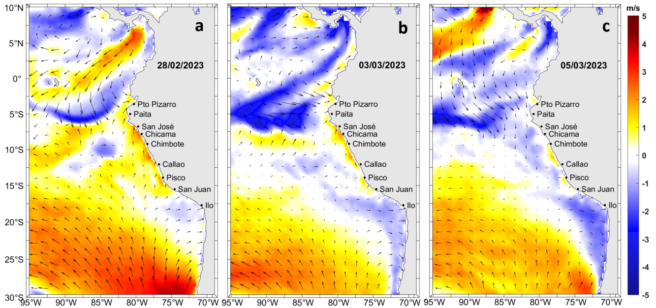
Figura 9. Distribución espacial del pronóstico de las anomalías de la velocidad del viento (m/s) y dirección del viento (°) para el a) 28 de febrero, b) 03 y c) 05 de marzo de 2023, frente a la costa entre Panamá y Chile. Fuente: Modelo Climate Forecast System (GFS) de la NOAA.
