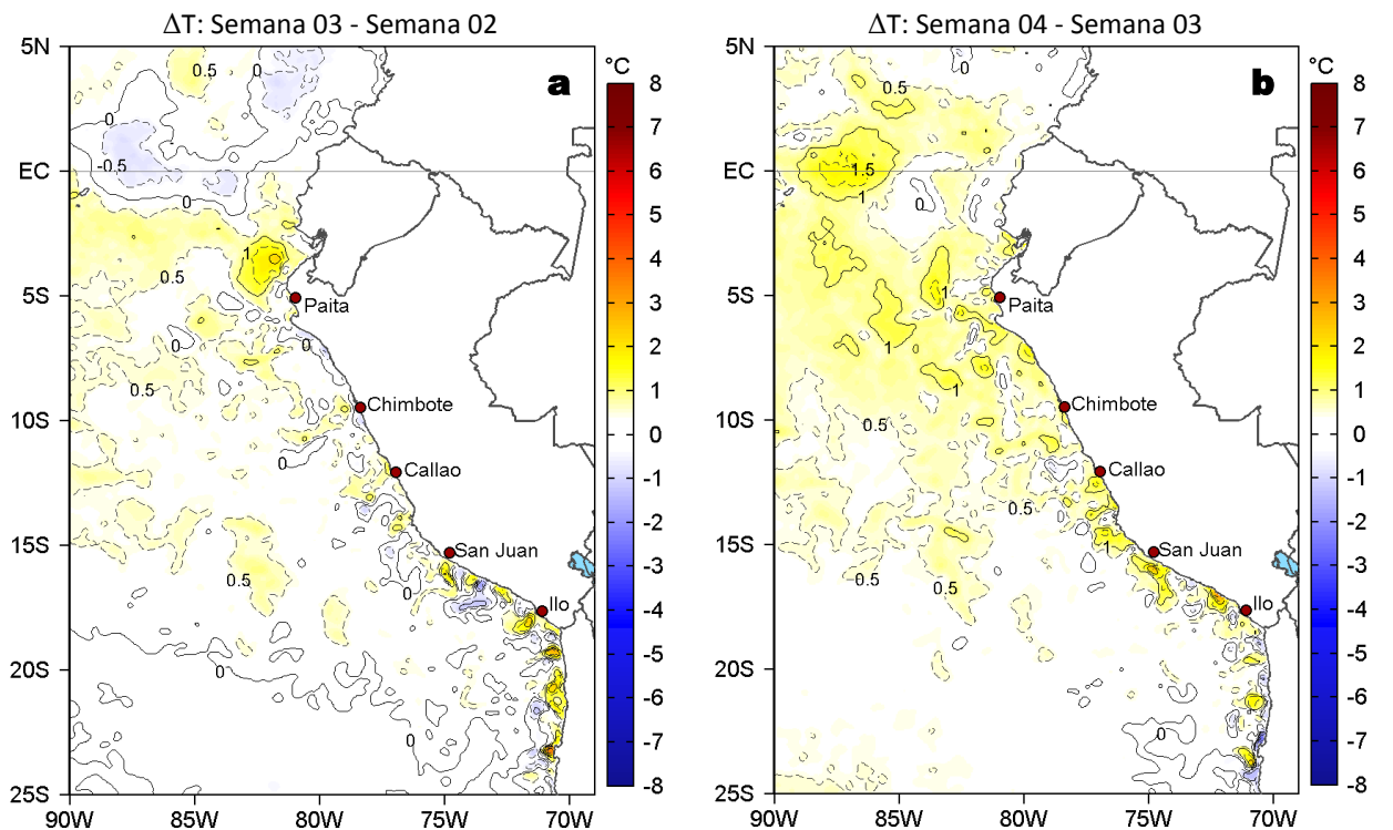
Figura 3. Variación semanal de la TSM (°C) en el océano Pacífico tropical oriental entre: a) tercera (15-21 de enero) y segunda (08-14 de enero) semana de 2023 y b) cuarta (22-28 de enero) y tercera (15-21 de enero) semana de 2023. Los mapas, que indican el grado de calentamiento o enfriamiento de una semana a otra, provienen de OSTIA-UKMO-L4-GLOB-v2.0 (UK Met Office, 2012; Donlon et al, 2012). La barra de colores a la derecha muestra la diferencia de la temperatura entre la presente y la semana previa.
