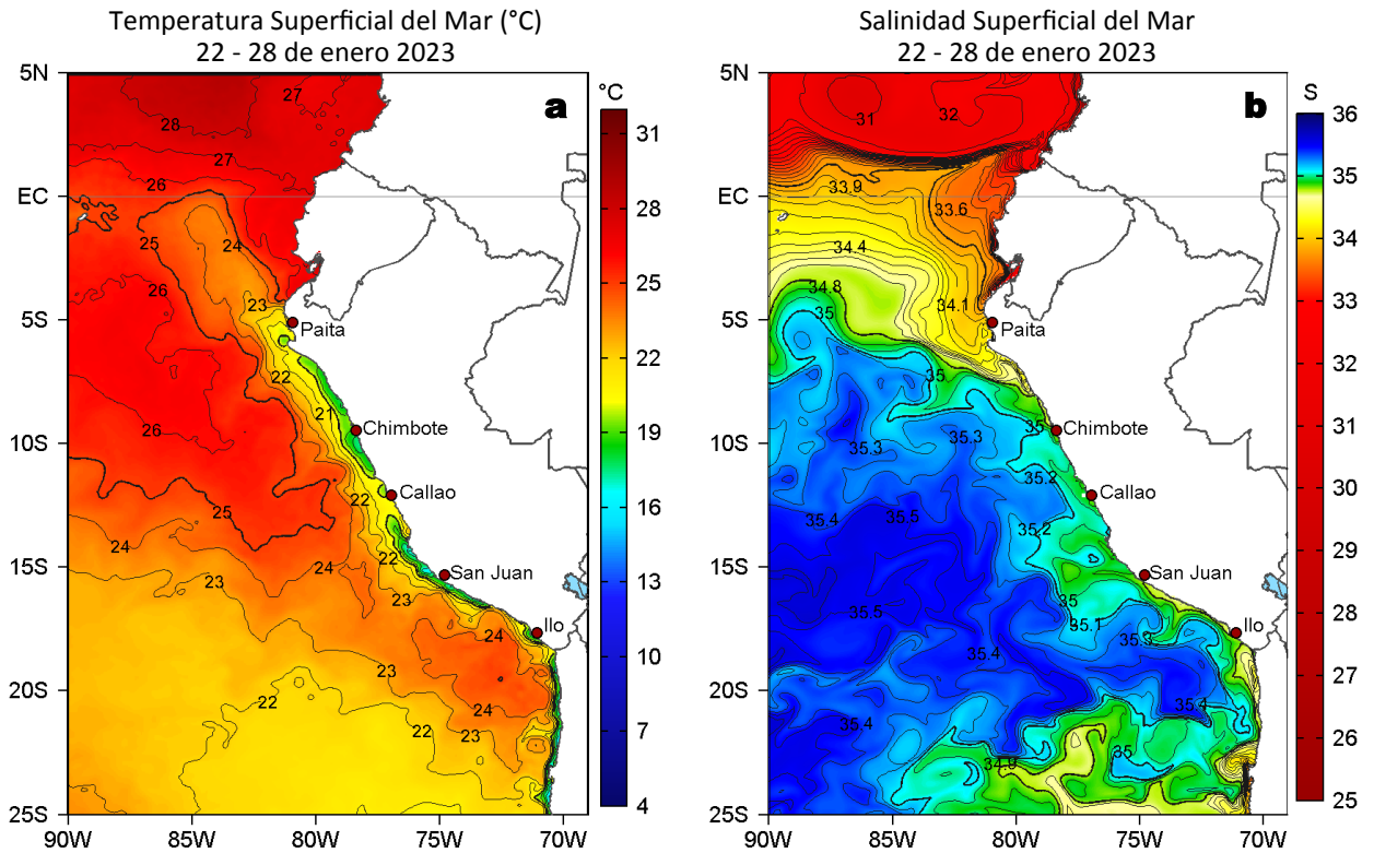
Figura 2. Distribución espacial promedio de: a) TSM (°C) y b) Salinidad superficial del mar (SSM) para la semana del 22 al 28 de enero 2023. Datos: OSTIA-UKMO-L4-GLOB-v2.0 (UK Met Office, 2012; Donlon et al, 2012) disponible en https://podaac.jpl.nasa.gov/dataset/OSTIA-UKMO-L4-GLOB-v2.0 para (a) y del GLOBAL_ANALYSIS_FORECAST_PHY_001_024 (Lellouche, J. M. et al, 2013) disponible en http://marine.copernicus.eu/services-portfolio/access-to-products/?option=com_csw&view=details&product_id=GLOBAL_ANALYSIS_FORECAST_PHY_001_024 para (b). Las escalas de colores se presentan a la derecha de cada gráfico.
