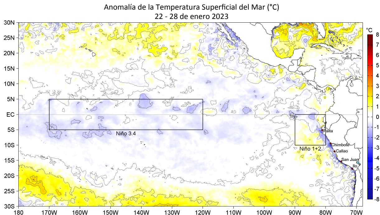
Figura 1. Anomalías promedio de la Temperatura superficial del mar (TSM, °C) en el océano Pacífico tropical para la semana del 22 al 28 de enero 2023. Las regiones Niño 3.4 y Niño 1+2 en los sectores central y oriental del océano, respectivamente, están delimitadas con una línea de color gris. Datos: OSTIA-UKMO-L4-GLOB-v2.0 (UK Met Office, 2012; Donlon et al, 2012) disponible en https://podaac.jpl.nasa.gov/dataset/OSTIA-UKMO-L4-GLOB-v2.0 . Las anomalías se calcularon con respecto de la climatología para el período 2007-2016.
