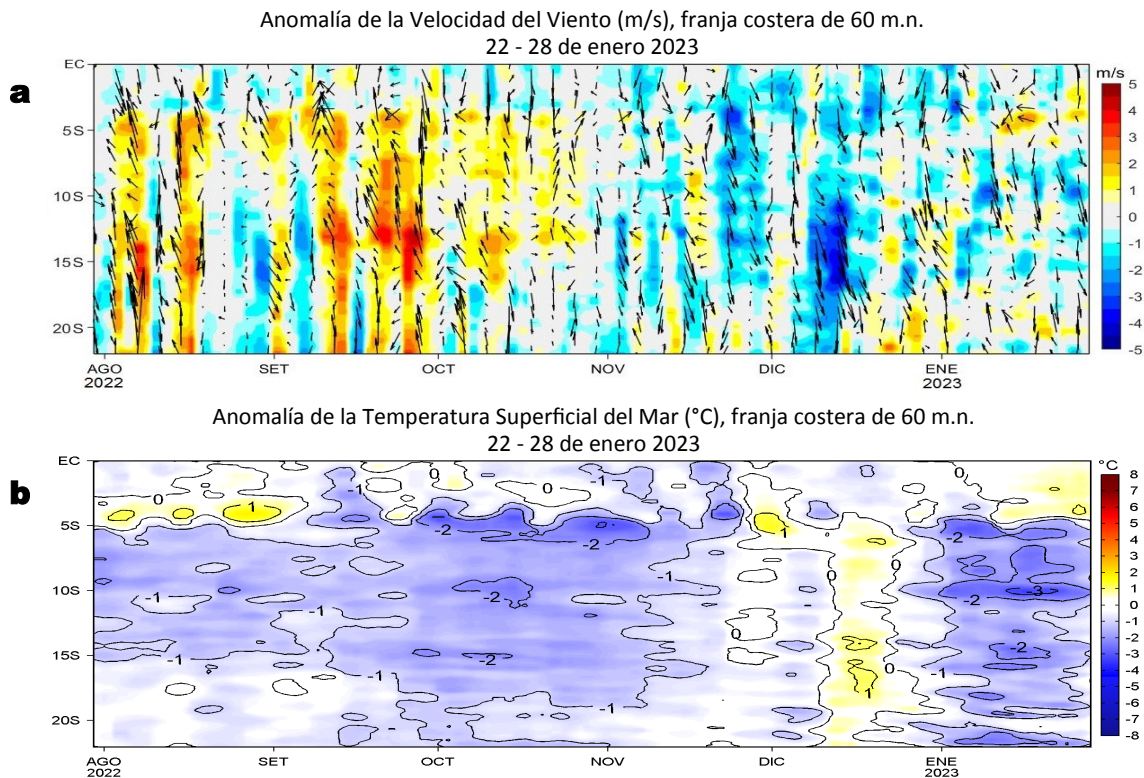
Figura 4. Evolución de las anomalías diarias de: a) Velocidad del viento (m/s) y b) Temperatura superficial del mar (°C) para el último semestre, actualizado al 28 de enero de 2023. Datos: de IFREMER/CERSAT para (a) y de OSTIA-UKMO -L4-GLOB-v2.0 para (b). Las anomalías fueron calculadas para una franja de 60 m.n. adyacente a la costa entre el ecuador geográfico y 22°S según los promedios climatológicos diarios de 2000-2014 para (a) y de 2007-2016 para (b). La barra de colores a la derecha muestra la escala de las anomalías en cada caso.
