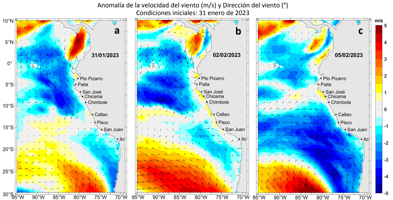
Figura 7. Distribución espacial del pronóstico de las anomalías de la velocidad del viento (m/s) y dirección del viento (°) para el a) 31 de enero, b) 02 y c) 05 de febrero de 2023, frente a la costa entre Panamá y Chile. Fuente: Modelo Climate Forecast System (GFS) de la NOAA.
