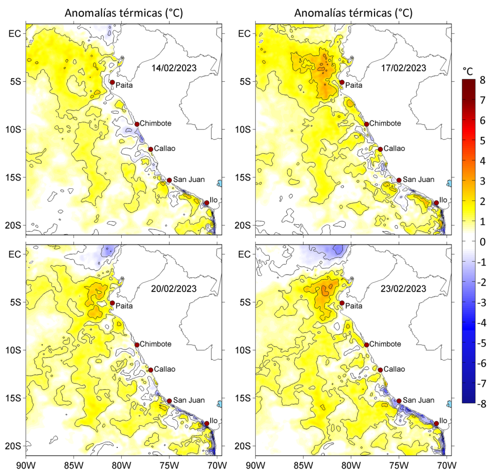
Figura 3. Anomalías de la temperatura superficial del mar (°C) para el a) 14, b) 17, c) 20 y d) 23 de febrero de 2023. Las anomalías se calcularon respecto de la climatología para el periodo 2007-2016. Datos: OSTIA-UKMO-L4-GLOB-v2.0 (UK Met Office, 2012; Donlon et al, 2012).
