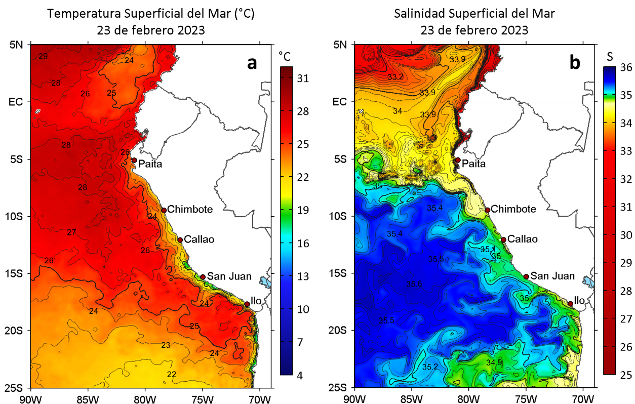
Figura 2. a) Temperatura superficial del mar (C) y b) Salinidad superficial del mar para el 23 de febrero de 2023. Datos: OSTIA-UKMO-L4-GLOB-v2.0 (UK Met Office, 2012; Donlon et al, 2012) y del GLOBAL_ANALYSIS_FORECAST_PHY_001_024 (Lellouche, J. M. et al, 2013), respectivamente.
