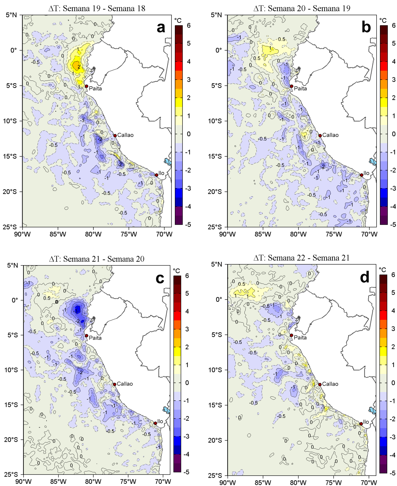
Figura 3. Variación semanal de la temperatura superficial del mar (°C) en el océano Pacífico tropical oriental entre: a) décimo novena (06-12 de mayo) y décimo octava (29 de abril - 05 de mayo) semana del 2020, b) vigésima (13-19 de mayo) y décimo novena (06-12 de mayo) semana del 2020, c) vigésima primera (20-26 de mayo) y vigésima (13-19 de mayo) semana del 2020 y d) vigésima segunda (27 de mayo - 02 de junio) y vigésima primera (20-26 de mayo) semana del 2020. Los mapas, que indican el grado de calentamiento o enfriamiento de una semana a otra, provienen de OSTIA-UKMO-L4-GLOB-v2.0 (UK Met Office, 2012; Donlon et al, 2012). La barra de colores a la derecha muestra la diferencia de la temperatura entre la presente y la semana previa. Procesamiento: LHFM/AFIOF/DGIOCC/IMARPE.
