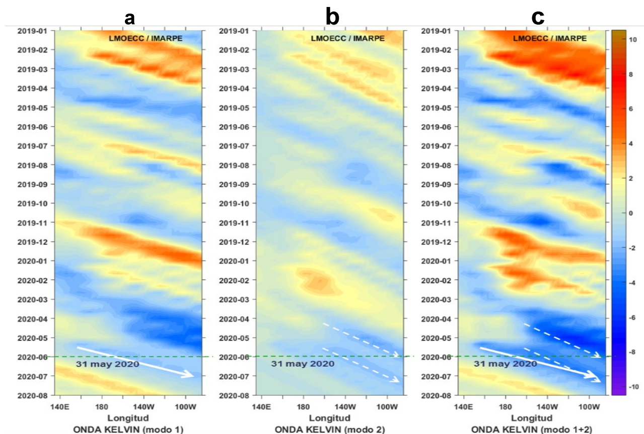
Figura 8. Diagramas Hovmöller longitudin-tiempo de las Ondas Kelvin Ecuatoriales (contribución de los modos baroclínicos a las anomalías del nivel mar (cm) en el Océano Pacífico Ecuatorial entre 130°E y 95°W forzado con anomalías del esfuerzo del viento ( N/m^2 ) del NCEP (Kalnay et al., 1996) de acuerdo con la metodología de Illig et al. (2004) y Dewitte et al. (2002): a) Modo 1, b) Modo 2 y c) Modos 1+2. La línea discontinua horizontal de color verde indica el inicio del pronóstico con anomalías del esfuerzo del viento igual a cero. Se graficó la contribución de los modos baroclínicos 1 (flechas continuas), modo 2 (flechas discontinuas) y la contribución conjunta modo 1+2 de las ondas Kelvin ecuatoriales a las anomalías del nivel del mar (cm). Los valores negativos corresponden a ondas Kelvin de afloramiento “frías” (flechas blancas).
