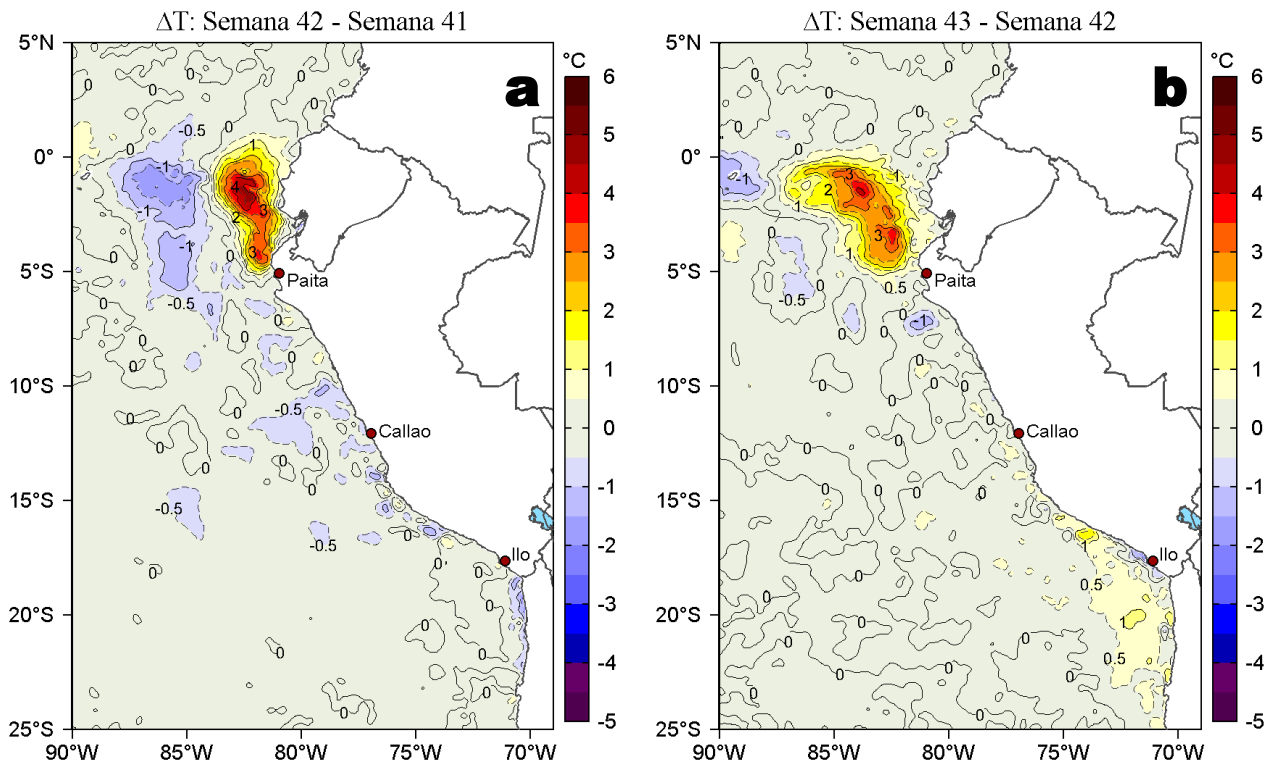
Figura 3. Variación semanal de la temperatura superficial del mar (°C) en el océano Pacífico tropical oriental entre: a) cuadragésima segunda (15-21 de octubre) y cuadragésima primera (08-14 de octubre) semana de 2021 y b) cuadragésima tercera (22-28 de octubre) y cuadragésima segunda (15-21 de octubre) semana de 2021. Los mapas, que indican el grado de calentamiento o enfriamiento de una semana a otra, provienen de OSTIA-UKMO-L4-GLOB-v2.0 (UK Met Office, 2012; Donlon et al, 2012). La barra de colores a la derecha muestra la diferencia de la temperatura entre la presente y la semana previa.
