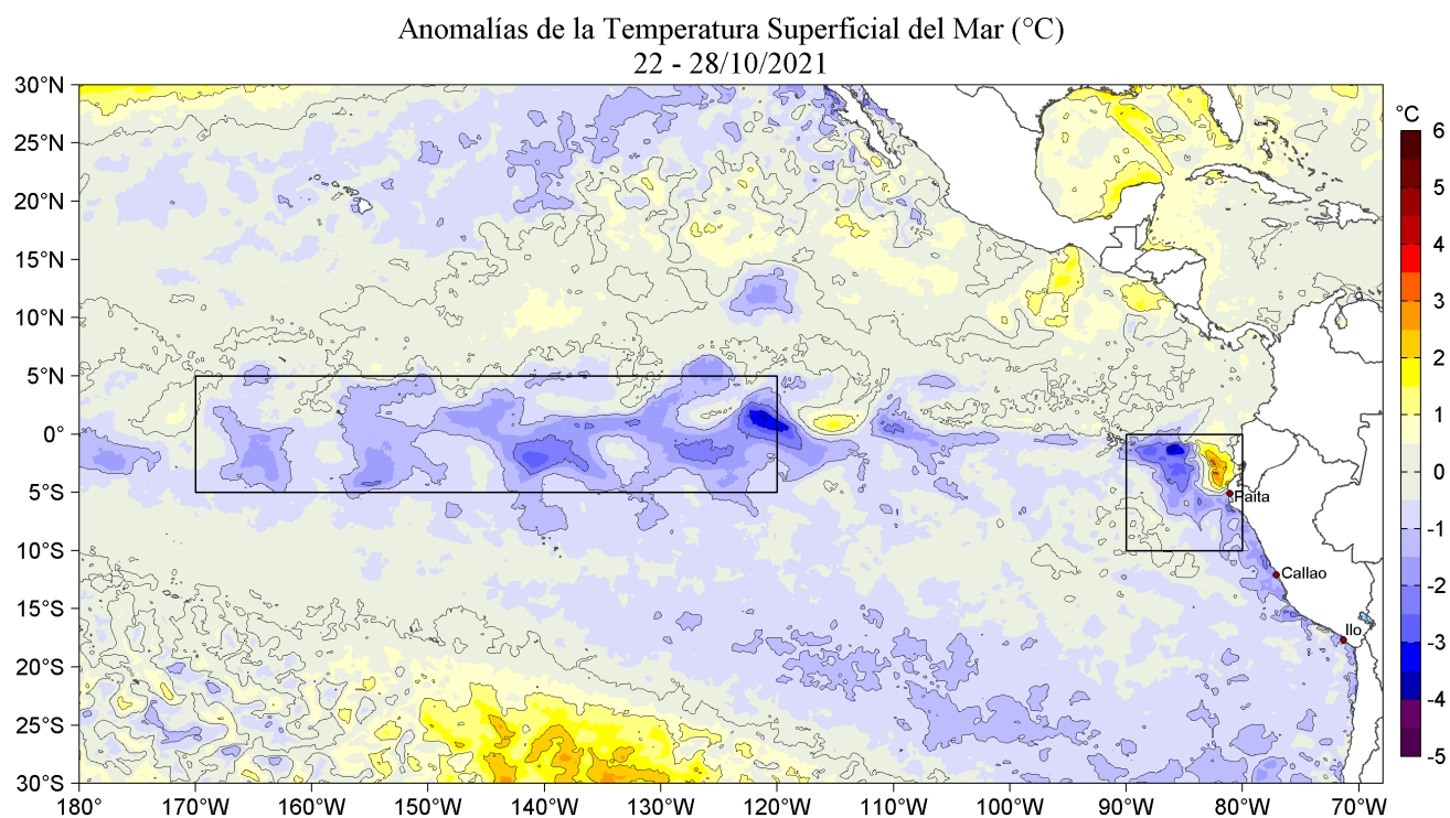
Figura 1. Anomalías promedio de la Temperatura superficial del mar (°C) en el océano Pacífico tropical para la semana del 22 al 28 de octubre de 2021. Las regiones Niño 3.4 y Niño 1+2 en los sectores central y oriental del océano, respectivamente están delimitadas con una línea de color gris. Datos: OSTIA-UKMO-L4-GLOB-v2.0 (UK Met Office, 2012; Donlon et al, 2012) disponible en https://podaac.jpl.nasa.gov/dataset/OSTIA-UKMO-L4-GLOB-v2.0 . Las anomalías se calcularon con respecto de la climatología para el período 2007-2016.
