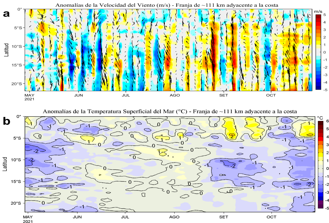
Figura 4. Evolución de las anomalías diarias de: a) Velocidad del viento (m/s) y b) Temperatura superficial del mar (°C) para el último semestre, actualizado al 27 y 28 de octubre de 2021, respectivamente. Datos: de IFREMER/CERSAT para (a) y de OSTIA-UKMO-L4-GLOB-v2.0 para (b). Las anomalías fueron calculadas para una franja de 111 km adyacente a la costa entre el ecuador geográfico y 22°S según los promedios climatológicos diarios de 2000-2014 para (a) y de 2007-2016 para (b). La barra de colores a la derecha muestra la escala de las anomalías en cada caso.
