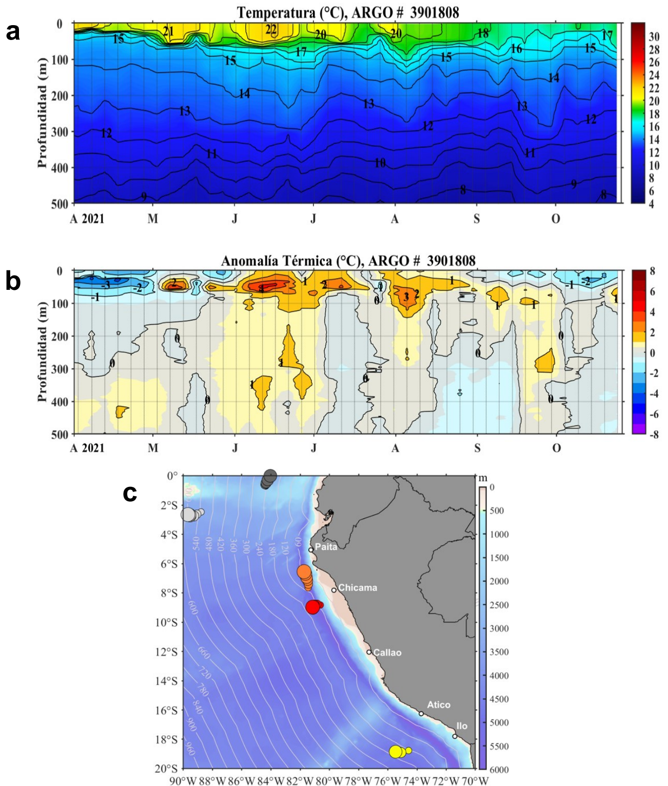
Figura 6. Diagrama Hovmöller de: a) Temperatura del mar (°C) y b) Anomalías térmicas (°C) del perfilador ARGO No. 3901808 localizado a 149 millas (8,98°S y 81,15°W) frente a Chicama del 01 de abril al 24 de octubre de 2021. Las anomalías de la temperatura del agua (°C) se calcularon de acuerdo a Domínguez et al (2017). Los puntos en la columna de agua indican los días en que el perfilador ARGO registró información. En la Figura (c) se muestra la ubicación de los perfiladores ARGO disponibles en el área de estudio. La ubicación del perfilador ARGO No. 3901808 se presenta con el círculo de color rojo. Datos: ARGO.
