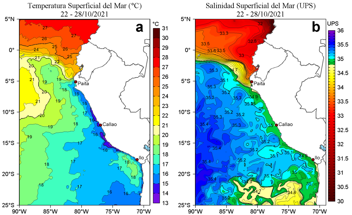
Figura 2. Distribución espacial promedio de: a) Temperatura (TSM, °C) y b) Salinidad superficial del mar (SSM) para la semana del 22 al 28 de octubre de 2021, en el océano Pacífico oriental. Datos: OSTIA-UKMO-L4-GLOB-v2.0 (UK Met Office, 2012; Donlon et al, 2012) disponible en http://podaac.jpl.nasa.gov/dataset/OSTIA-UKMO-L4-GLOB-v2.0 para (a) y del GLOBAL_ANALYSIS_FORECAST_PHY_001_024 (Lellouche, J. M. et al, 2013) disponible en http://marine.copernicus.eu/services-portfolio/access-to-products/?option=com_csw&view=details&product_id=GLOBAL_ANALYSIS_FORECAST_PHY_001_024 para (b). Las escalas de colores se presentan a la derecha de cada gráfico.
