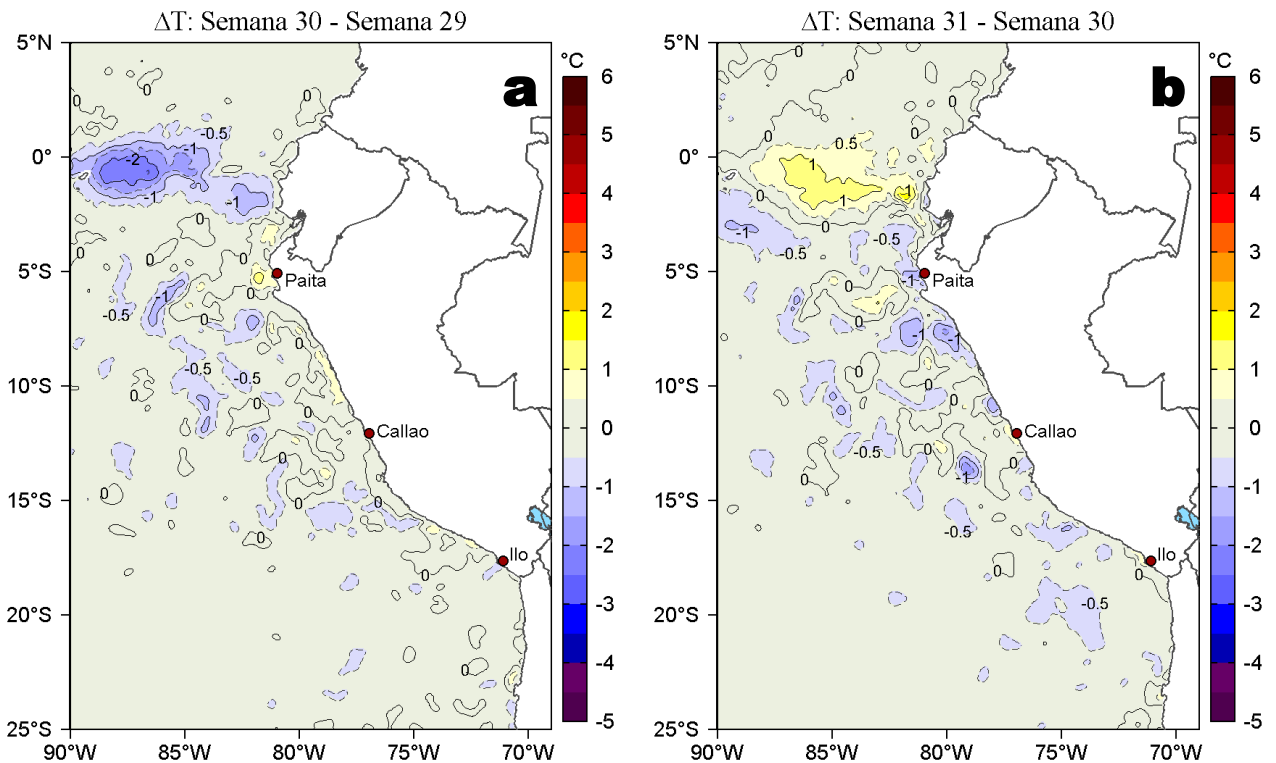
Figura 3. Variación semanal de la temperatura superficial del mar (°C) en el océano Pacífico tropical oriental entre: a) trigésima (23-29 de julio) y vigésima novena (16-22 de julio) semana de 2021 y b) trigésima primera (30 de julio - 05 de agosto) y trigésima (23-29 de julio) semana de 2021. Los mapas, que indican el grado de calentamiento o enfriamiento de una semana a otra, provienen de OSTIA-UKMO-L4-GLOB-v2.0 (UK Met Office, 2012; Donlon et al, 2012). La barra de colores a la derecha muestra la diferencia de la temperatura entre la presente y la semana previa.
