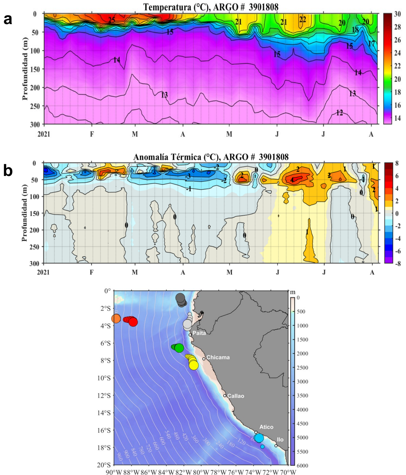
Figura 6. Diagrama Hovmöller de: a) Temperatura del mar (°C) y b) Anomalías térmicas (°C) del perfilador ARGO No. 3901808 localizado a 110 millas (8,56°S y 80,85°W) frente a Chicama del 01 de enero al 05 de agosto de 2021. Las anomalías de la temperatura del agua (°C) se calcularon de acuerdo a Domínguez et al (2017). Los puntos en la columna de agua indican los días en que el perfilador ARGO registró información. En la Figura (c) se muestra la ubicación de los perfiladores ARGO disponibles en el área de estudio. La ubicación del perfilador ARGO No. 3901808 se presenta con el círculo de color amarillo. Datos: ARGO.
