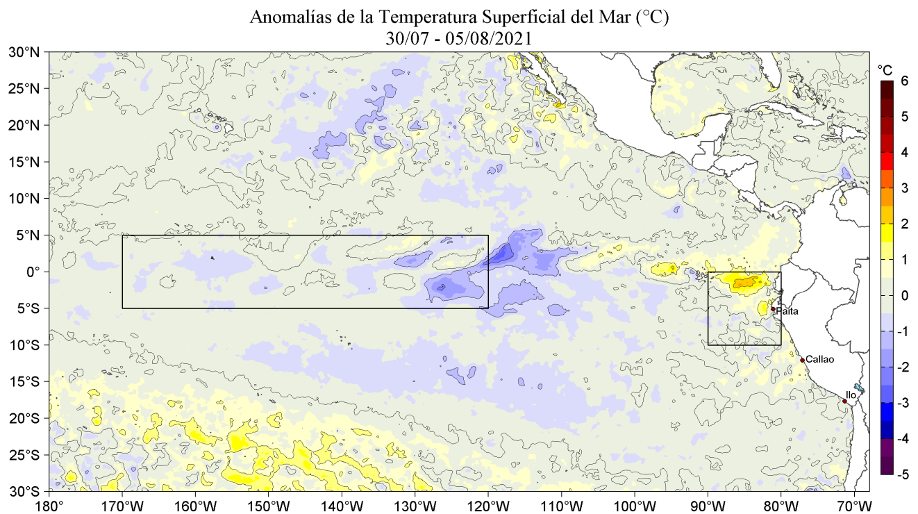
Figura 1. Anomalías promedio de la Temperatura superficial del mar (°C) en el océano Pacífico tropical para la semana del 30 de julio al 05 de agosto de 2021. Las regiones Niño 3.4 y Niño 1+2 en los sectores central y oriental del océano, respectivamente están delimitadas con una línea de color gris. Datos: OSTIA-UKMO-L4-GLOB-v2.0 (UK Met Office, 2012; Donlon et al, 2012) disponible en https://podaac.jpl.nasa.gov/dataset/OSTIA-UKMO-L4-GLOB-v2.0 . Las anomalías se calcularon con respecto de la climatología para el periodo 2007-2016.
