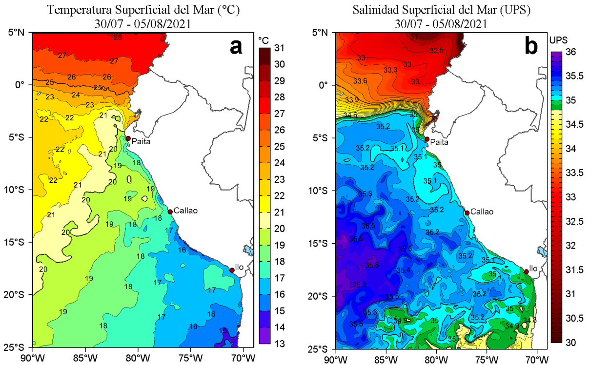
Figura 2. Distribución espacial promedio de: a) Temperatura (TSM, °C) y b) Salinidad superficial del mar (SSM) para la semana del 30 de julio al 05 de agosto de 2021, en el océano Pacífico oriental. Datos: OSTIA-UKMO-L4-GLOB-v2.0 (UK Met Office, 2012; Donlon et al, 2012) disponible en https://podaac.jpl.nasa.gov/dataset/OSTIA-UKMO-L4-GLOB-v2.0 para (a) y del GLOBAL_ANALYSIS_FORECAST_PHY_001_024 (Lellouche, J. M. et al, 2013) disponible en http://marine.copernicus.eu/services-portfolio/access-to-products/?option=com_csw&view=details&product_id=GLOBAL_ANALYSIS_FORECAST_PHY_001_024 para (b). Las escalas de colores se presentan a la derecha de cada gráfico.
