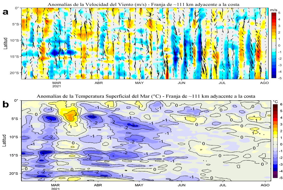
Figura 4. Evolución de las anomalías diarias de: a) Velocidad del viento (m/s) y b) Temperatura superficial del mar (°C) para el último semestre, actualizado al 04 y 05 de agosto de 2021, respectivamente. Datos: de IFREMER/CERSAT para (a) y de OSTIA-UKMO-L4-GLOB-v2.0 para (b). Las anomalías fueron calculadas para una franja de 111 km adyacente a la costa entre el ecuador geográfico y 22°S según los promedios climatológicos diarios de 2000-2014 para (a) y de 2007-2016 para (b). La barra de colores a la derecha muestra la escala de las anomalías en cada caso.
