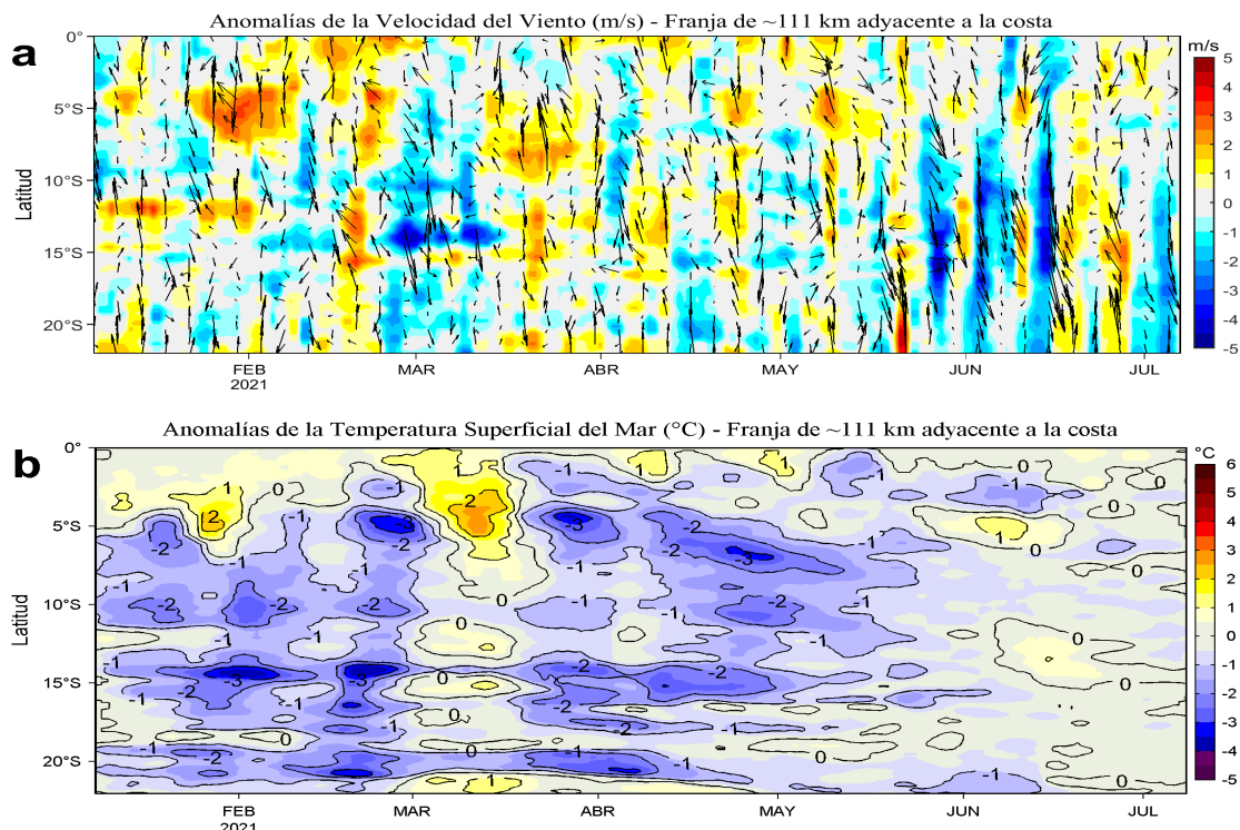
Figura 4. Evolución de las anomalías diarias de: a) Velocidad del viento (m/s) y b) Temperatura superficial del mar (°C) para el último semestre, actualizado al 07 y 08 de julio de 2021, respectivamente. Datos: de IFREMER/CERSAT para (a) y de OSTIA-UKMO-L4-GLOB-v2.0 para (b). Las anomalías fueron calculadas para una franja de 111 km adyacente a la costa entre el ecuador geográfico y 22°S según los promedios climatológicos diarios de 2000-2014 para (a) y de 2007-2016 para (b). La barra de colores a la derecha muestra la escala de las anomalías en cada caso.
