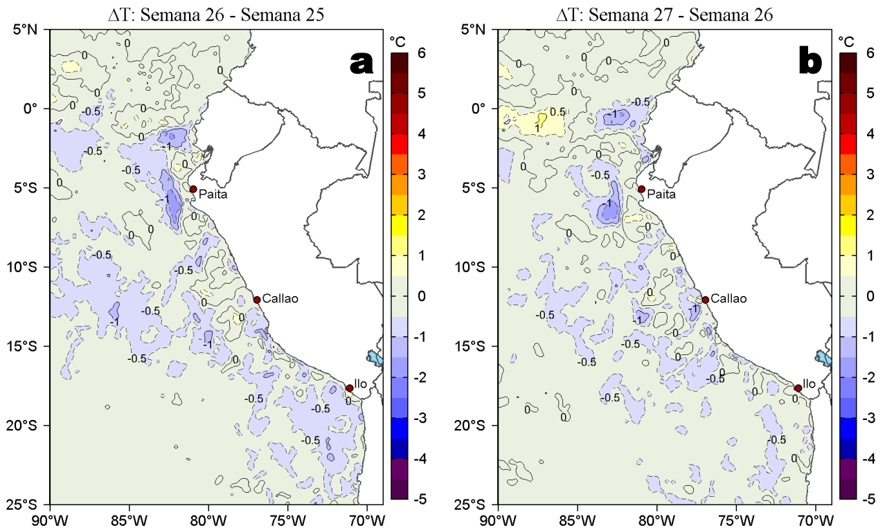
Figura 3. Variación semanal de la temperatura superficial del mar (°C) en el océano Pacífico tropical oriental entre: a) vigésima sexta (25 de junio - 01 de julio) y vigésima quinta (18-24 de junio) semana de 2021 y b) vigésima séptima (02-08 de julio) y vigésima sexta (25 de junio - 01 de julio) semana de 2021. Los mapas, que indican el grado de calentamiento o enfriamiento de una semana a otra, provienen de OSTIA-UKMO-L4-GLOB-v2.0 (UK Met Office, 2012; Donlon et al, 2012). La barra de colores a la derecha muestra la diferencia de la temperatura entre la presente y la semana previa.
