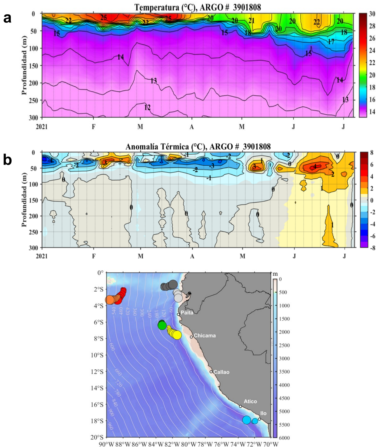
Figura 6. Diagrama Hovmöller de: a) Temperatura del mar (°C) y b) Anomalías térmicas (°C) del perfilador ARGO No. 3901808 localizado a 99 millas (7,6°S y 81,4°W) frente a Chicama del 01 de enero al 06 de julio de 2021. Las anomalías de la temperatura del agua (°C) se calcularon de acuerdo a Domínguez et al (2017). Los puntos en la columna de agua indican los días en que el perfilador ARGO registró información. En la Figura (c) se muestra la ubicación de los perfiladores ARGO disponibles en el área de estudio. La ubicación del perfilador ARGO No. 3901808 se presenta con el círculo de color amarillo. Datos: ARGO.
