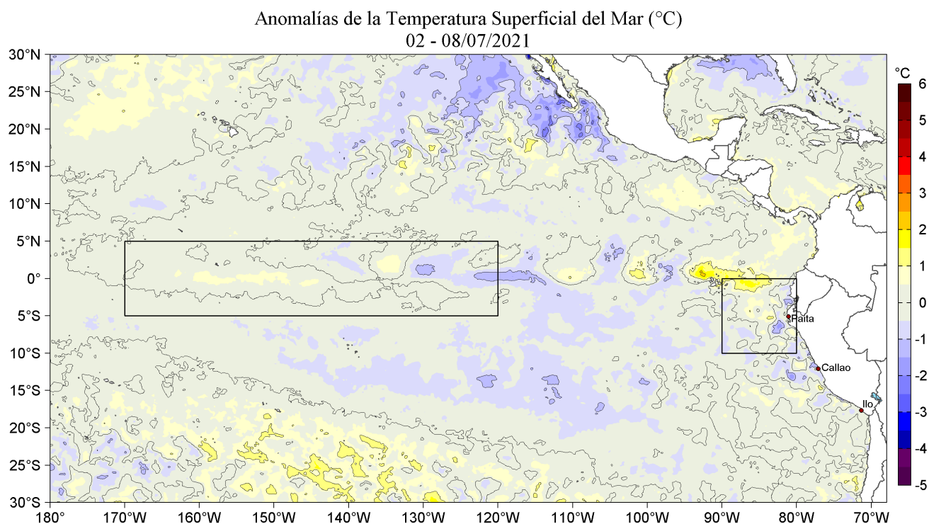
Figura 1. Anomalías promedio de la Temperatura superficial del mar (°C) en el océano Pacífico tropical para la semana del 02 al 08 de julio de 2021. Las regiones Niño 3.4 y Niño 1+2 en los sectores central y oriental del océano, respectivamente están delimitadas con una línea de color gris. Datos: OSTIA-UKMO-L4-GLOB-v2.0 (UK Met Office, 2012; Donlon et al, 2012) disponible en https://podaac.jpl.nasa.gov/dataset/OSTIA-UKMO-L4-GLOB-v2.0 . Las anomalías se calcularon con respecto de la climatología para el período 2007-2016.
