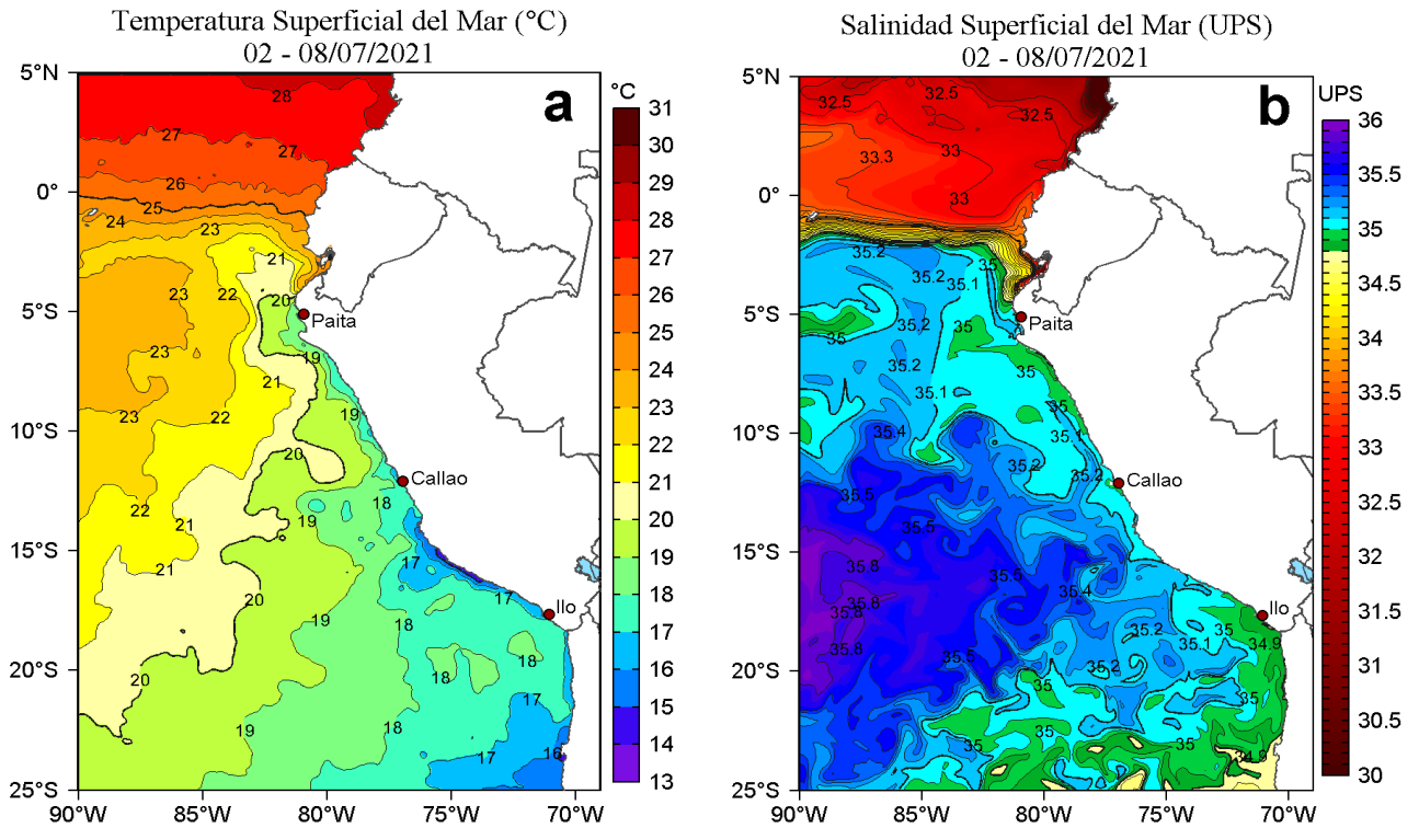
Figura 2. Distribución espacial promedio de: a) Temperatura (TSM, °C) y b) Salinidad superficial del mar (SSM) para la semana del 02 al 08 de julio de 2021, en el océano Pacífico oriental. Datos: OSTIA-UKMO-L4-GLOB-v2.0 (UK Met Office, 2012; Donlon et al, 2012) disponible en https://podaac.jpl.nasa.gov/dataset/OSTIA-UKMO-L4-GLOB-v2.0 para (a) y del GLOBAL_ANALYSIS_FORECAST_PHY_001_024 (Lellouche, J. M. et al, 2013) disponible en http://marine.copernicus.eu/services-portfolio/access-to-products/?option=com_csw&view=details&product_id=GLOBAL_ANALYSIS_FORECAST_PHY_001_024 para (b). Las escalas de colores se presentan a la derecha de cada gráfico.
