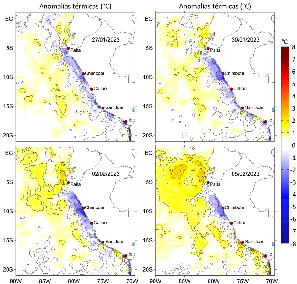
Figura 3. Anomalías de la temperatura superficial del mar (°C) para el a) 27 y b) 30 de enero, así como para el c) 02 y d) 05 de febrero de 2023. Las anomalías se calcularon respecto de la climatología para el periodo 2007-2016. Datos: OSTIA-UKMO-L4-GLOB-v2.0 (UK Met Office, 2012; Donlon et al, 2012).
