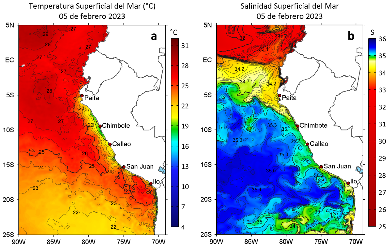
Figura 2. a) Temperatura superficial del mar (C) y b) Salinidad superficial del mar para el 05 de febrero de 2023. Datos: OSTIA-UKMO-L4-GLOB-v2.0 (UK Met Office, 2012; Donlon et al, 2012) y del GLOBAL_ANALYSIS_FORECAST_PHY_001_024 (Lellouche, J. M. et al, 2013), respectivamente.
