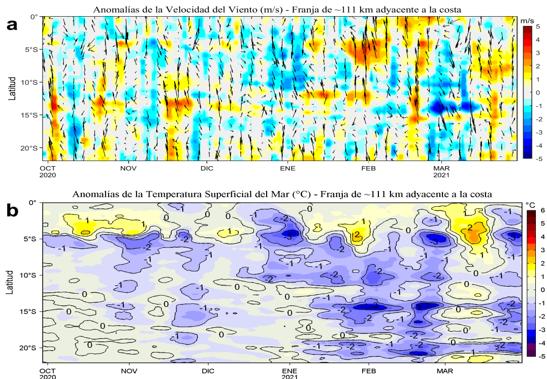
Figura 4. Evolución de las anomalías diarias de: a) Velocidad del viento (m/s) y b) Temperatura superficial del mar (°C) para el último semestre, actualizado al 30 de marzo de 2021. Datos: de IFREMER/CERSAT para (a) y de OSTIA-UKMO-L4-GLOB-v2.0 para (b). Las anomalías fueron calculadas para una franja de 111 km adyacente a la costa entre el ecuador geográfico y 22°S según los promedios climatológicos diarios de 2000-2014 para (a) y de 2007-2016 para (b). La barra de colores a la derecha muestra la escala de las anomalías en cada caso.
