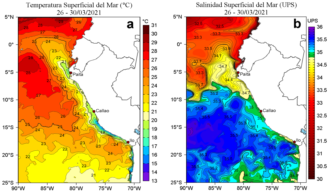
Figura 2. Distribución espacial promedio de: a) Temperatura (TSM, °C) y b) Salinidad superficial del mar (SSM) para la semana del 26 al 30 de marzo de 2021, en el océano Pacífico oriental. Datos: OSTIA-UKMO-L4-GLOB-v2.0 (UK Met Office, 2012; Donlon et al, 2012) disponible en https://podaac.jpl.nasa.gov/dataset/OSTIA-UKMO-L4-GLOB-v2.0 para (a) y del GLOBAL_ANALYSIS_FORECAST_PHY_001_024 (Lellouche, J. M. et al, 2013) disponible en http://marine.copernicus.eu/services-portfolio/access-to-products/?option=com_csw&view=details&product_id=GLOBAL_ANALYSIS_FORECAST_PHY_001_024 para (b). Las escalas de colores se presentan a la derecha de cada gráfico.
