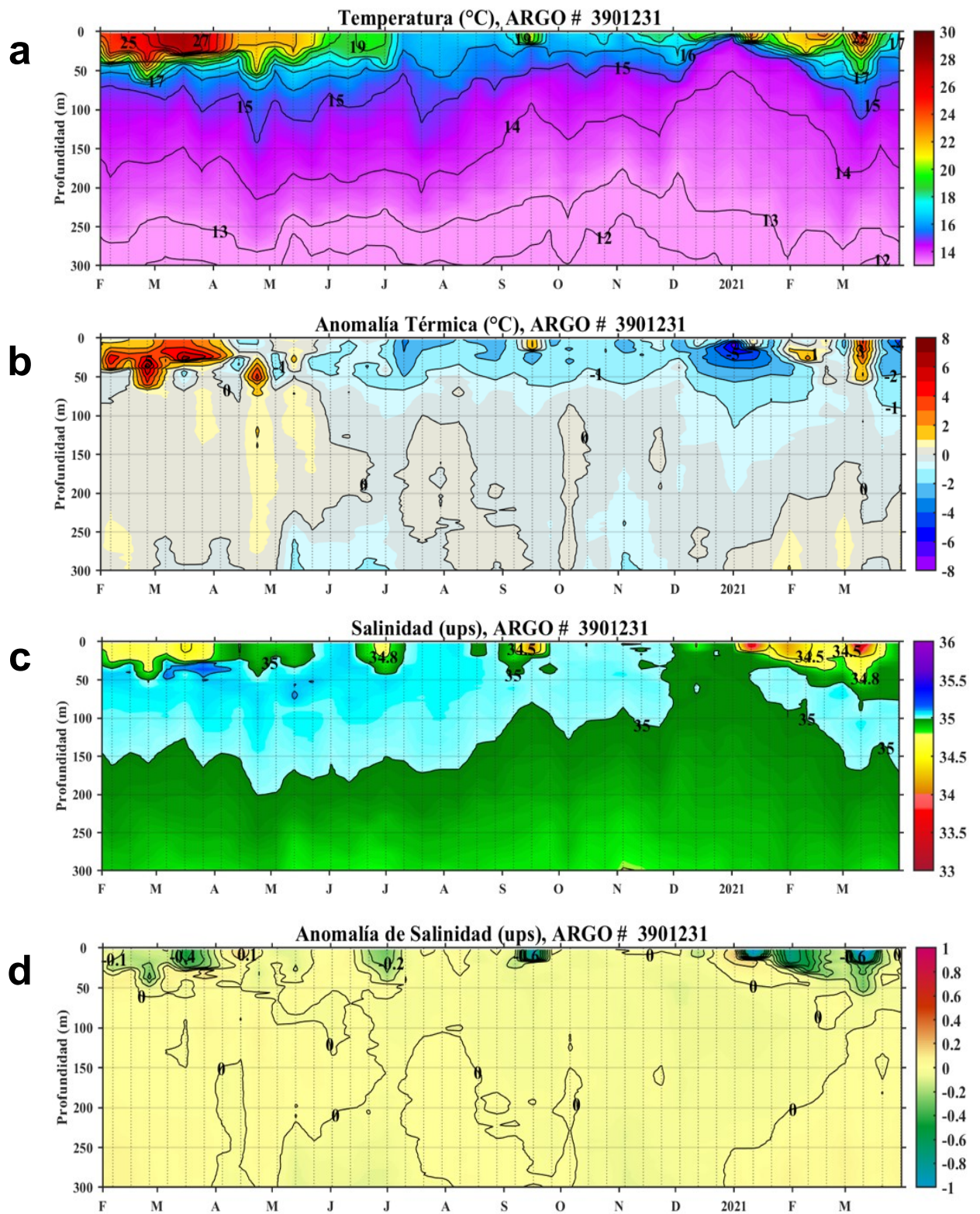
Figura 6. Diagrama Hovmöller de: a) Temperatura del mar (°C), b) Anomalías térmicas (°C), c) Salinidad del agua de mar (ups) y d) Anomalia de la salinidad del mar (ups) a 10 millas (5,96°S y 81,34°W) frente a Punta Falsa de febrero del 2020 al 30 de marzo de 2021. Las anomalías de la temperatura del agua (°C) y de salinidad (ups) se calcularon de acuerdo a Domínguez et al (2017). Los puntos en la columna de agua indican los días en que el perfilador ARGO registró información. La ubicación del perfilador ARGO No. 3901231 se presenta con el círculo de color amarillo en el gráfico de la derecha. Datos: ARGO.
