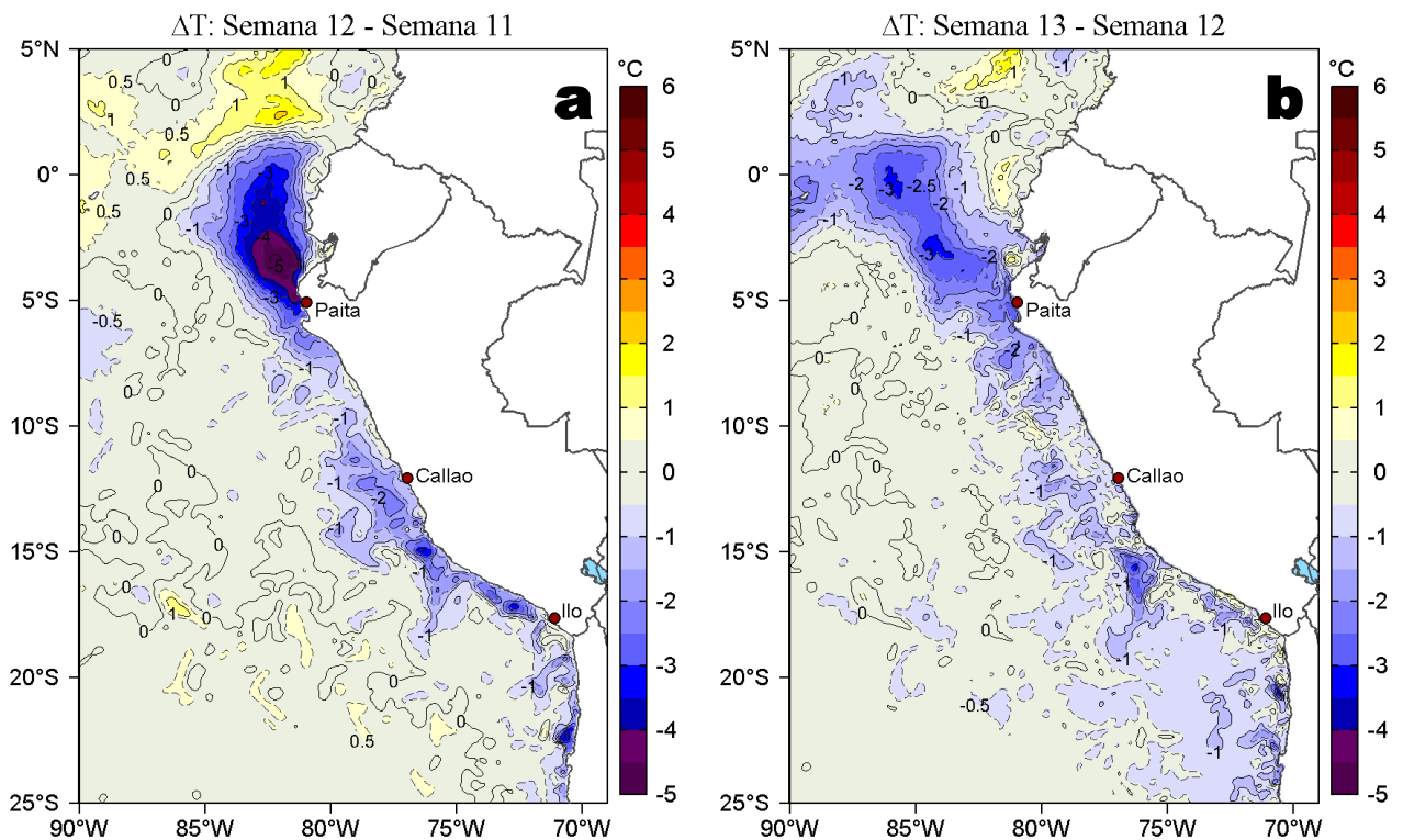
Figura 3. Variación semanal de la temperatura superficial del mar (°C) en el océano Pacífico tropical oriental entre: a) décima segunda (19-25 de marzo) y décima primera (12-18 de marzo) semana del 2021 y b) décima tercera (26-30 de marzo) y décima segunda (19-25 de marzo) semana del 2021. Los mapas, que indican el grado de calentamiento o enfriamiento de una semana a otra, provienen de OSTIA-UKMO-L4-GLOB-v2.0 (UK Met Office, 2012; Donlon et al, 2012). La barra de colores a la derecha muestra la diferencia de la temperatura entre la presente y la semana previa.
