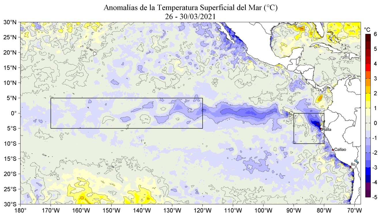
Figura 1. Anomalías promedio de la Temperatura superficial del mar (°C) en el océano Pacífico tropical para la semana del 26 al 30 de marzo de 2021. Las regiones Niño 3.4 y Niño 1+2 en los sectores central y oriental del océano, respectivamente están delimitadas con una línea de color gris. Datos: OSTIA-UKMO-L4-GLOB-v2.0 (UK Met Office, 2012; Donlon et al, 2012) disponible en https://podaac.jpl.nasa.gov/dataset/OSTIA-UKMO-L4-GLOB-v2.0 . Las anomalías se calcularon con respecto de la climatología para el periodo 2007-2016.
