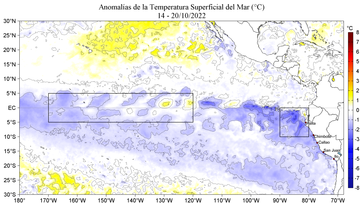
Figura 1. Anomalías promedio de la Temperatura superficial del mar (°C) en el océano Pacífico tropical para la semana del 14 al 20 de octubre de 2022. Las regiones Niño 3.4 y Niño 1+2 en los sectores central y oriental del océano, respectivamente están delimitadas con una línea de color gris. Datos: OSTIA-UKMO-L4-GLOB-v2.0 (UK Met Office, 2012; Donlon et al, 2012) disponible en https://podaac.jpl.nasa.gov/dataset/OSTIA-UKMO-L4-GLOB-v2.0 . Las anomalías se calcularon con respecto de la climatología para el período 2007-2016.
