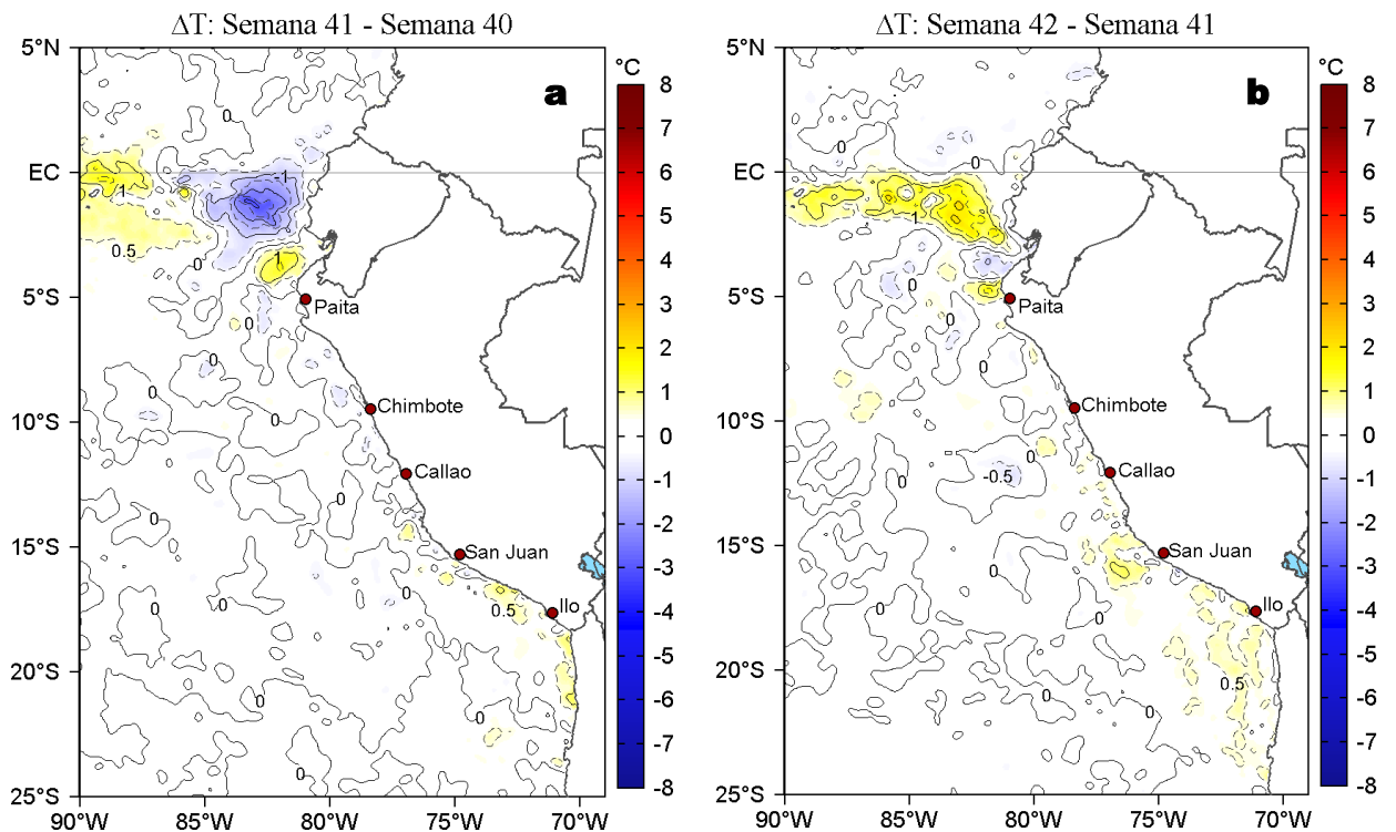
Figura 3. Variación semanal de la temperatura superficial del mar (°C) en el océano Pacífico tropical oriental entre: a) cuadragésima primera (07-13 de octubre) y cuadragésima (30 de setiembre - 06 de octubre) semana de 2022 y b) cuadragésima segunda (14-20 de octubre) y cuadragésima primera (07-13 de octubre) semana de 2022. Los mapas, que indican el grado de calentamiento o enfriamiento de una semana a otra, provienen de OSTIA-UKMO-L4-GLOB-v2.0 (UK Met Office, 2012; Donlon et al, 2012). La barra de colores a la derecha muestra la diferencia de la temperatura entre la presente y la semana previa.
