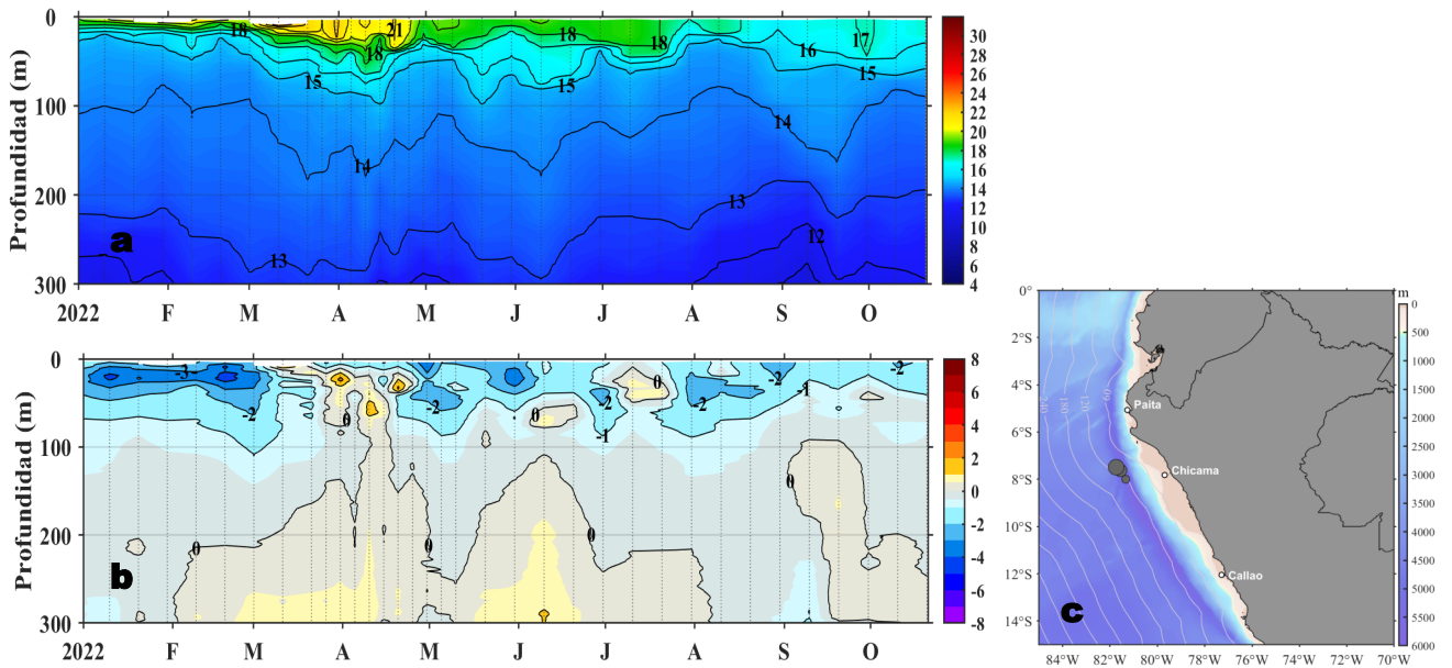
Figura 7. Diagrama Hovmöller de: a) Temperatura del mar (°C) y b) Anomalías térmicas (°C), registradas por el perfilador ARGO No. 6903003 localizado a 91 m.n. (7,49°S, 81,74°W) de Chicama el 20 de octubre de 2022, respectivamente. Las anomalías de la temperatura del agua se calcularon de acuerdo a Dominguez et al (2017). Los puntos en la columna de agua indican los días en que el perfilador registró información. La Figura 7 c muestra la ubicación de los perfiladores. Datos: ARGO.
