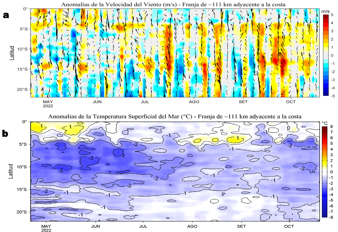
Figura 4. Evolución de las anomalías diarias de: a) Velocidad del viento (m/s) y b) Temperatura superficial del mar (°C) para el último semestre, actualizado al 19 y 20 de octubre 2022, respectivamente. Datos: de IFREMER/CERSAT para (a) y de OSTIA-UKMO-L4-GLOB-v2.0 para (b). Las anomalías fueron calculadas para una franja de 111 km adyacente a la costa entre el ecuador geográfico y 22°S según los promedios climatológicos diarios de 2000-2014 para (a) y de 2007-2016 para (b). La barra de colores a la derecha muestra la escala de las anomalías en cada caso.
