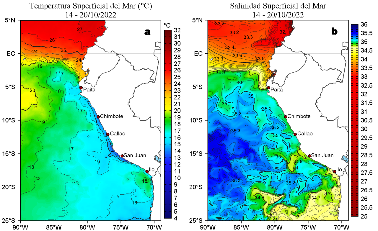
Figura 2. Distribución espacial promedio de: a) Temperatura (TSM, °C) y b) Salinidad superficial del mar (SSM) para la semana del 14 al 20 de octubre de 2022, en el océano Pacífico oriental. Datos: OSTIA-UKMO-L4-GLOB-v2.0 (UK Met Office, 2012; Donlon et al, 2012) disponible en https://podaac.jpl.nasa.gov/dataset/OSTIA-UKMO-L4-GLOB-v2.0 para (a) y del GLOBAL_ANALYSIS_FORECAST_PHY_001_024 (Lellouche, J. M. et al, 2013) disponible en http://marine.copernicus.eu/services-portfolio/access-to-products/?option=com_csw&view=details&product_id=GLOBAL_ANALYSIS_FORECAST_PHY_001_024 para (b). Las escalas de colores se presentan a la derecha de cada gráfico.
