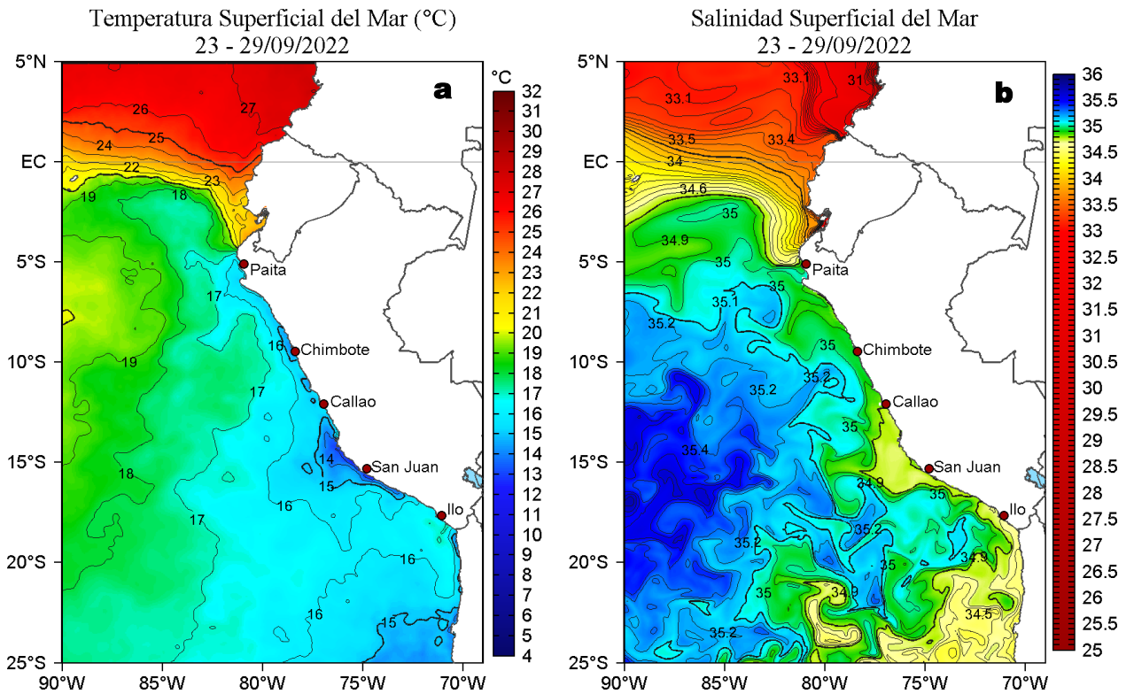
Figura 2. Distribución espacial promedio de: a) Temperatura (TSM, °C) y b) Salinidad superficial del mar (SSM) para la semana del 23 al 29 de setiembre de 2022, en el océano Pacífico oriental. Datos: OSTIA-UKMO-L4-GLOB-v2.0 (UK Met Office, 2012; Donlon et al, 2012) disponible en https://podaac.jpl.nasa.gov/dataset/OSTIA-UKMO-L4-GLOB-v2.0 para (a) y del GLOBAL ANALYSIS FORECAST PHY 001_024 (Lellouche, J. M. et al, 2013) disponible en http://marine.copernicus.eu/services-portfolio/access-to-products/?option=com_csw&view=details&product_id=GLOBAL_ANALYSIS_FORECAST_PHY_001_024 para (b). Las escalas de colores se presentan a la derecha de cada gráfico.
