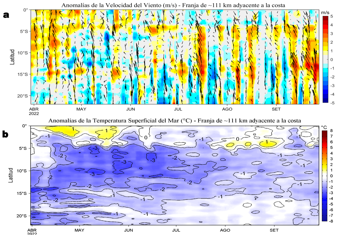
Figura 4. Evolución de las anomalías diarias de: a) Velocidad del viento (m/s) y b) Temperatura superficial del mar (°C) para el último semestre, actualizado al 28 y 29 de setiembre 2022, respectivamente. Datos: de IFREMER/CERSAT para (a) y de OSTIA-UKMO-L4-GLOB-v2.0 para (b). Las anomalías fueron calculadas para una franja de 111 km adyacente a la costa entre el ecuador geográfico y 22°S según los promedios climatológicos diarios de 2000-2014 para (a) y de 2007-2016 para (b). La barra de colores a la derecha muestra la escala de las anomalías en cada caso.
