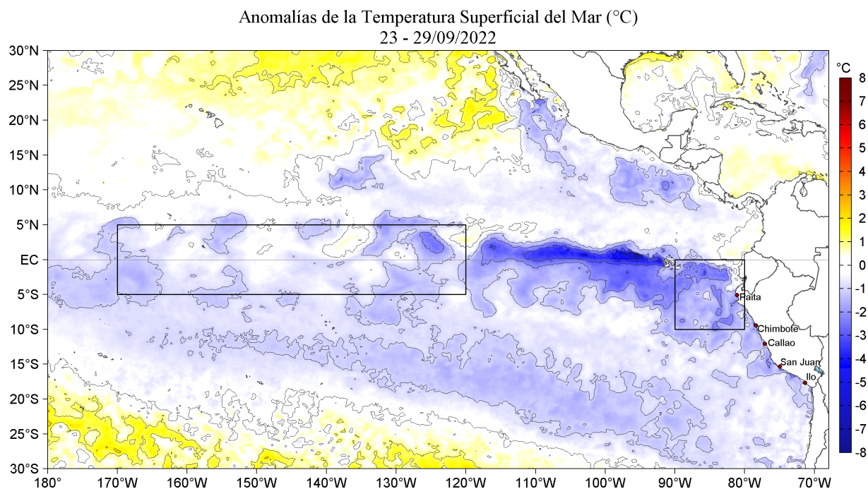
Figura 1. Anomalías promedio de la Temperatura superficial del mar (°C) en el océano Pacífico tropical para la semana del 23 al 29 de setiembre de 2022. Las regiones Niño 3.4 y Niño 1+2 en los sectores central y oriental del océano, respectivamente están delimitadas con una línea de color gris. Datos: OSTIA-UKMO-L4-GLOB-v2.0 (UK Met Office, 2012; Donlon et al, 2012) disponible en https://podaac.jpl.nasa.gov/dataset/OSTIA-UKMO-L4-GLOB-v2.0 . Las anomalías se calcularon con respecto de la climatología para el período 2007-2016.
