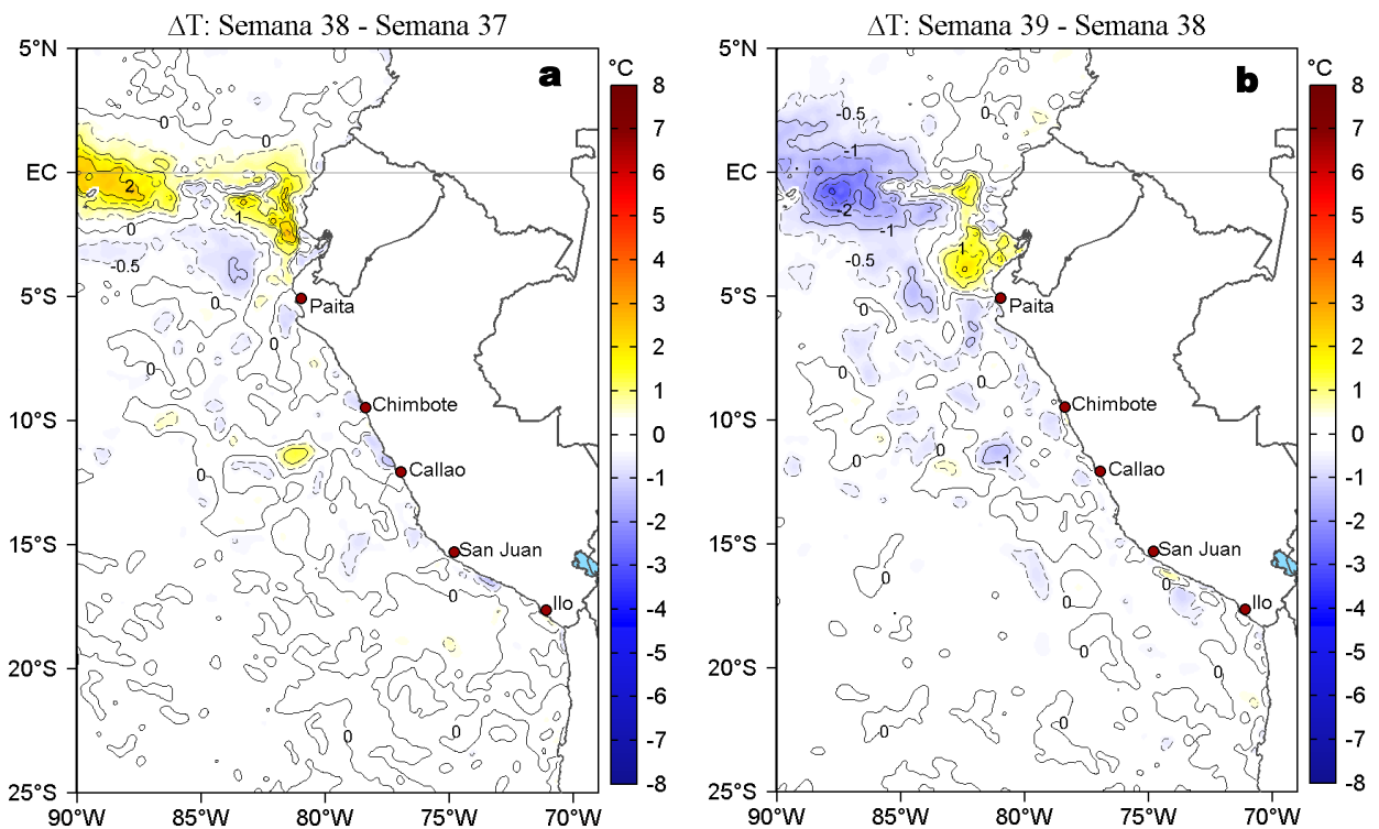
Figura 3. Variación semanal de la temperatura superficial del mar (°C) en el océano Pacífico tropical oriental entre: a) trigésima octava (16-22 de setiembre) y trigésima séptima (09-15 de setiembre) semana de 2022 y b) trigésima novena (23-29 de setiembre) y trigésima octava (16-22 de setiembre) semana de 2022. Los mapas, que indican el grado de calentamiento o enfriamiento de una semana a otra, provienen de OSTIA-UKMO-L4-GLOB-v2.0 (UK Met Office, 2012; Donlon et al, 2012). La barra de colores a la derecha muestra la diferencia de la temperatura entre la presente y la semana previa.
