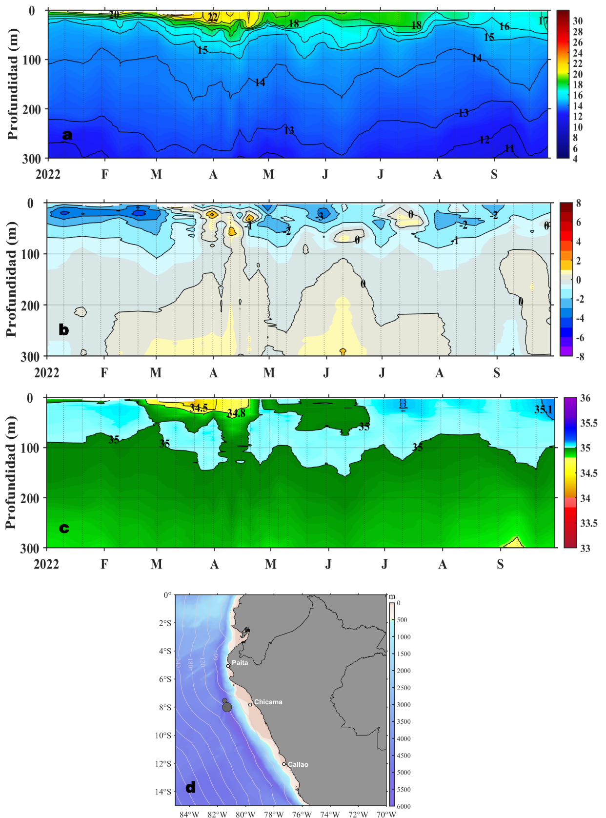
Figura 6. Diagrama Hovmöller de: a) Temperatura del mar (°C), b) Anomalías térmicas (°C) y c) Salinidad del mar, registradas por el perfilador ARGO No. 6903003 localizado a 109 m.n. (8,00°S, 81,34°W) de Chicama el 30 de setiembre de 2022, respectivamente. Las anomalías de la temperatura del agua se calcularon de acuerdo a Domínguez et al (2017). Los puntos en la columna de agua indican los días en que el perfilador registró información. La Figura 6 d muestra la ubicación de los perfiladores. Datos: ARGO.
