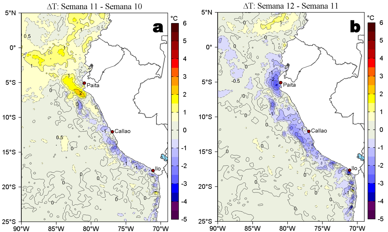
Figura 3. Variación semanal de la temperatura superficial del mar (°C) en el océano Pacífico tropical oriental entre: a) décima primera (11-17 de marzo) y décima (04-10 de marzo) semana de 2022 y b) décima segunda (18-24 de marzo) y décima primera (11-17 de marzo) semana de 2022. Los mapas, que indican el grado de calentamiento o enfriamiento de una semana a otra, provienen de OSTIA-UKMO-L4-GLOB-v2.0 (UK Met Office, 2012; Donlon et al, 2012). La barra de colores a la derecha muestra la diferencia de la temperatura entre la presente y la semana previa.
