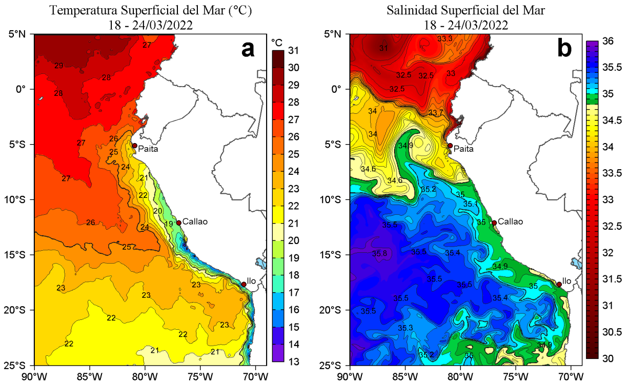
Figura 2. Distribución espacial promedio de: a) Temperatura (TSM, °C) y b) Salinidad superficial del mar (SSM) para la semana del 18 al 24 de marzo de 2022, en el océano Pacífico oriental. Datos: OSTIA-UKMO-L4-GLOB-v2.0 (UK Met Office, 2012; Donlon et al, 2012) disponible en http://podaac.jpl.nasa.gov/dataset/OSTIA-UKMO-L4-GLOB-v2.0 para (a) y del GLOBAL_ANALYSIS_FORECAST_PHY_001_024 (Lellouche, J. M. et al, 2013) disponible en http://marine.copernicus.eu/services-portfolio/access-to-products/?option=com_csw&view=details&product_id=GLOBAL_ANALYSIS_FORECAST_PHY_001_024 para (b). Las escalas de colores se presentan a la derecha de cada gráfico.
