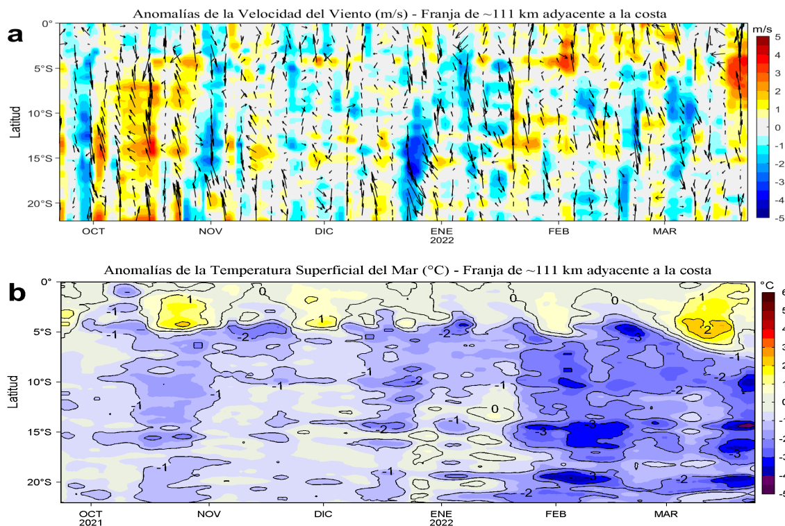
Figura 4. Evolución de las anomalías diarias de: a) Velocidad del viento (m/s) y b) Temperatura superficial del mar (°C) para el último semestre, actualizado al 23 y 24 de marzo de 2022, respectivamente. Datos: de IFREMER/CERSAT para (a) y de OSTIA-UKMO-L4-GLOB-v2.0 para (b). Las anomalías fueron calculadas para una franja de 111 km adyacente a la costa entre el ecuador geográfico y 22°S según los promedios climatológicos diarios de 2000-2014 para (a) y de 2007-2016 para (b). La barra de colores a la derecha muestra la escala de las anomalías en cada caso.
