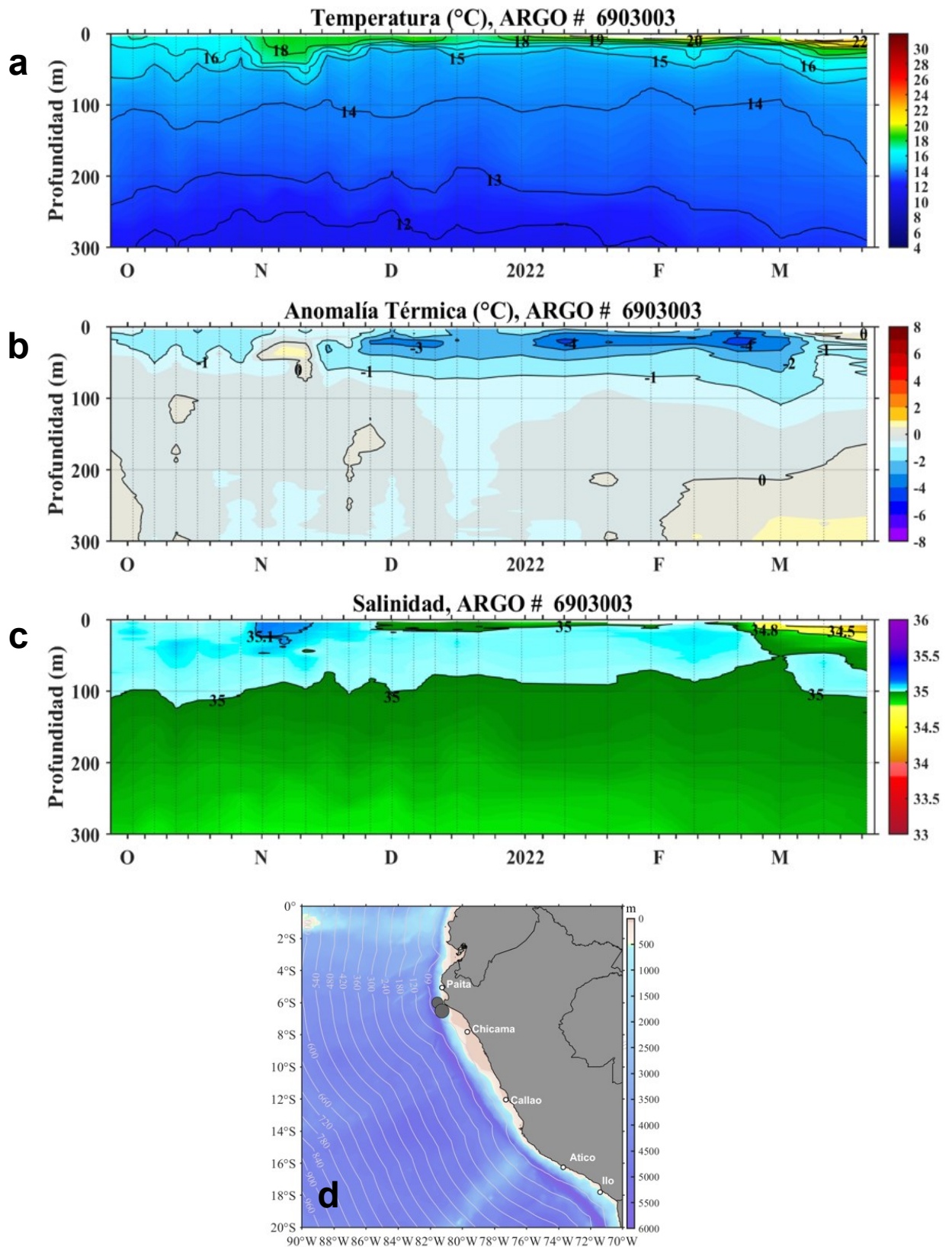
Figura 6. Diagrama Hovmöller de: a) Temperatura del mar (°C), b) Anomalías térmicas (°C) y c) Salinidad del mar, registradas por el perfilador ARGO No. 6903003 localizado a 30 m. n. (6,52 °S, 81,27 °W) de Punta Falsa el día 21 de marzo de 2022. Las anomalías de la temperatura del agua (Figura 6 b) se calcularon de acuerdo a Domínguez et al (2017). Los puntos en la columna de agua indican los días en que el perfilador registró información. La Figura 6 d muestra la ubicación del perfilador. Datos: ARGO.
