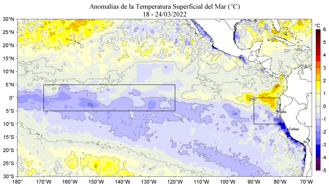
Figura 1. Anomalías promedio de la Temperatura superficial del mar ( ^{\circ}\text{C} ) en el océano Pacífico tropical para la semana del 18 al 24 de marzo de 2022. Las regiones Niño 3.4 y Niño 1+2 en los sectores central y oriental del océano, respectivamente están delimitadas con una línea de color gris. Datos: OSTIA-UKMO-L4-GLOB-v2.0 (UK Met Office, 2012; Donlon et al, 2012) disponible en https://podaac.jpl.nasa.gov/dataset/OSTIA-UKMO-L4-GLOB-v2.0 . Las anomalías se calcularon con respecto de la climatología para el periodo 2007-2016.
