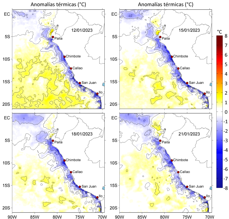
Figura 3. Anomalías de la temperatura superficial del mar (°C) para el a) 12, b) 15, c) 18 y d) 21 de enero de 2023. Las anomalías se calcularon respecto de la climatología para el periodo 2007-2016. Datos: OSTIA-UKMO-L4-GLOB-v2.0 (UK Met Office, 2012; Donlon et al, 2012).
