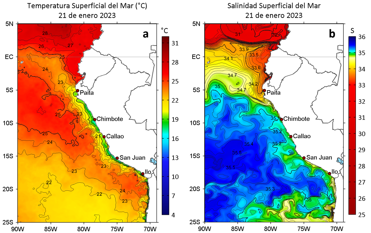
Figura 2. a) Temperatura superficial del mar (°C) y b) Salinidad superficial del mar para el 21 de enero de 2023. Datos: OSTIA-UKMO-L4-GLOB-v2.0 (UK Met Office, 2012; Donlon et al, 2012) y del GLOBAL_ANALYSIS_FORECAST_PHY_001_024 (Lellouche, J. M. et al, 2013), respectivamente.
