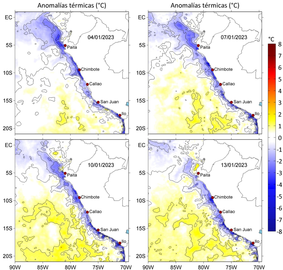
Figura 3. Anomalías de la temperatura superficial del mar (°C) para el a) 04, b) 07, c) 10 y d) 13 de enero de 2023. Las anomalías se calcularon respecto de la climatología para el periodo 2007-2016. Datos: OSTIA-UKMO-L4-GLOB-v2.0 (UK Met Office, 2012; Donlon et al, 2012).
