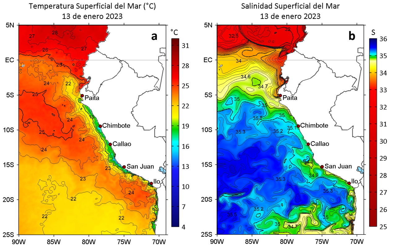
Figura 2. a) Temperatura superficial del mar (°C) y b) Salinidad superficial del mar para el 13 de enero de 2023. Datos: OSTIA-UKMO-L4-GLOB-v2.0 (UK Met Office, 2012; Donlon et al, 2012) y del GLOBAL_ANALYSIS_FORECAST_PHY_001_024 (Lellouche, J. M. et al, 2013), respectivamente.
