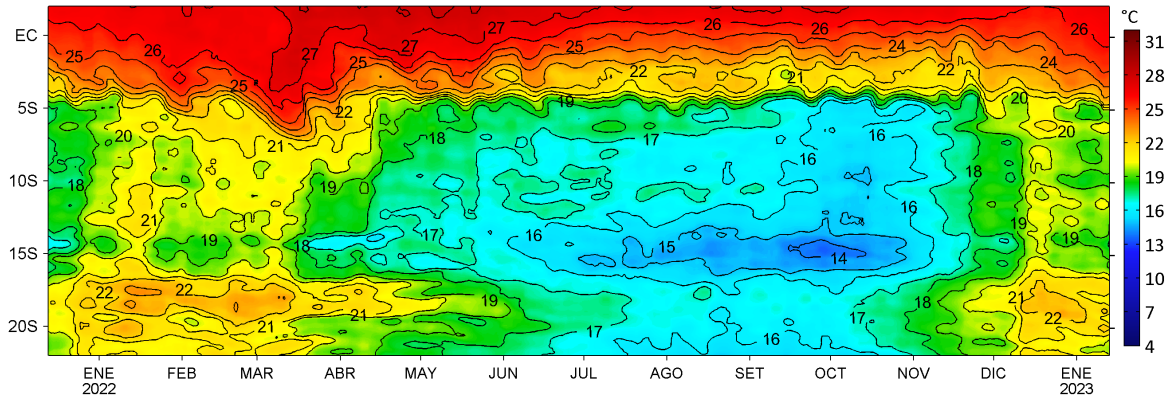
Anomalías de la Temperatura Superficial del mar (°C), franja costera de 60 m.n. 13 de diciembre 2021 - 13 de enero 2023
