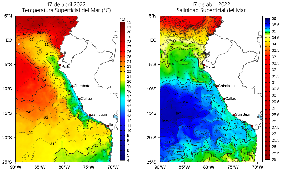
Figura 2. Temperatura superficial del mar (a la izquierda) y Salinidad superficial del mar (a la derecha) para el 17 de abril de 2022. Datos: OSTIA-UKMO-L4-GLOB-v2.0 (UK Met Office, 2012; Donlon et al, 2012) y Hybrid Coordinate Ocean Model v. GOFS 3.1 (HYCOM; Halliwell et al., 1998; 2000; Bleck, 2001), respectivamente.
