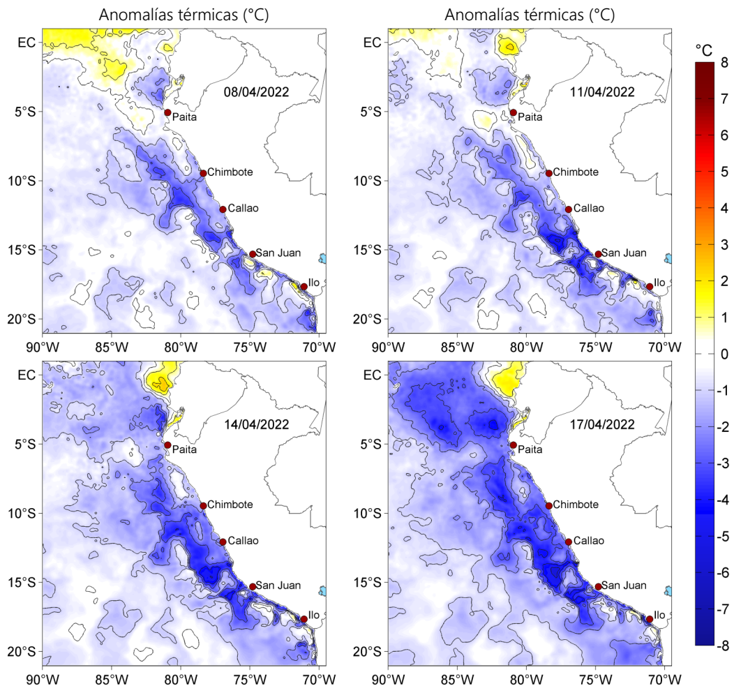
Figura 3. Anomalías de la temperatura superficial del mar (°C) para el 08, 11, 14 y 17 de abril de 2022. Las anomalías se calcularon respecto de la climatología para el periodo 2007-2016. Datos: OSTIA-UKMO-L4-GLOB-v2.0 (UK Met Office, 2012; Donlon et al, 2012).
