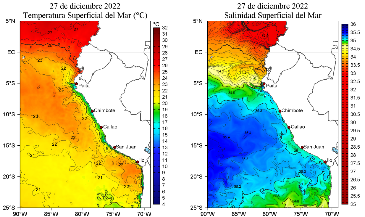
Figura 2. Temperatura superficial del mar (a la izquierda) y Salinidad superficial del mar (a la derecha) para el 27 de diciembre de 2022. Datos: OSTIA-UKMO-L4-GLOB-v2.0 (UK Met Office, 2012; Donlon et al, 2012) y Hybrid Coordinate Ocean Model v. GOFS 3.1 (HYCOM; Halliwell et al., 1998; 2000; Bleck, 2001), respectivamente.
