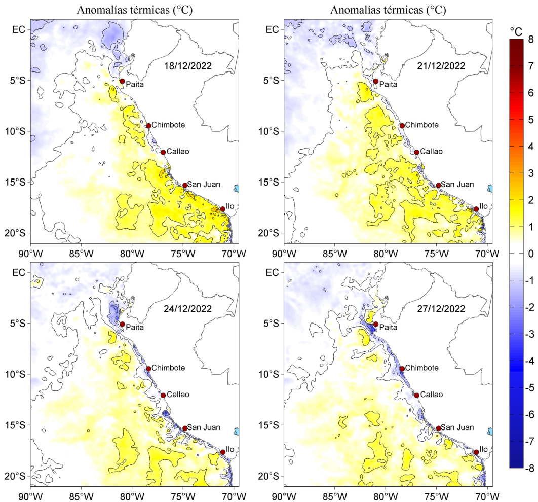
Figura 3. Anomalías de la temperatura superficial del mar (°C) para el 18, 21, 24 y 27 de diciembre de 2022. Las anomalías se calcularon respecto de la climatología para el periodo 2007-2016. Datos: OSTIA-UKMO-L4-GLOB-v2.0 (UK Met Office, 2012; Donlon et al, 2012).
