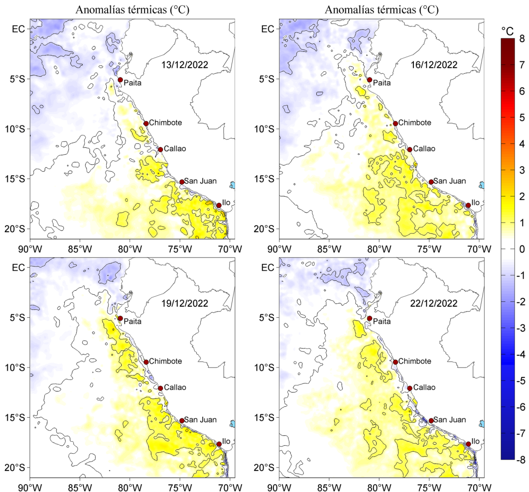
Figura 3. Anomalías de la temperatura superficial del mar (°C) para el 13, 16, 19 y 22 de diciembre de 2022. Las anomalías se calcularon respecto de la climatología para el periodo 2007-2016. Datos: OSTIA-UKMO-L4-GLOB-v2.0 (UK Met Office, 2012; Donlon et al, 2012).
