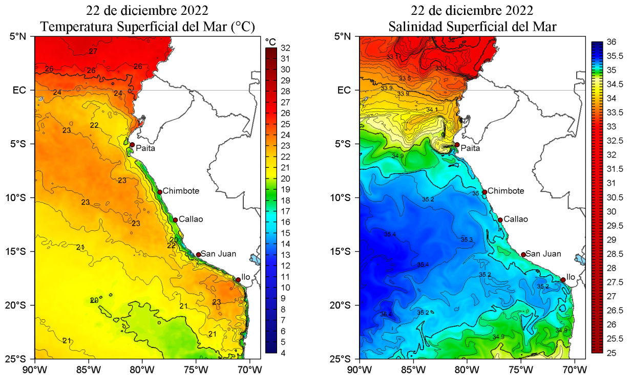
Figura 2. Temperatura superficial del mar (a la izquierda) y Salinidad superficial del mar (a la derecha) para el 22 de diciembre de 2022. Datos: OSTIA-UKMO-L4-GLOB-v2.0 (UK Met Office, 2012; Donlon et al, 2012) y Hybrid Coordinate Ocean Model v. GOFS 3.1 (HYCOM; Halliwell et al., 1998; 2000; Bleck, 2001), respectivamente.
