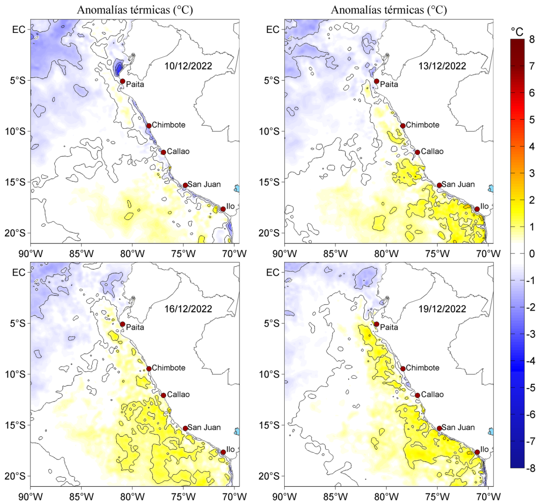
Figura 3. Anomalías de la temperatura superficial del mar (°C) para el 10, 13, 16 y 19 de diciembre de 2022. Las anomalías se calcularon respecto de la climatología para el periodo 2007-2016. Datos: OSTIA-UKMO-L4-GLOB-v2.0 (UK Met Office, 2012; Donlon et al, 2012).
