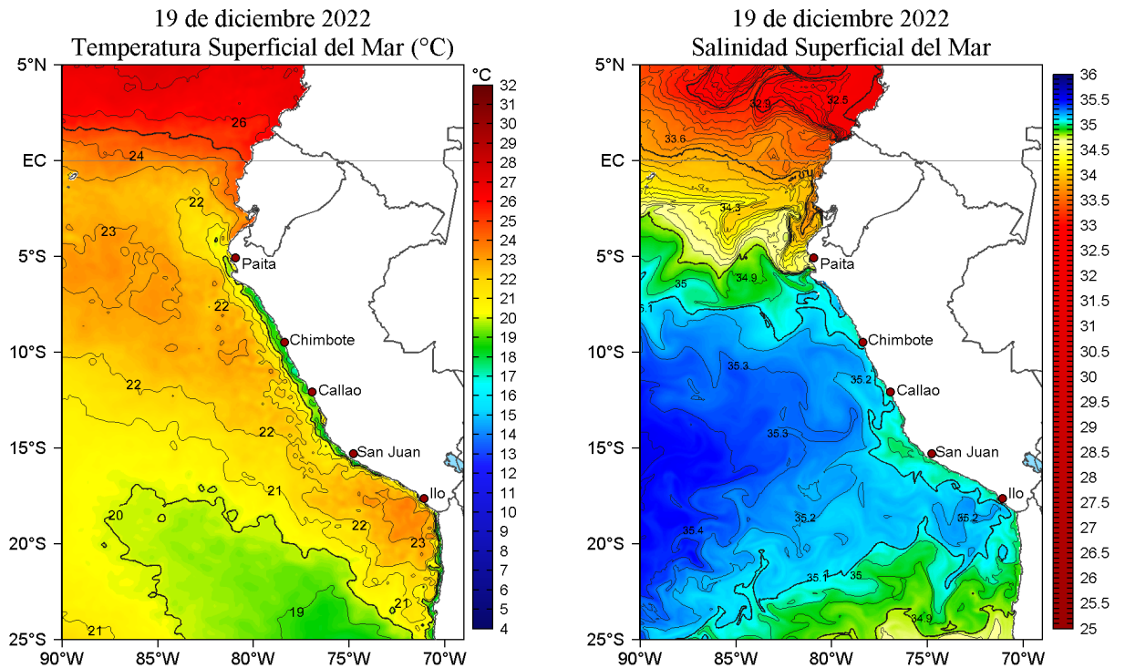
Figura 2. Temperatura superficial del mar (a la izquierda) y Salinidad superficial del mar (a la derecha) para el 19 de diciembre de 2022. Datos: OSTIA-UKMO-L4-GLOB-v2.0 (UK Met Office, 2012; Donlon et al, 2012) y Hybrid Coordinate Ocean Model v. GOFS 3.1 (HYCOM; Halliwell et al., 1998; 2000; Bleck, 2001), respectivamente.
