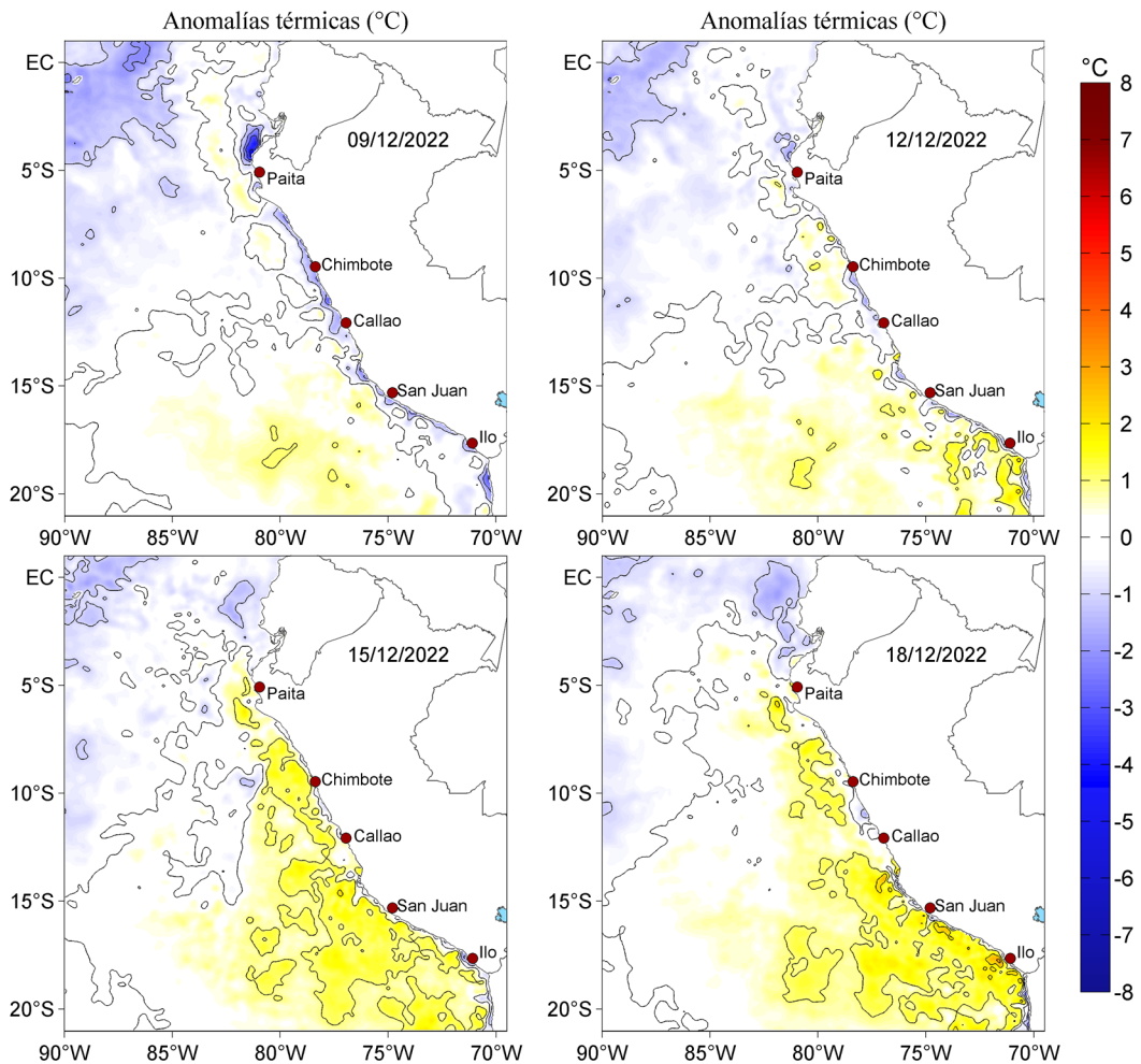
Figura 3. Anomalías de la temperatura superficial del mar (°C) para el 09, 12, 15 y 18 de diciembre de 2022. Las anomalías se calcularon respecto de la climatología para el periodo 2007-2016. Datos: OSTIA-UKMO-L4-GLOB-v2.0 (UK Met Office, 2012; Donlon et al, 2012).
