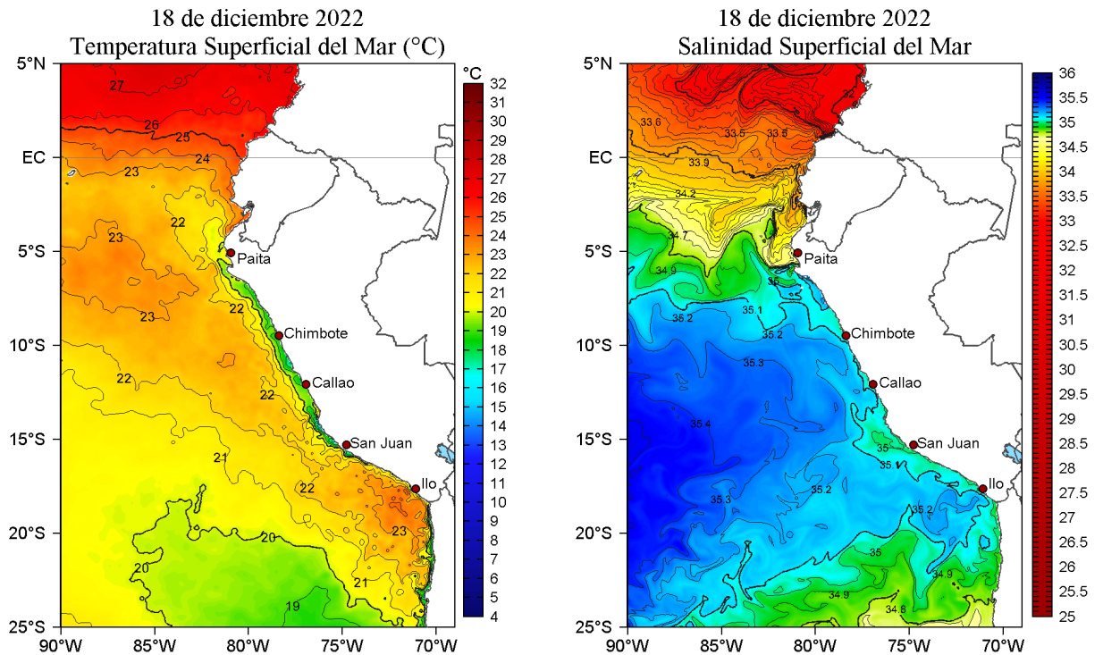
Figura 2. Temperatura superficial del mar (a la izquierda) y Salinidad superficial del mar (a la derecha) para el 18 de diciembre de 2022. Datos: OSTIA-UKMO-L4-GLOB-v2.0 (UK Met Office, 2012; Donlon et al, 2012) y Hybrid Coordinate Ocean Model v. GOFS 3.1 (HYCOM; Halliwell et al., 1998; 2000; Bleck, 2001), respectivamente.
