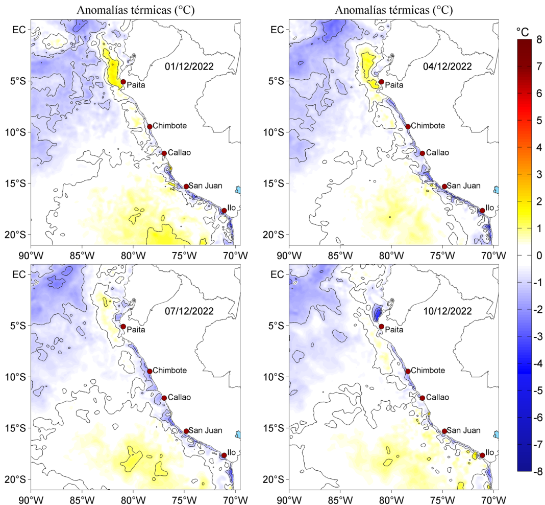
Figura 3. Anomalías de la temperatura superficial del mar (°C) para el 01, 04, 07 y 10 de diciembre de 2022. Las anomalías se calcularon respecto de la climatología para el periodo 2007-2016. Datos: OSTIA-UKMO-L4-GLOB-v2.0 (UK Met Office, 2012; Donlon et al, 2012).
