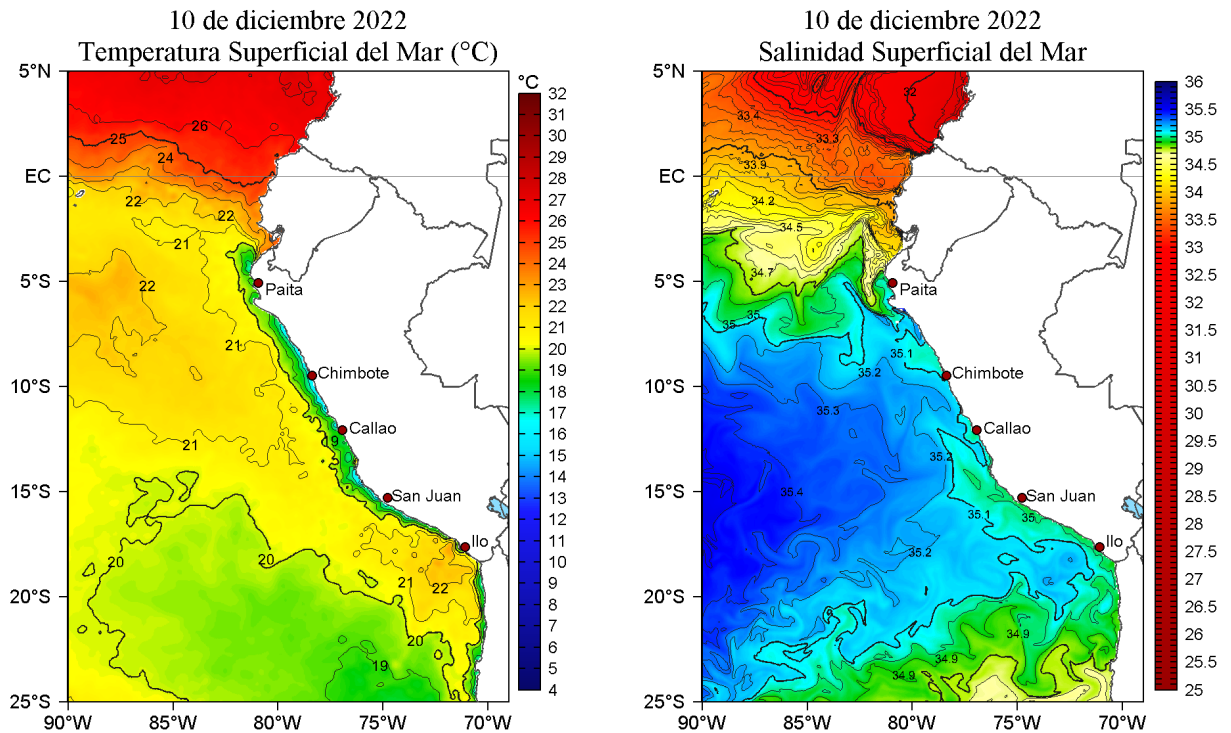
Figura 2. Temperatura superficial del mar (a la izquierda) y Salinidad superficial del mar (a la derecha) para el 10 de diciembre de 2022. Datos: OSTIA-UKMO-L4-GLOB-v2.0 (UK Met Office, 2012; Donlon et al, 2012) y Hybrid Coordinate Ocean Model v. GOFS 3.1 (HYCOM; Halliwell et al., 1998; 2000; Bleck, 2001), respectivamente.
