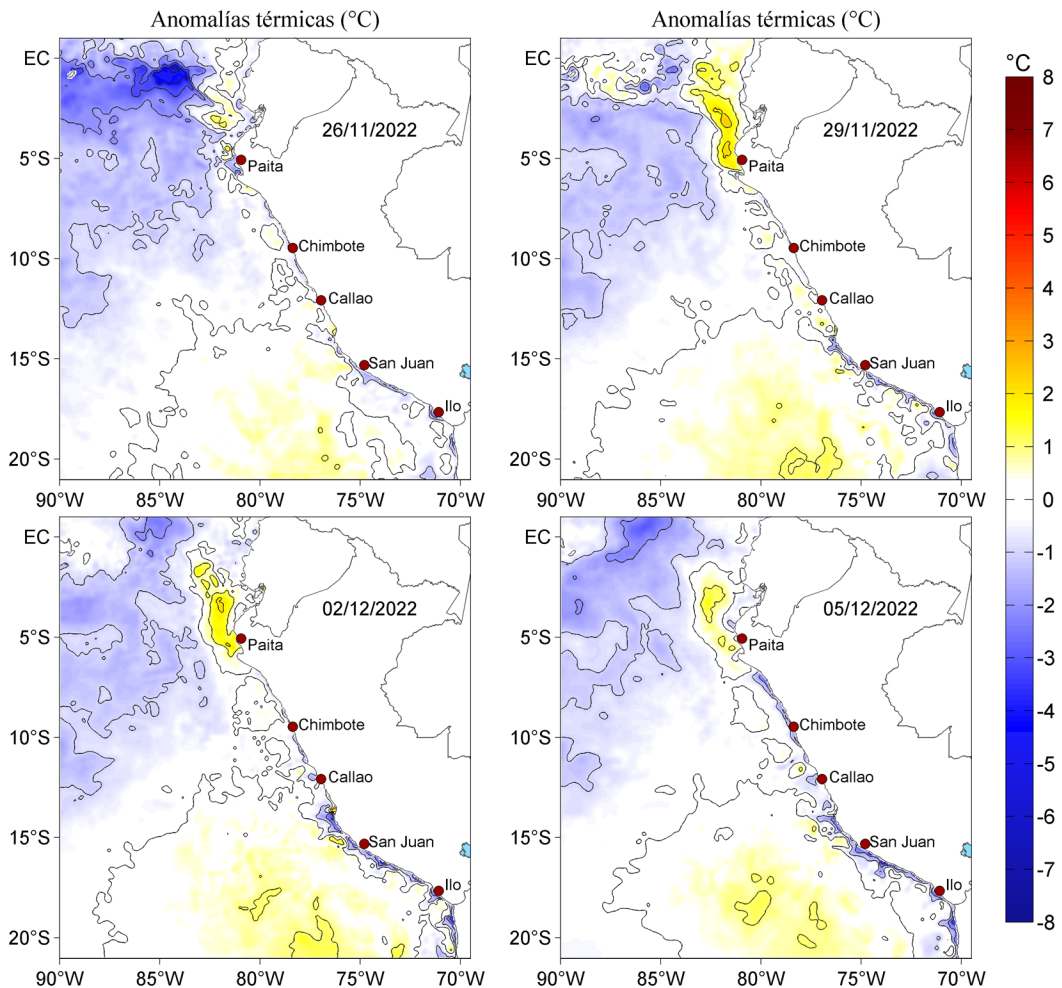
Figura 3. Anomalías de la temperatura superficial del mar (°C) para el 26 y 29 de noviembre, así como para el 02 y 05 de diciembre de 2022. Las anomalías se calcularon respecto de la climatología para el periodo 2007-2016. Datos: OSTIA-UKMO-L4-GLOB-v2.0 (UK Met Office, 2012; Donlon et al, 2012).
