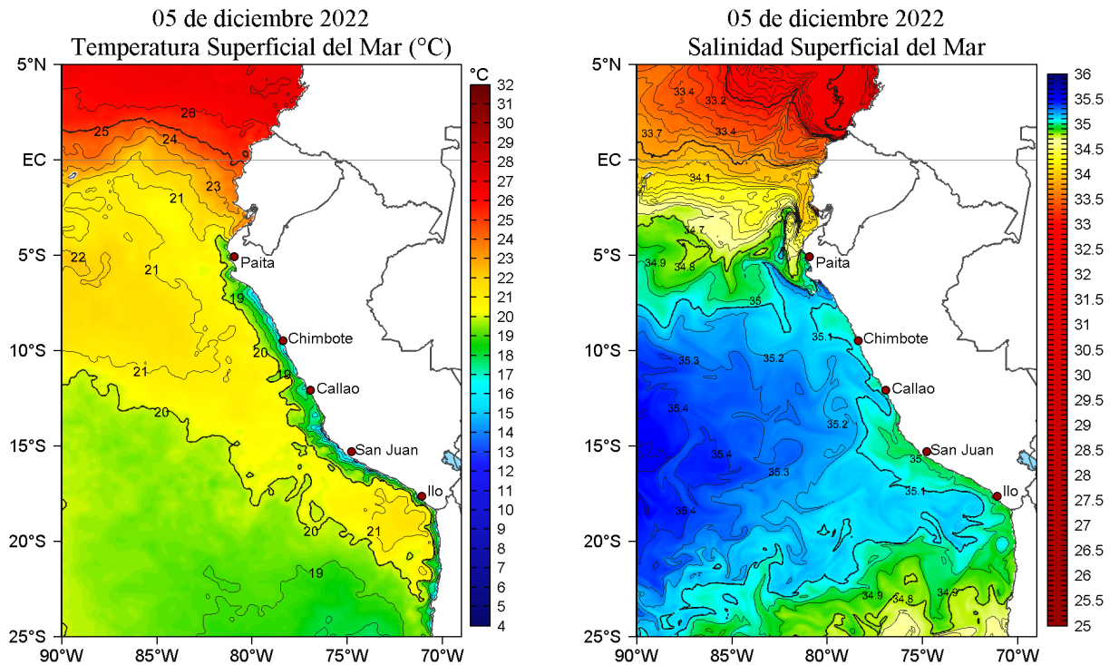
Figura 2. Temperatura superficial del mar (a la izquierda) y Salinidad superficial del mar (a la derecha) para el 05 de diciembre de 2022. Datos: OSTIA-UKMO-L4-GLOB-v2.0 (UK Met Office, 2012; Donlon et al, 2012) y Hybrid Coordinate Ocean Model v. GOFS 3.1 (HYCOM; Halliwell et al., 1998; 2000; Bleck, 2001), respectivamente.
