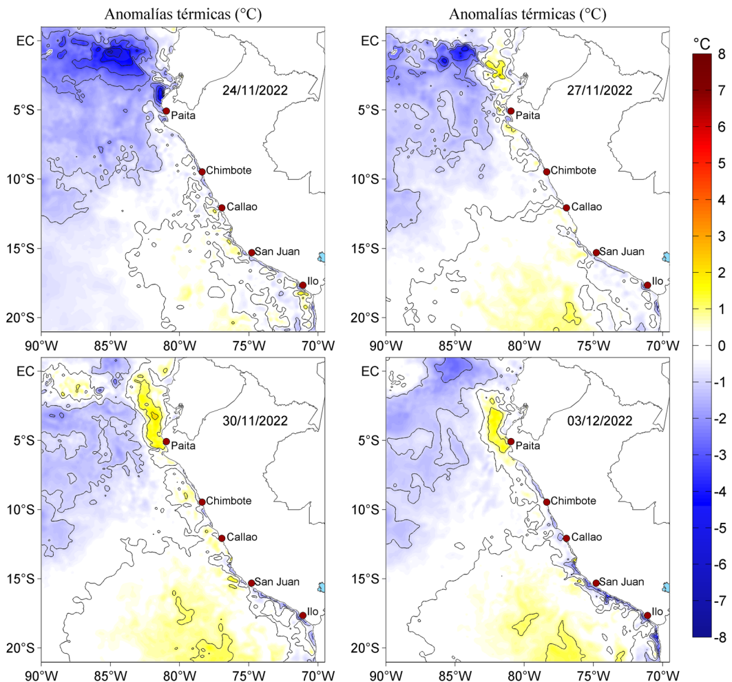
Figura 3. Anomalías de la temperatura superficial del mar (°C) para el 24, 27 y 30 de noviembre, así como para el 03 de diciembre de 2022. Las anomalías se calcularon respecto de la climatología para el periodo 2007-2016. Datos: OSTIA-UKMO-L4-GLOB-v2.0 (UK Met Office, 2012; Donlon et al, 2012).
