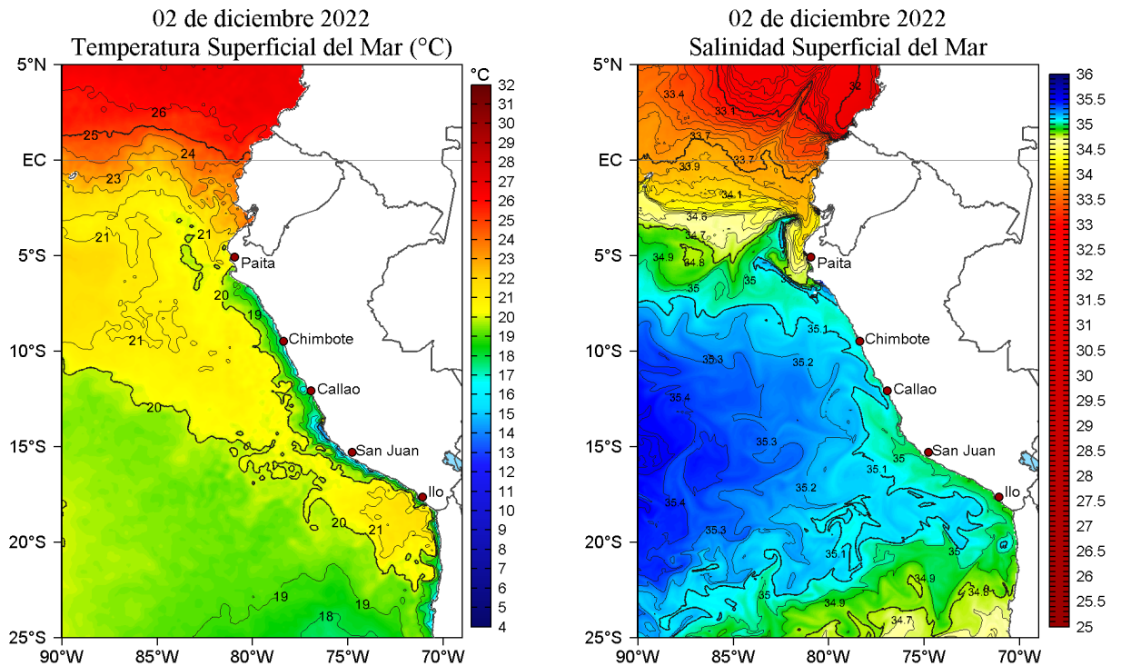
Figura 2. Temperatura superficial del mar (a la izquierda) y Salinidad superficial del mar (a la derecha) para el 02 de diciembre de 2022. Datos: OSTIA-UKMO-L4-GLOB-v2.0 (UK Met Office, 2012; Donlon et al, 2012) y Hybrid Coordinate Ocean Model v. GOFS 3.1 (HYCOM; Halliwell et al., 1998; 2000; Bleck, 2001), respectivamente.
