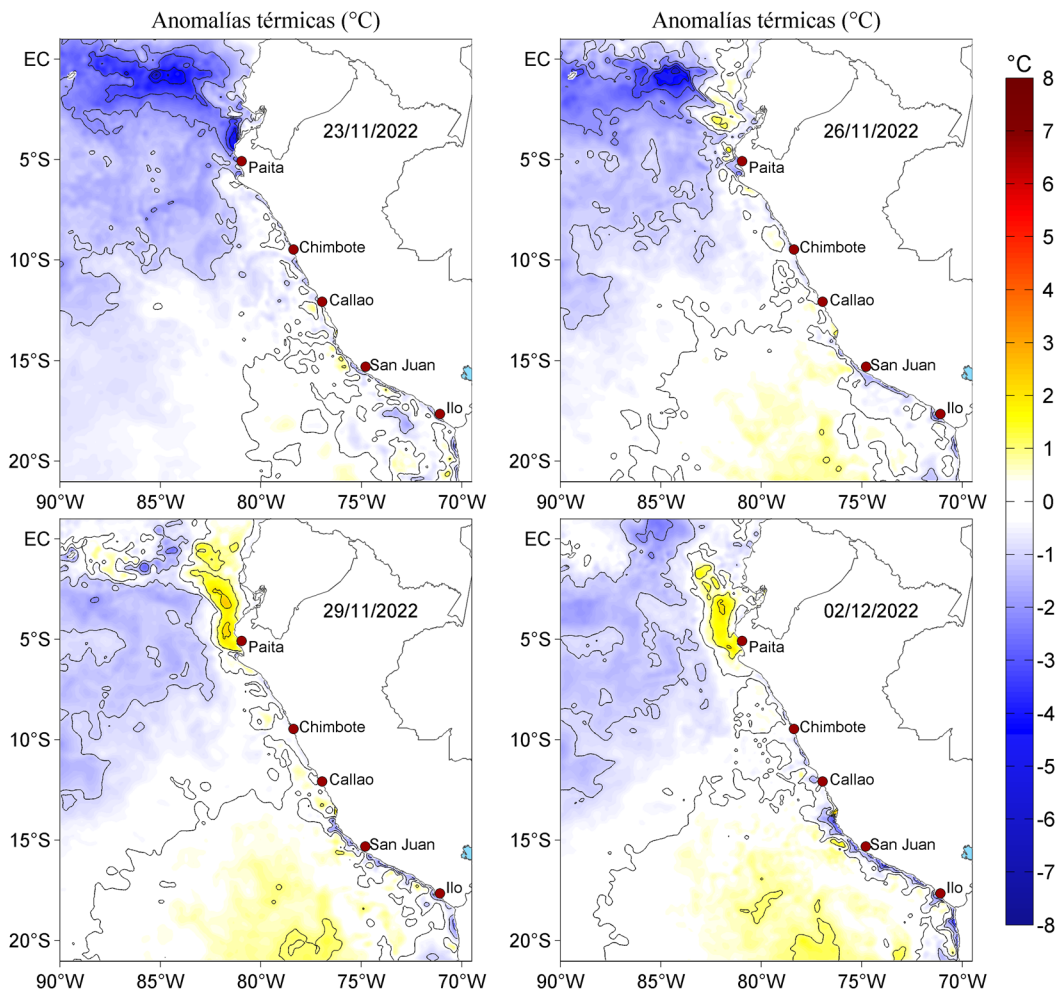
Figura 3. Anomalías de la temperatura superficial del mar (°C) para el 23, 26 y 29 de noviembre, así como para el 02 de diciembre de 2022. Las anomalías se calcularon respecto de la climatología para el periodo 2007-2016. Datos: OSTIA-UKMO-L4-GLOB-v2.0 (UK Met Office, 2012; Donlon et al, 2012).
