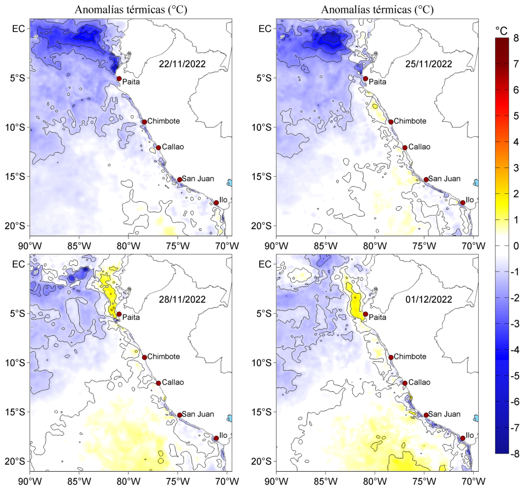
Figura 3. Anomalías de la temperatura superficial del mar (°C) para el 22, 25 y 28 de noviembre, así como para el 01 de diciembre de 2022. Las anomalías se calcularon respecto de la climatología para el periodo 2007-2016. Datos: OSTIA-UKMO-L4-GLOB-v2.0 (UK Met Office, 2012; Donlon et al, 2012).
