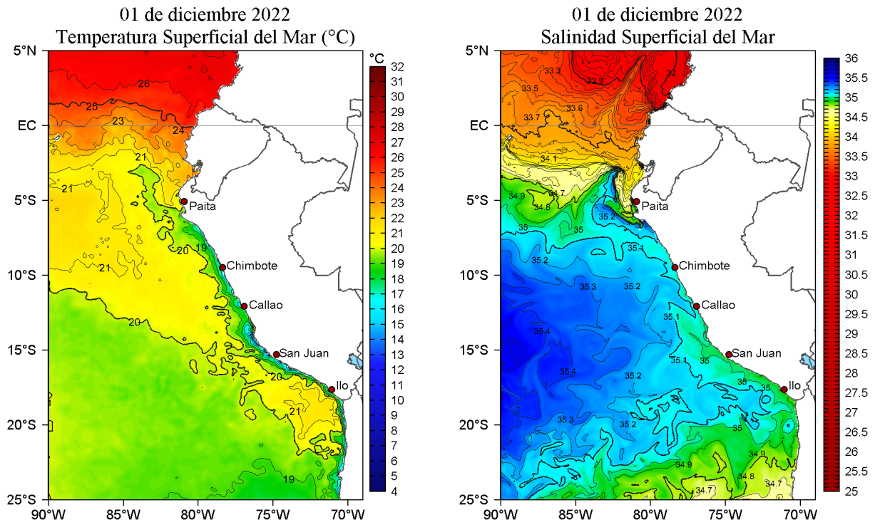
Figura 2. Temperatura superficial del mar (a la izquierda) y Salinidad superficial del mar (a la derecha) para el 01 de diciembre de 2022. Datos: OSTIA-UKMO-L4-GLOB-v2.0 (UK Met Office, 2012; Donlon et al, 2012) y Hybrid Coordinate Ocean Model v. GOFS 3.1 (HYCOM; Halliwell et al., 1998; 2000; Bleck, 2001), respectivamente.
