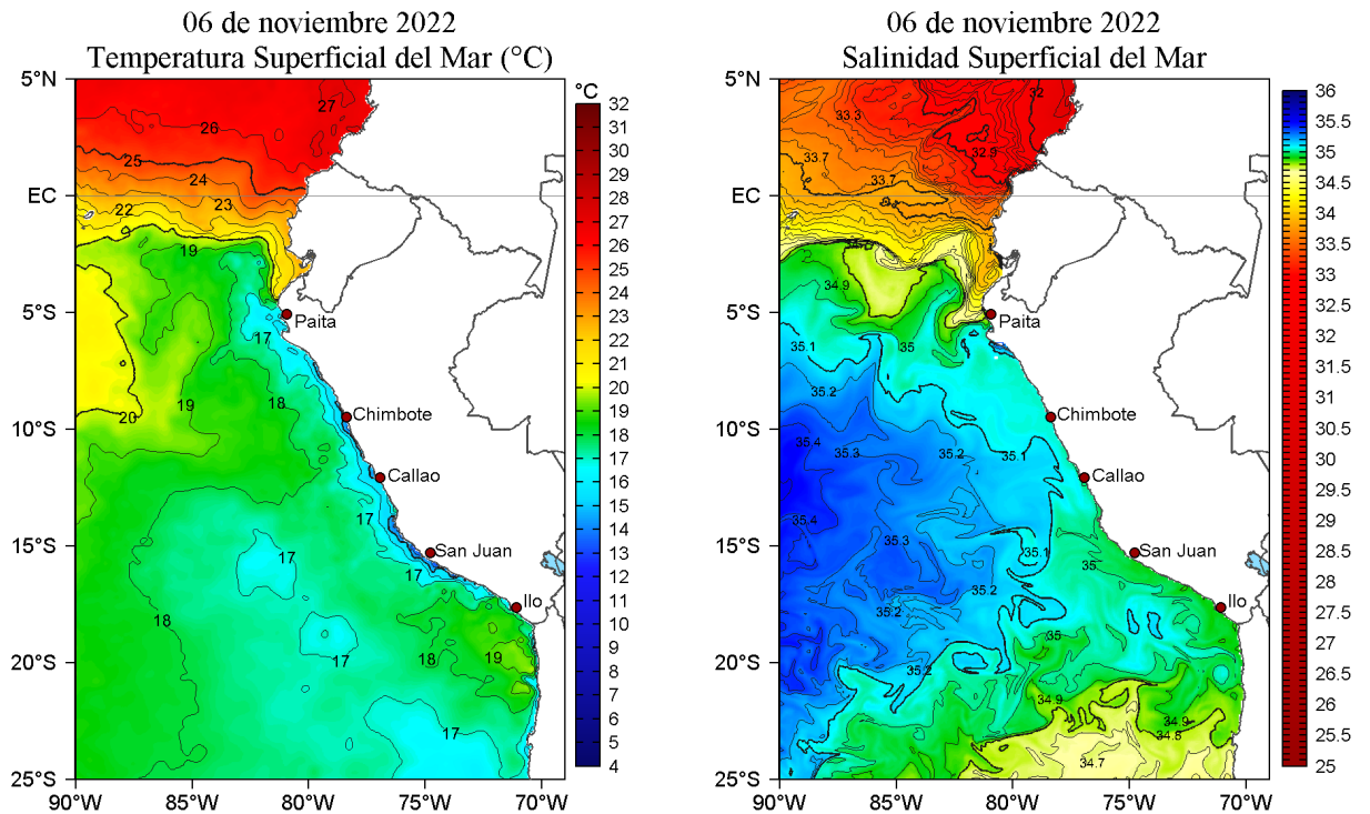
Figura 2. Temperatura superficial del mar (a la izquierda) y Salinidad superficial del mar (a la derecha) para el 06 de noviembre de 2022. Datos: OSTIA-UKMO-L4-GLOB-v2.0 (UK Met Office, 2012; Donlon et al, 2012) y Hybrid Coordinate Ocean Model v. GOFS 3.1 (HYCOM; Halliwell et al., 1998; 2000; Bleck, 2001), respectivamente.
