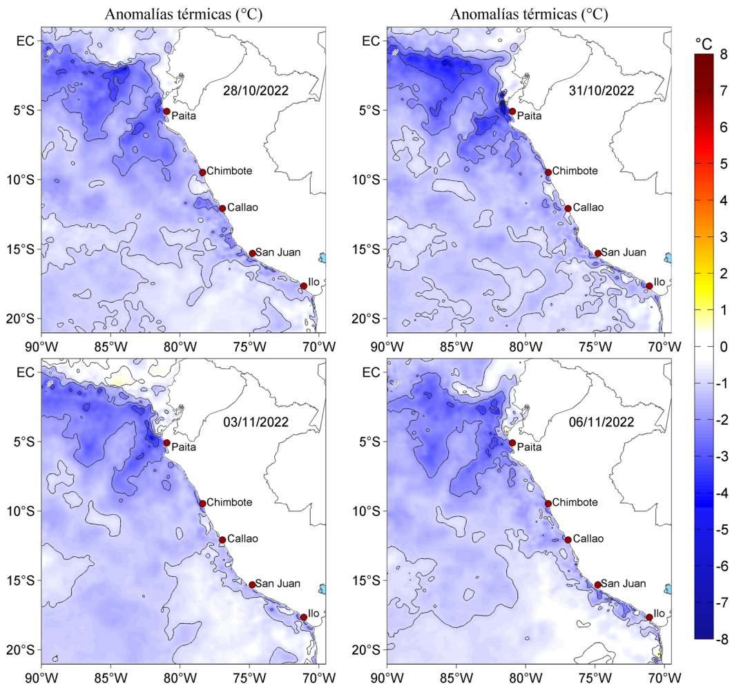
Figura 3. Anomalías de la temperatura superficial del mar (°C) para el 28 y 31 de octubre, así como para el 03 y 06 de noviembre de 2022. Las anomalías se calcularon respecto de la climatología para el periodo 2007-2016. Datos: OSTIA-UKMO-L4-GLOB-v2.0 (UK Met Office, 2012; Donlon et al, 2012).
