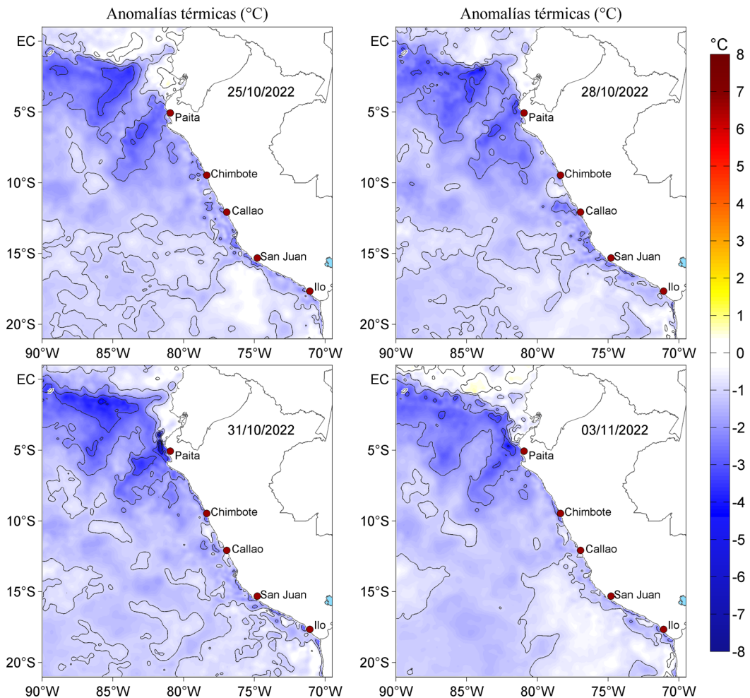
Figura 3. Anomalías de la temperatura superficial del mar (°C) para el 25, 28 y 31 de octubre, así como para el 03 de noviembre de 2022. Las anomalías se calcularon respecto de la climatología para el periodo 2007-2016. Datos: OSTIA-UKMO-L4-GLOB-v2.0 (UK Met Office, 2012; Donlon et al, 2012).
