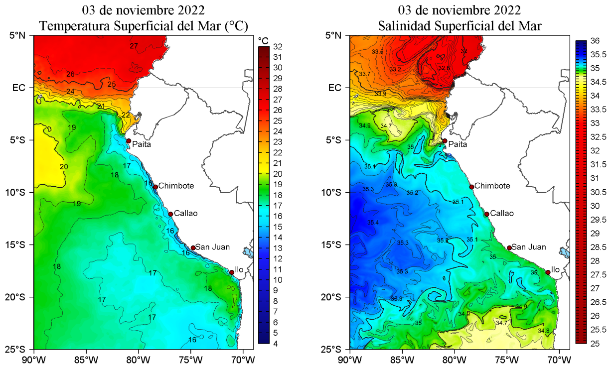
Figura 2. Temperatura superficial del mar (a la izquierda) y Salinidad superficial del mar (a la derecha) para el 03 de noviembre de 2022. Datos: OSTIA-UKMO-L4-GLOB-v2.0 (UK Met Office, 2012; Donlon et al, 2012) y Hybrid Coordinate Ocean Model v. GOFS 3.1 (HYCOM; Halliwell et al., 1998; 2000; Bleck, 2001), respectivamente.
