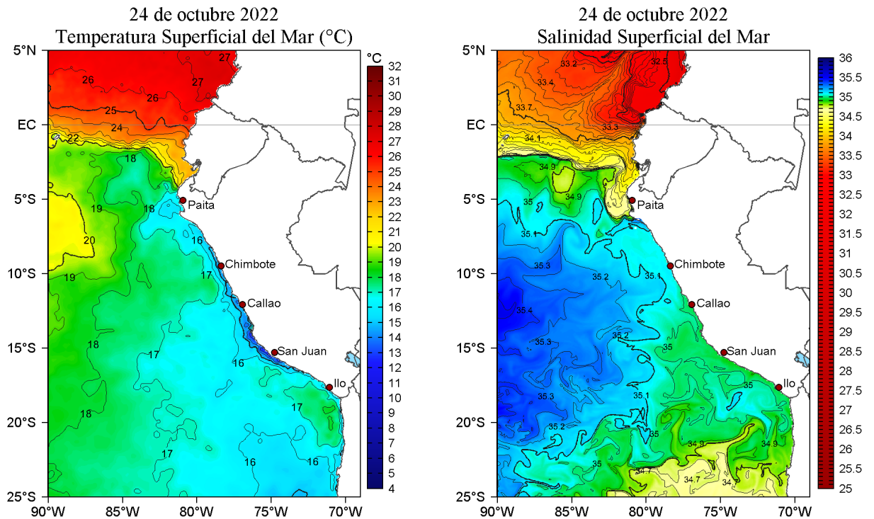
Figura 2. Temperatura superficial del mar (a la izquierda) y Salinidad superficial del mar (a la derecha) para el 24 de octubre de 2022. Datos: OSTIA-UKMO-L4-GLOB-v2.0 (UK Met Office, 2012; Donlon et al, 2012) y Hybrid Coordinate Ocean Model v. GOFS 3.1 (HYCOM; Halliwell et al., 1998; 2000; Bleck, 2001), respectivamente.
