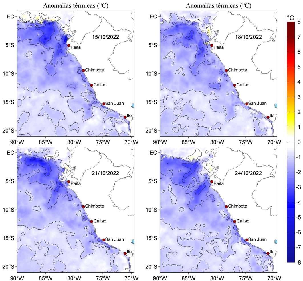
Figura 3. Anomalías de la temperatura superficial del mar (°C) para el 15, 18, 21 y 24 de octubre de 2022. Las anomalías se calcularon respecto de la climatología para el periodo 2007-2016. Datos: OSTIA-UKMO-L4-GLOB-v2.0 (UK Met Office, 2012; Donlon et al, 2012).
